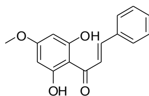
Illustration 54 : DMC
