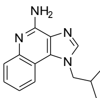
Illustration 13 : Imiquimod®
