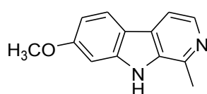
Illustration 47 : Harmine
