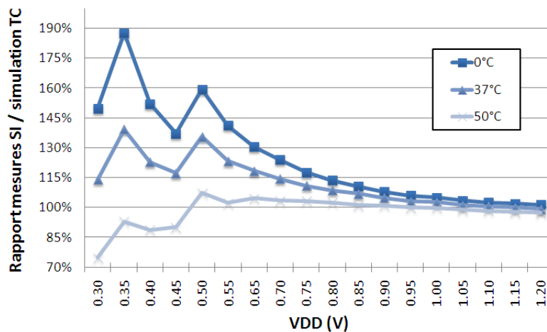
Figure 3.11 – Alignement des oscillateurs avec le modèle en fonction de la température.
