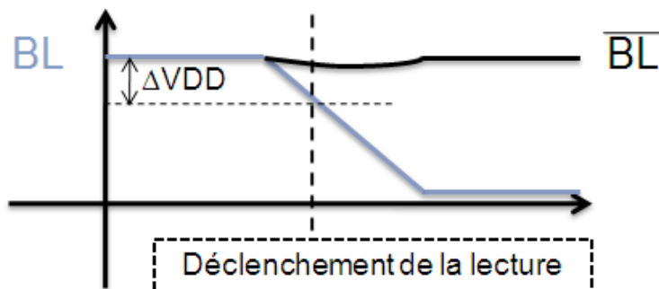
Figure 4.23 – Principe de lecture par l’utilisation d’un amplificateur différentiel.
