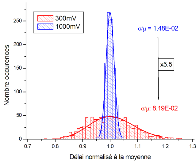
Figure 2.14 - Distribution du délai à tension nominale et à très faible tension, pour 1000 tirages Monte-Carlo.
