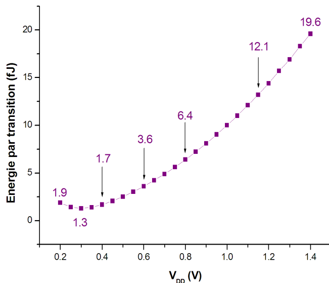
Figure 2.11 – Énergie par transition de la chaîne qF04 en fonction de la tension d'alimentation.
