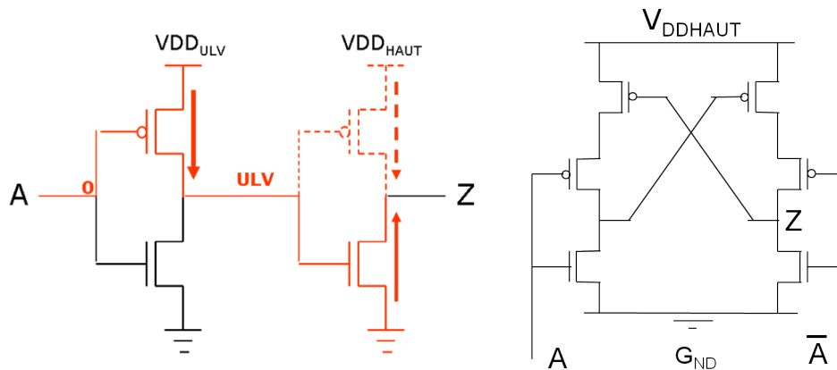
Figure 1.9 – Principe du Level Shifter et mise en évidence du court-circuit (gauche), et Level Shifter standard avec A l'entrée alimentée à la tension basse (droite).
