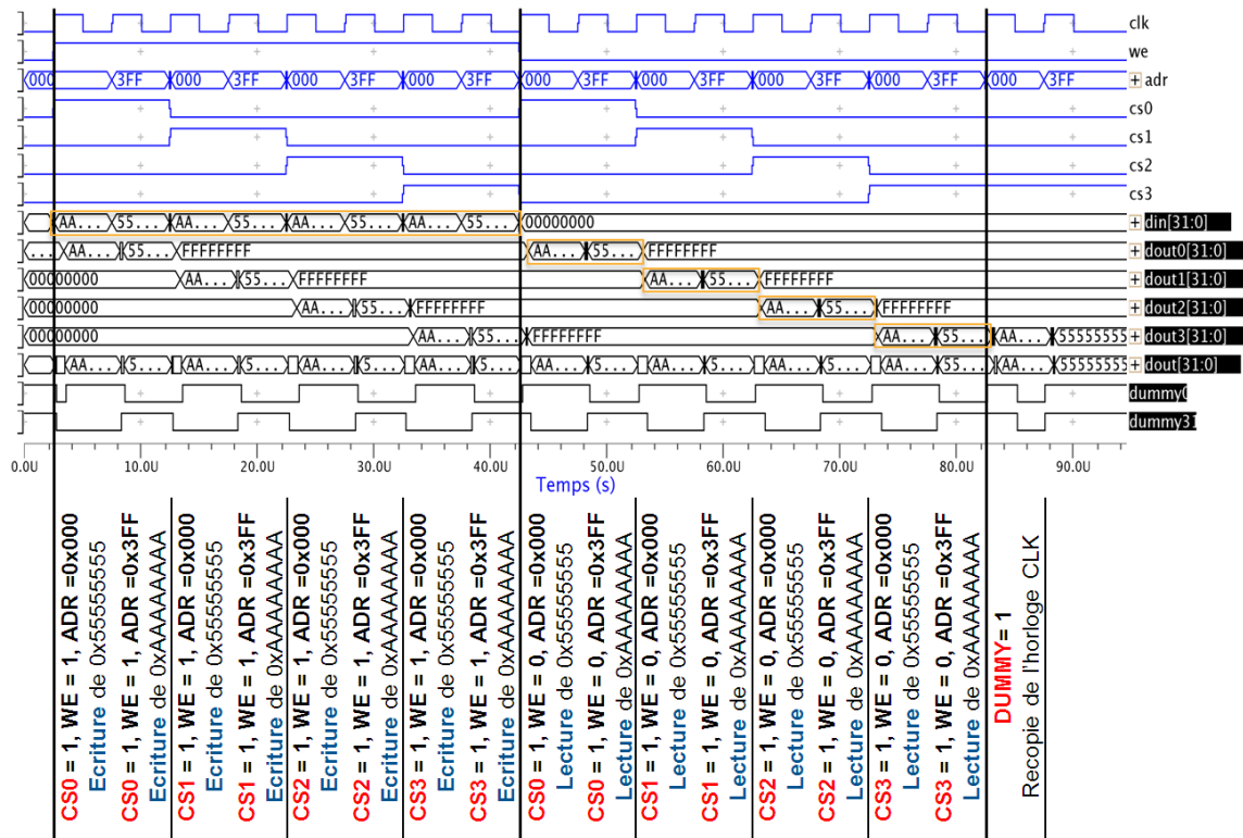
Figure 4.34 - Chronogrammes de la simulation à 0,35V, 25°C, du démonstrateur.
