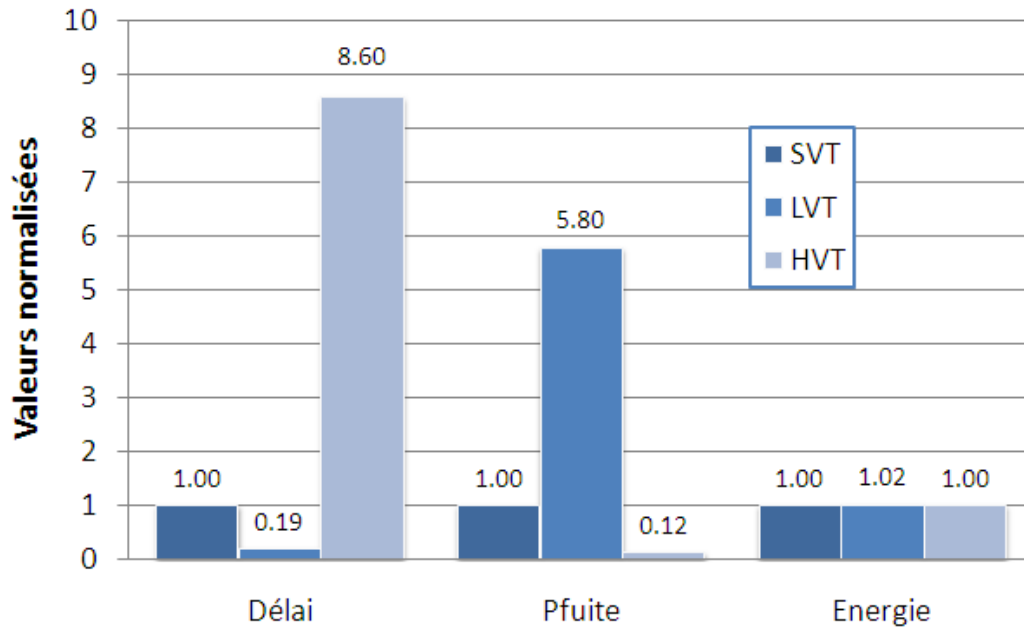
Figure 2.17 – Résultats de la simulation du qFO4 à 350mV pour plusieurs VT.
