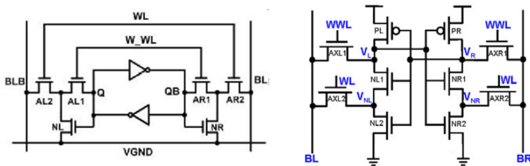
Figure 4.10 – Représentation schématique de la mémoire SRAM10T_KR (gauche) et de la mémoire SRAM10T_ST (droite).
