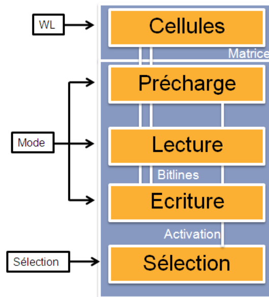
Figure 4.22 – Contenu du bloc de sélection et opération.
