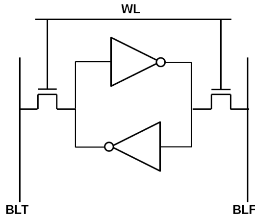
Figure 1.8 – Cellule SRAM à 6 transistors.
