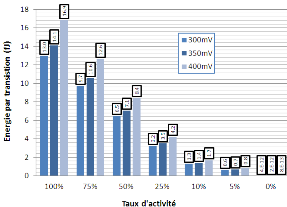
Figure 2.12 – Évolution de l'énergie par transition en fonction du taux d'activité, pour trois tensions différentes.
