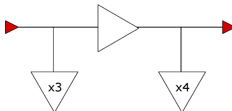
Figure 2.8 – Chemin logique rFO4 utilisant des charges fixées par la cellule de référence.
