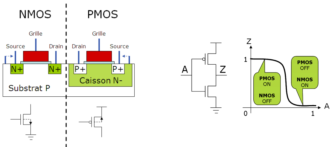
Figure 1.1 – Transistors MOS et exemple d'un inverseur CMOS.
