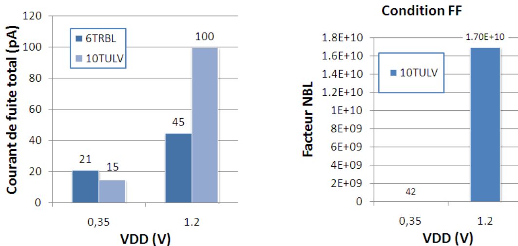
Figure 4.20 – Courant statique total des cellules 6T_RBL et 10T_ULV (gauche), et facteur N_{BL} pour la cellule 10T_ULV pour une hauteur de 128 lignes.
