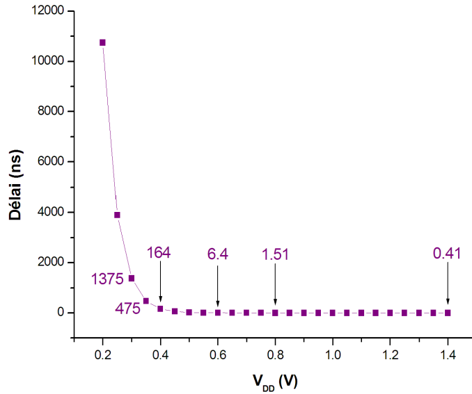
Figure 2.9 – Délai de la chaîne qF04 en fonction de la tension d’alimentation.
