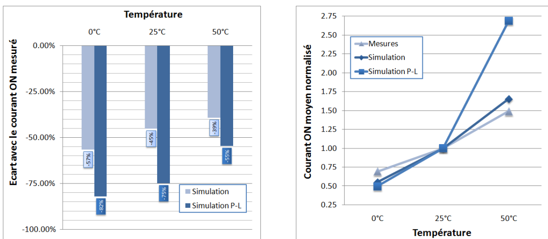
Figure 2.4 – Centrage et variation du courant dynamique en fonction de la température, mesurés à 350mV.
