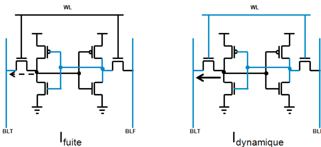
Figure 4.7 – Représentation schématique de la simulation permettant d'extraire le courant de fuite (gauche), et le courant dynamique (droite).
