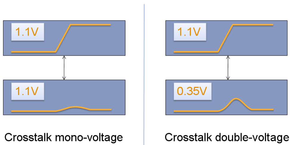
Figure 3.15 – Représentation du phénomène de Crosstalk.
