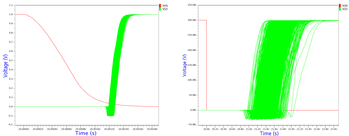
Figure 2.13 – Simulation Monte-carlo du délai sur le chemin logique qFO4 à 1.1V et 0.3V, à 25°
