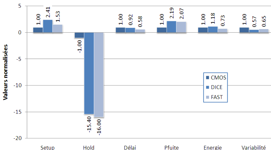
Figure 2.31 – Résultats de la simulation à 350mV pour les différents Flip-Flops.
