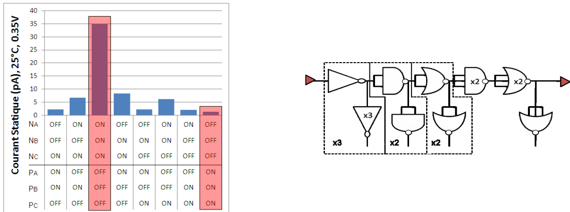
Figure 2.7 – Extraction des extremums en courant statique en fonction de la configuration des entrées (gauche) et chemin logique qFO4 (droite).
