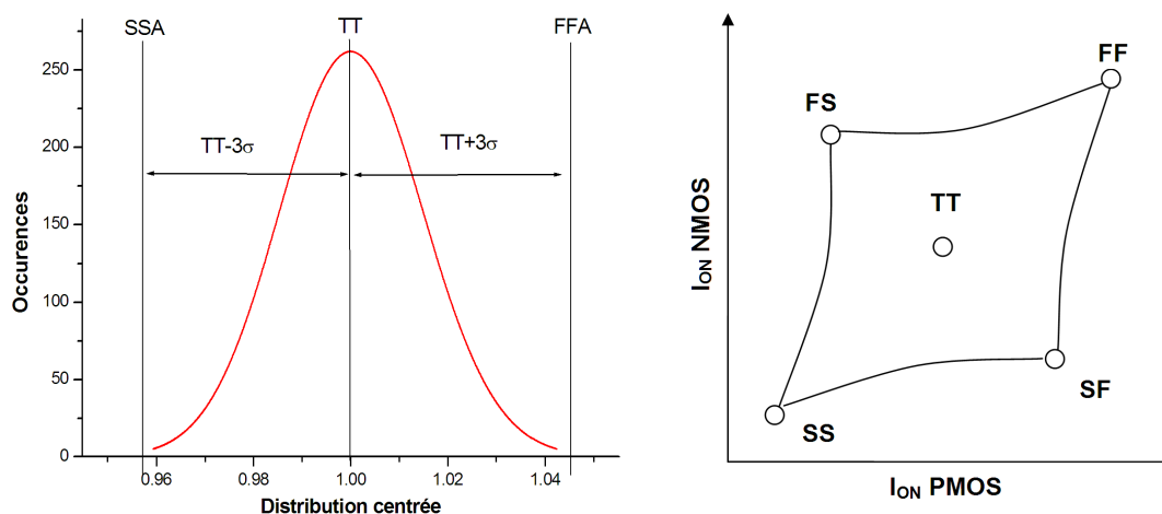
Figure 2.2 – Distribution des variations autour de la moyenne et espace des conditions du transistor.
