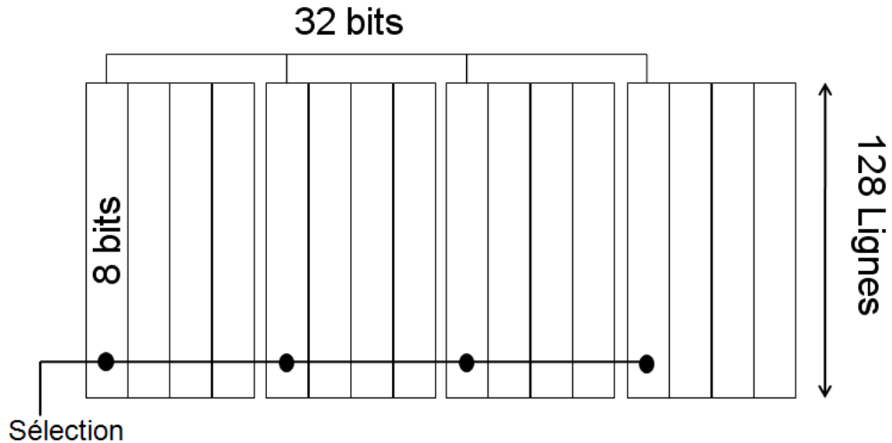
Figure 4.32 – Représentation schématique d'une mémoire.
