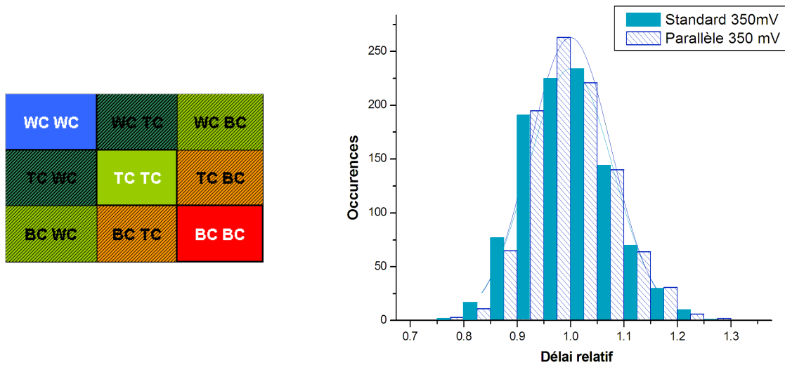
Figure 2.26 – Conditions du couple de transistor et simulation Monte-Carlo de la stratégie de mise en parallèle systématique à 350mV.
