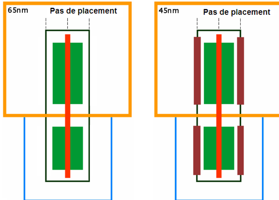
Figure 2.1 – Représentation de la répétition des motifs de grille en technologie 40nm. Ces motifs sont flottants.
