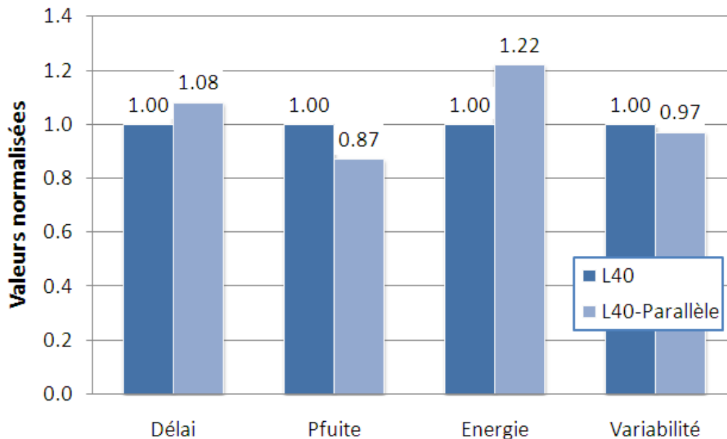
Figure 2.27 – Résultats de la simulation du qFO4 à 350mV pour les stratégies standards et mise en parallèle systématique.
