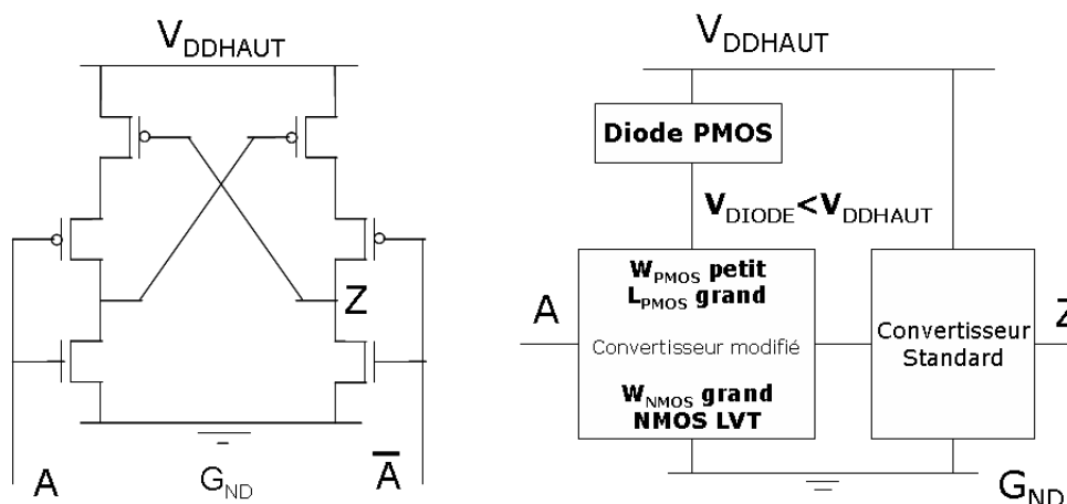
Figure 2.33 – Convertisseur de tension standard (gauche) et convertisseur de tension très faible tension (droite)
