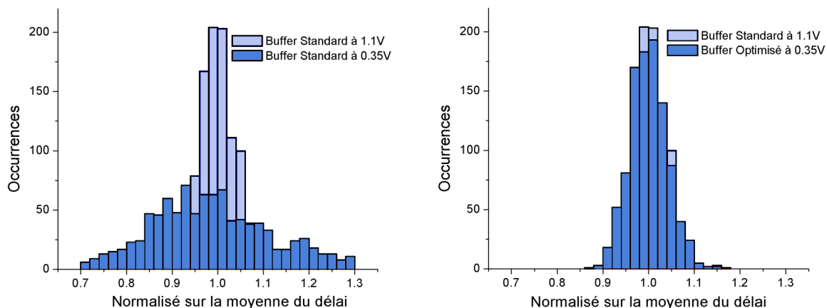
Figure 2.35 – Superposition des différentes distributions : Buffer standard avec V_{DD}=1.1V , Buffer standard avec V_{DD}=0.35V , et Buffer optimisé avec V_{DD} = 0.35V .
