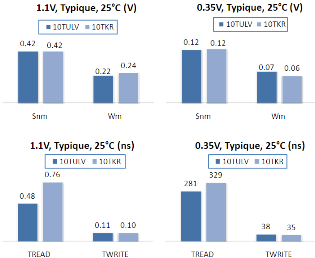
Figure 4.15 - Comparaison des résultats entre les structures SRAM10T_KR et SRAM10T_ULV.
