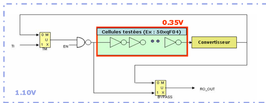
Figure 2.37 – Schéma de l’oscillateur conçu pour la validation sur silicium.
