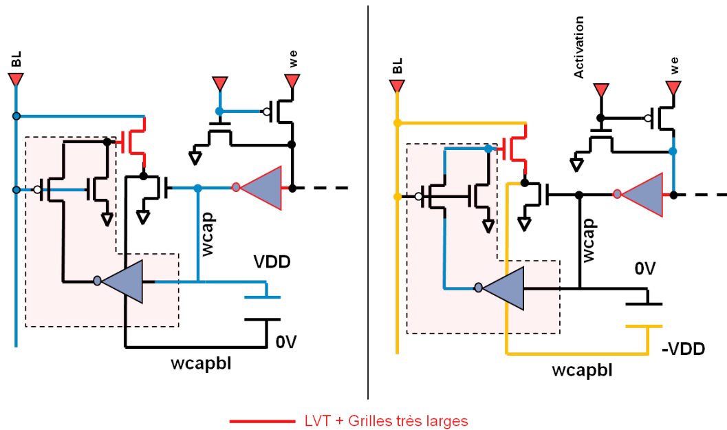
Figure 4.29 – Phases de précharge (gauche) et de charge (droite) de la solution d’assistance à l’écriture.
