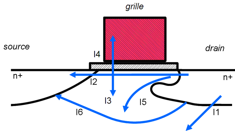
Figure 1.2 – Les courants de fuite du transistor MOS.
