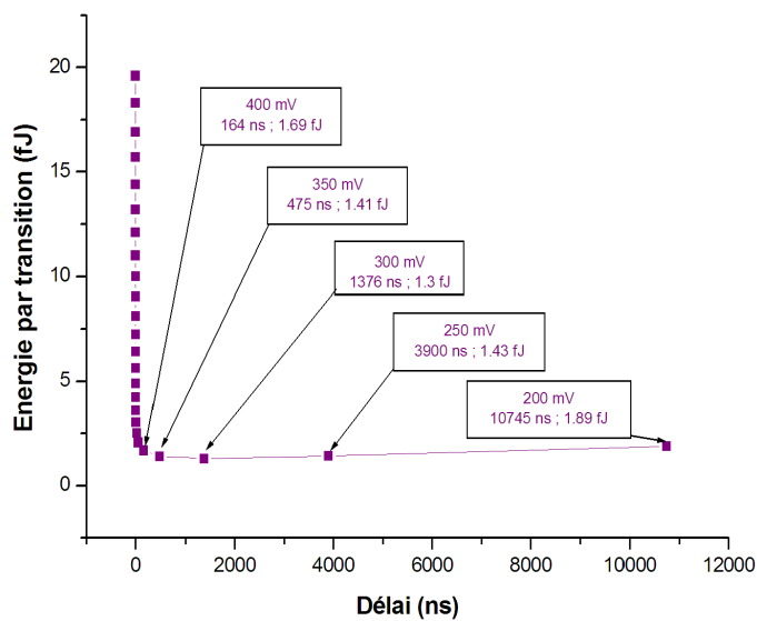
Figure 2.16 – Expression de l'énergie en fonction du délai pour la recherche du V_{OPT} .
