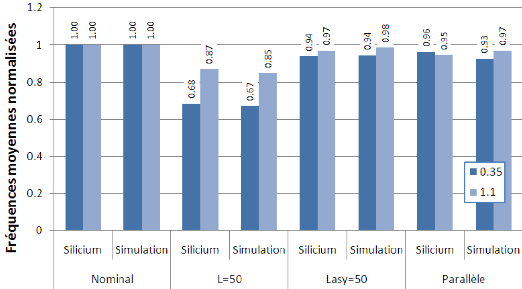
Figure 2.39 – Mesures sur silicium de la fréquence des différents oscillateurs, à 25°C.
