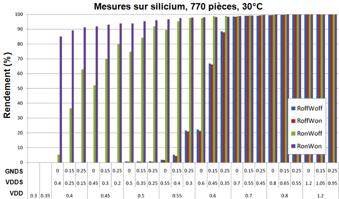
Figure 4.35 – Mesures sur silicium du rendement du démonstrateur à 30°C, en fonction de la tension d’alimentation, du Forward Body-Biasing appliqué, et de l’état d’activation des assistances.
