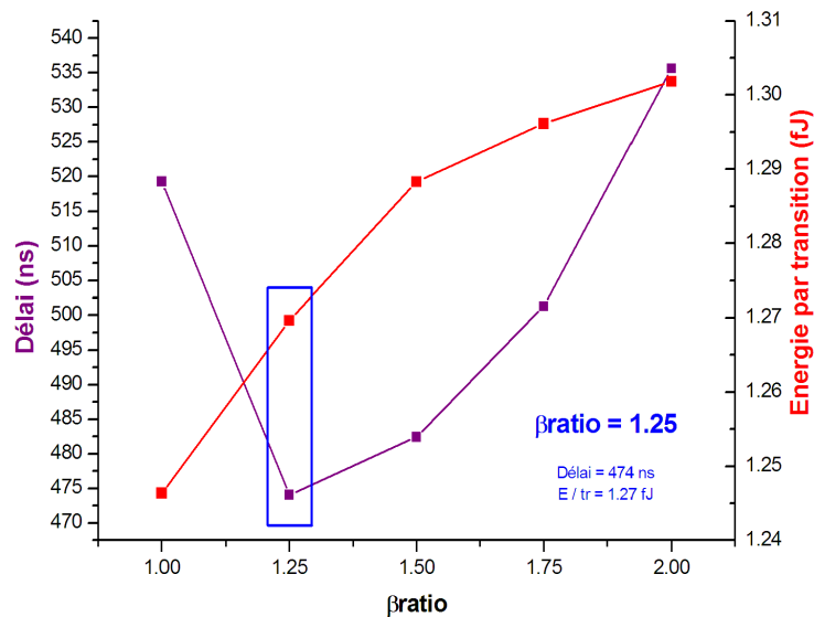
Figure 2.20 – Simulation de l’impact du \beta -ratio sur la fréquence et l’énergie, sur qFO4 à 350mV.
