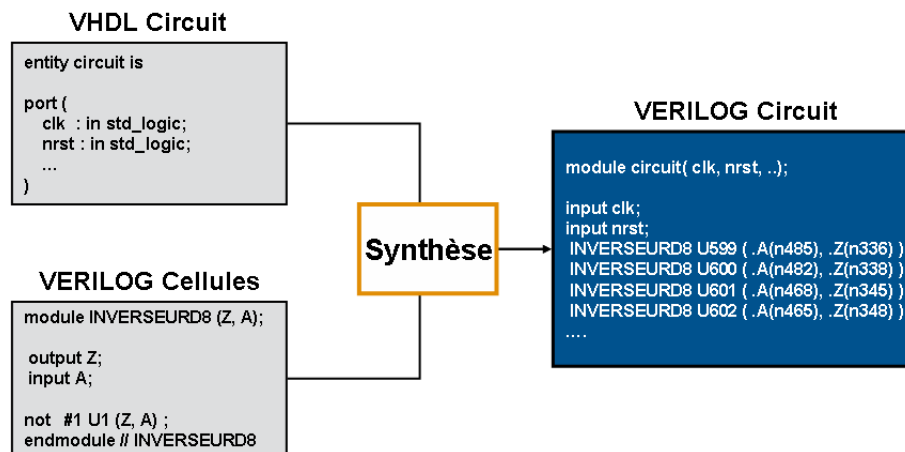
Figure 3.2 – Représentation de l'étape de synthèse d'un circuit.
