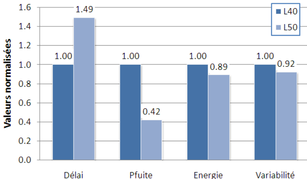
Figure 2.23 – Résultats de la simulation du qFO4 à 350mV pour les stratégies nominales et grilles longues systématiques.
