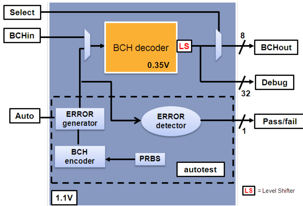
Figure 3.5 – Description schématique du décodeur d'erreur BCH. La sortie "pass" permet par un bit unique de vérifier la fonctionnalité du circuit.
