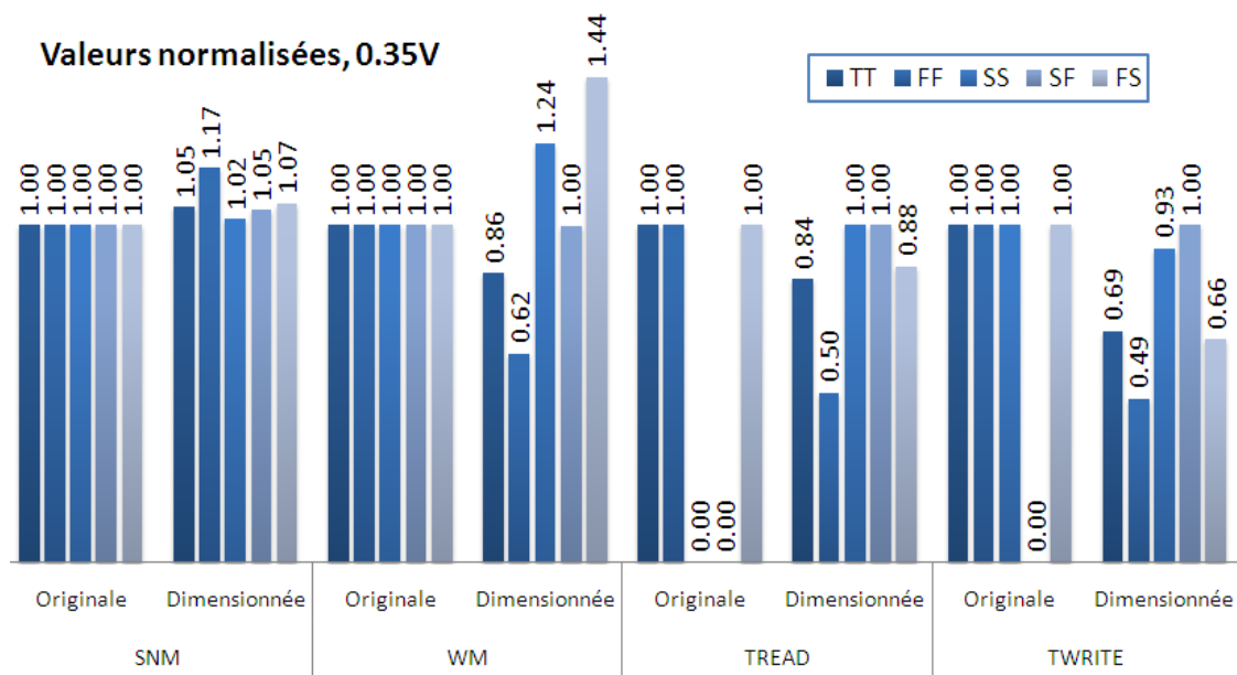
Figure 4.16 – Résultats obtenus sur l'ensemble des points de mesures.
