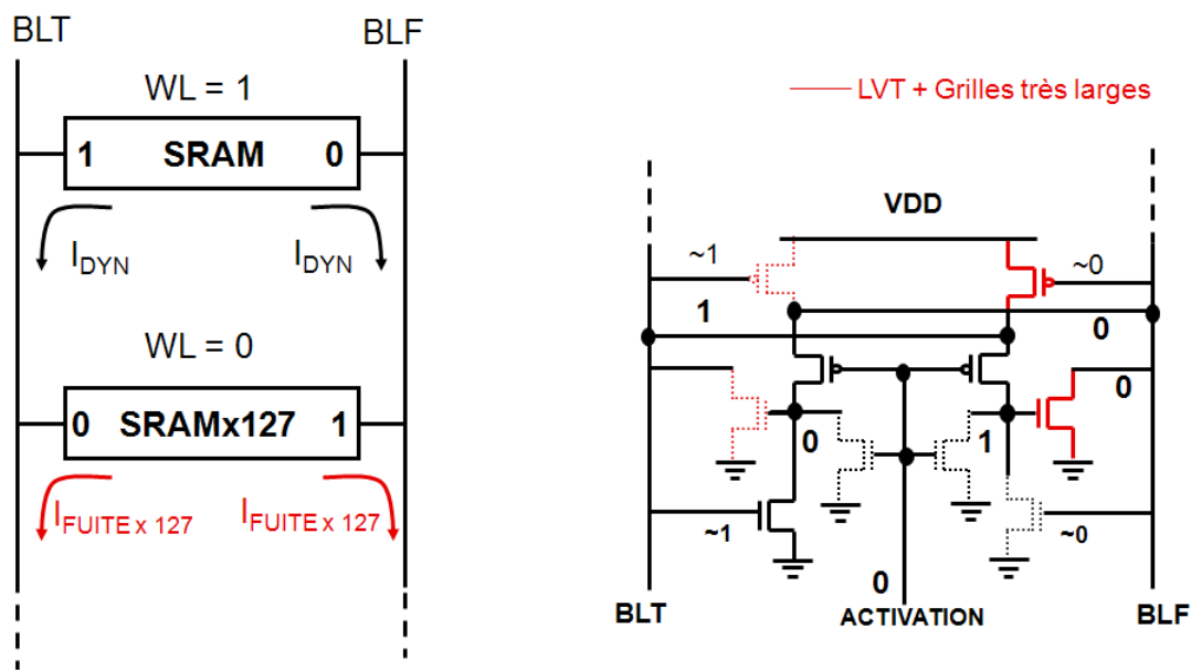
Figure 4.25 – Exemple de fonctionnement de l'assistance à la lecture.
