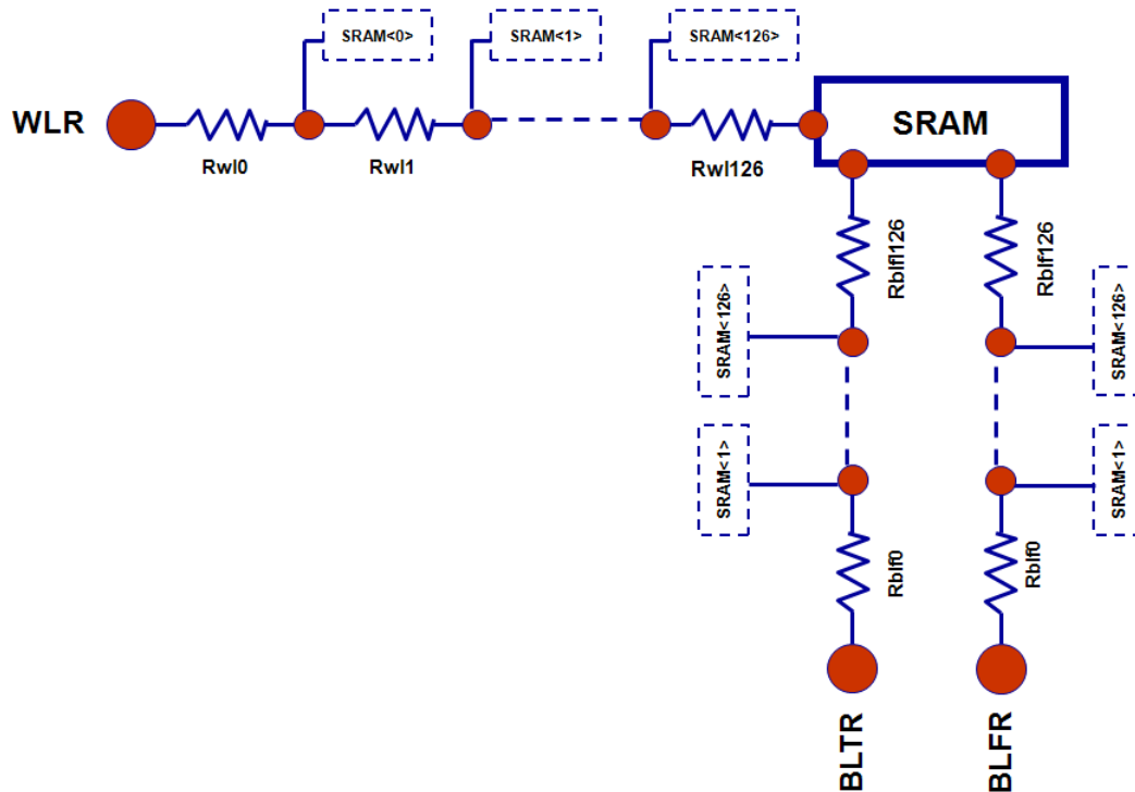
Figure 4.9 – Représentation schématique du chemin critique universel.
