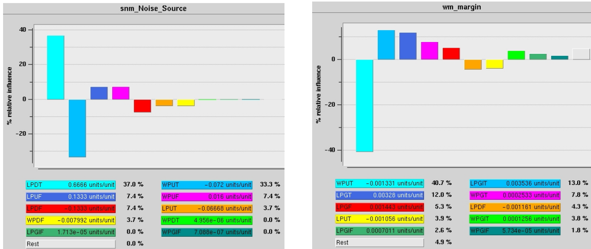
Figure 4.17 – Sensibilité de la SNM (gauche) et de la WM (droite) au dimensionnement des transistors de la cellule.
