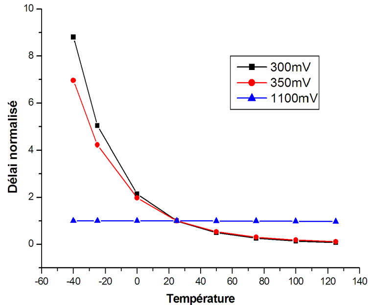
Figure 2.3 – Simulation du délai en fonction de la température.
