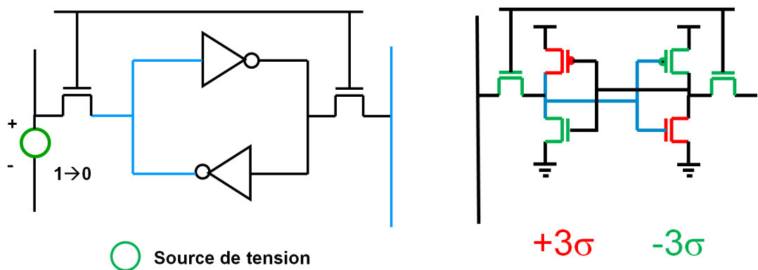
Figure 4.6 – Représentation schématique de la simulation permettant d'extraire la WM (gauche), et application de la méthodologie paramétrique (droite).
