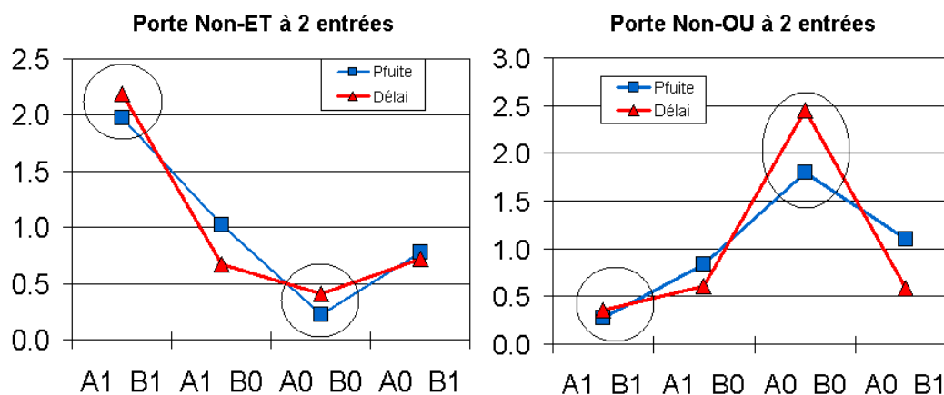
Figure 2.24 – Résultats de la simulation des portes Non-ET et Non-OU à 350mV en fonction des entrées.
