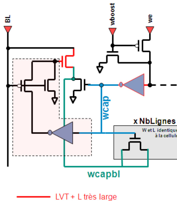
Figure 4.28 – Représentation schématique de la solution d'assistance à l'écriture.
