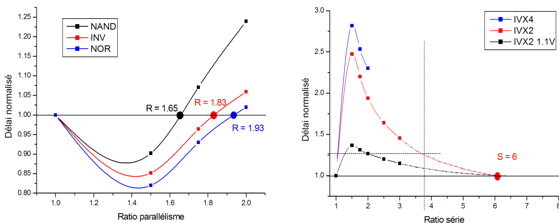
Figure 2.22 – Simulation du délai sur le chemin logique rFO4 à 350mV pour la mise en parallèle et la mise en série.
