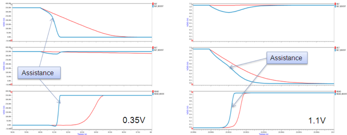
Figure 4.26 – Temps de lecture à 0.35V (gauche) et 1.1V (droite) obtenus avec l’utilisation de l’assistance à la lecture, en condition SS.
