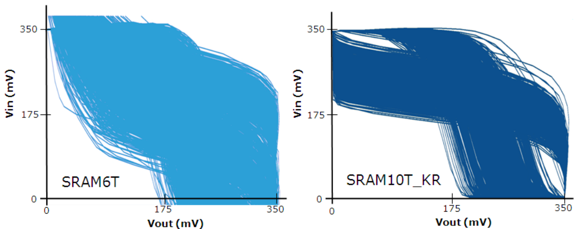
Figure 4.13 – Courbes en papillon des cellules 6T et 10T_KR après 1000 tirages Monte-Carlo.
