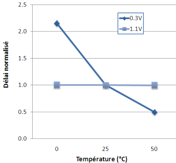
Figure 2.15 - Simulation du délai en fonction de la température du chemin logique qFO4.
