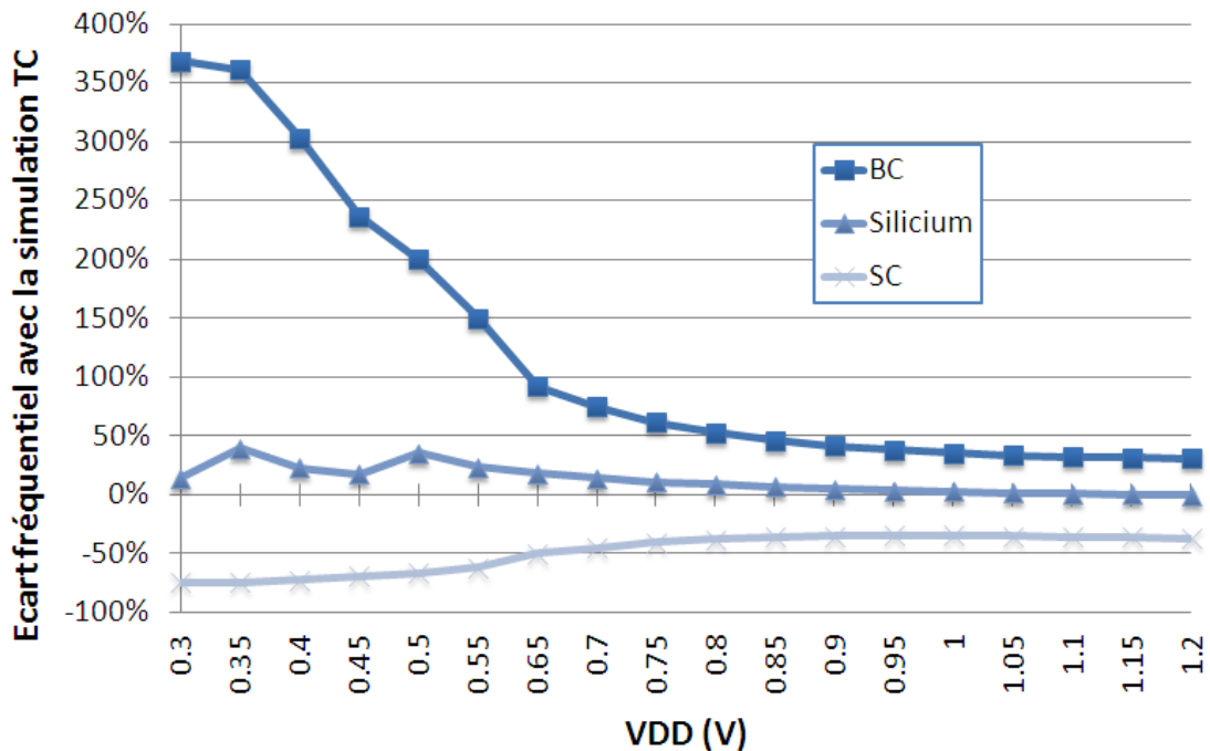
Figure 3.13 – Écart fréquentiel de la simulation BC et WC et des mesures silicium avec la simulation TC.
