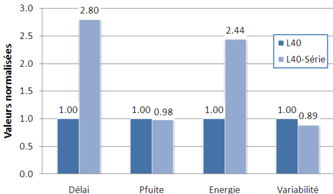
Figure 2.28 – Résultats de la simulation du qFO4 à 350mV pour les stratégies standards et mise en série systématique.
