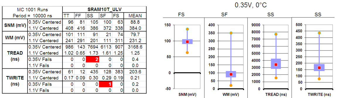
Figure 4.18 – Simulation Monte-Carlo sur l'ensemble des points de caractérisation, avec affichage du moins bon résultat (gauche). La distribution des différentes caractéristiques est affichée en box-plot (droite).
