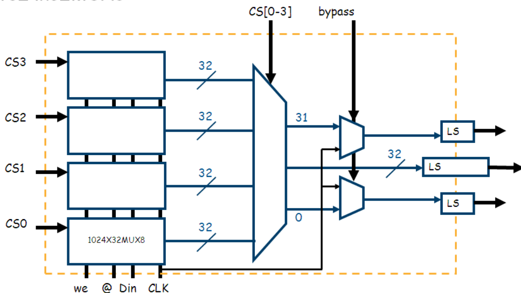
Figure 4.31 – Représentation schématique du démonstrateur mémoire.
