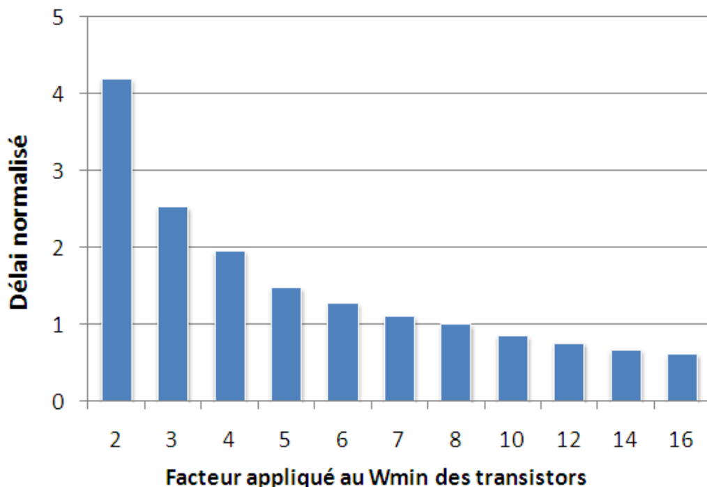
Figure 2.18 – Délai en fonction de W simulé sur rFO4.
