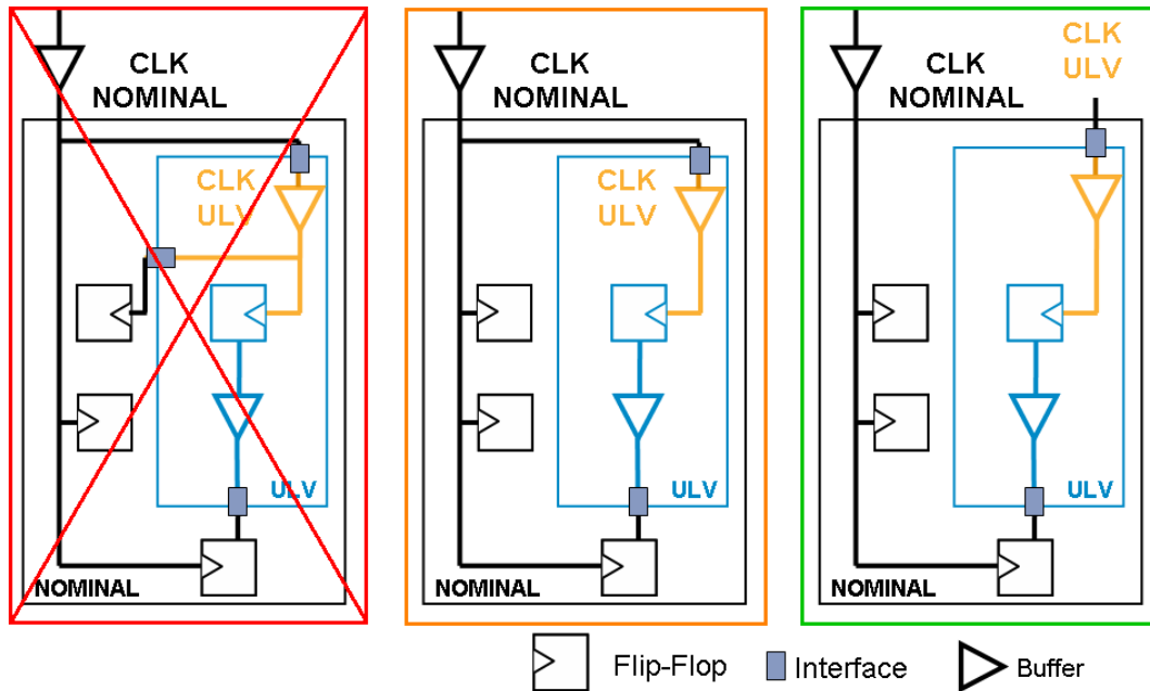
Figure 3.14 – Arbre d'horloge avec branches croisées (gauche), branches dédiées (centre), et arbres d'horloge dédiés (droite).
