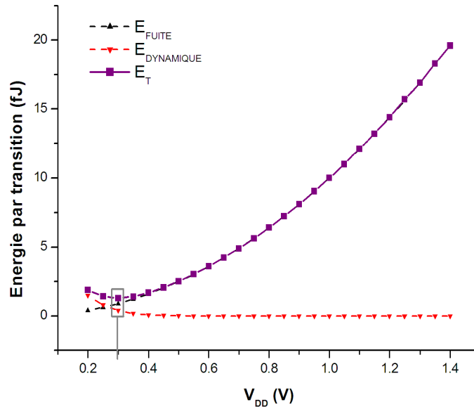
Figure 1.5 – Énergie totale par transition en fonction de la tension
