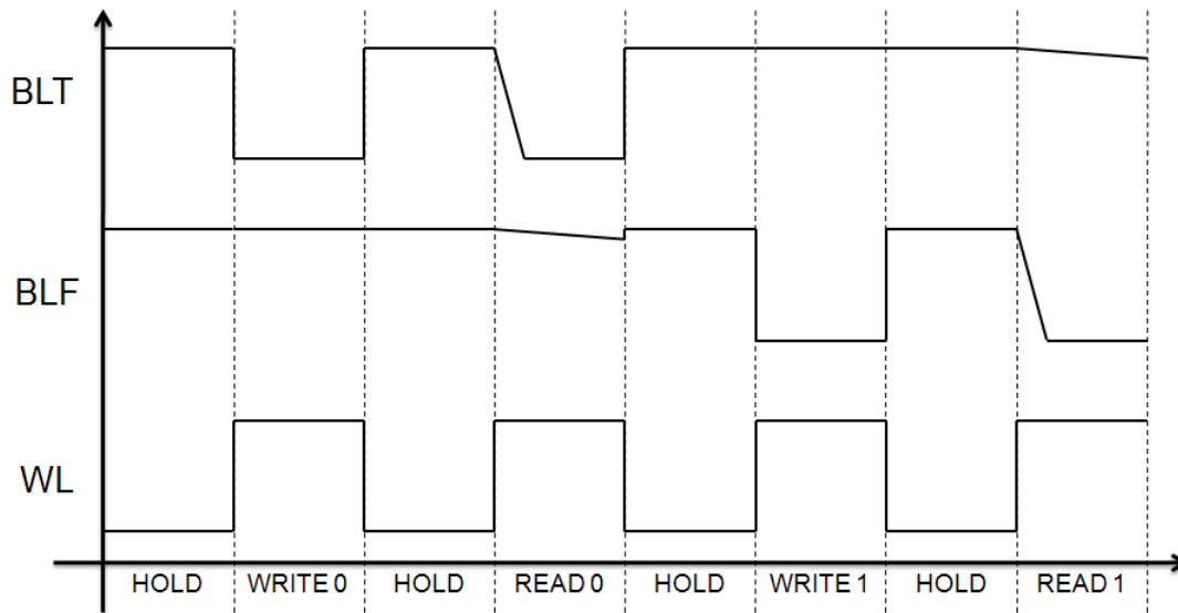
Figure 4.8 – Méthodologie de simulation dynamique des cellules mémoires.
