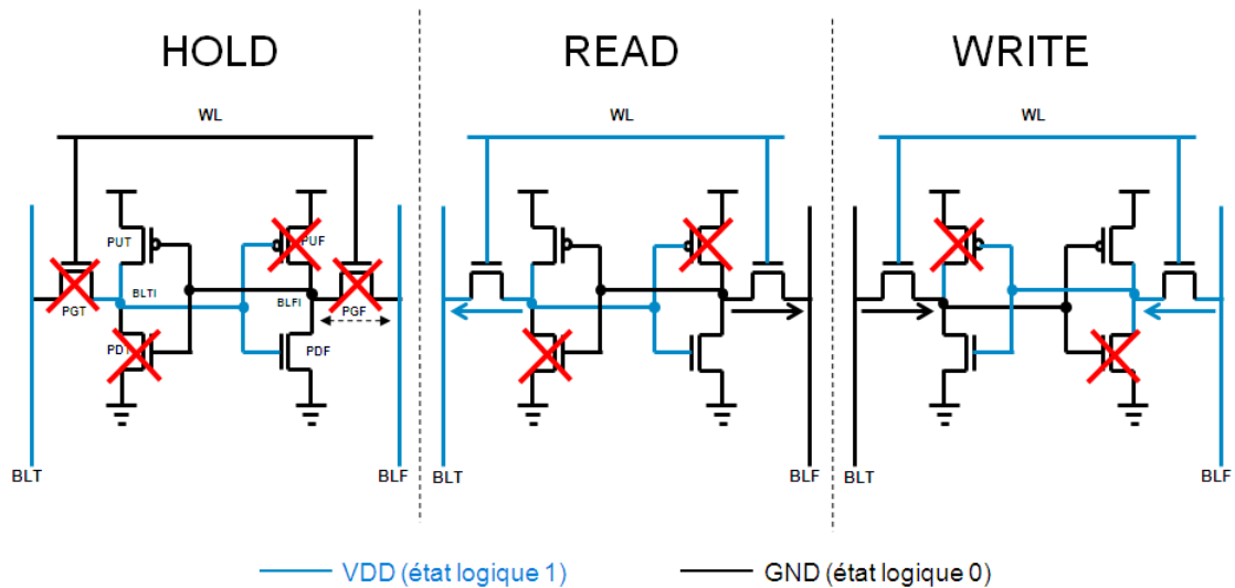
Figure 4.2 – Opérations de maintien (gauche), lecture (centre) et écriture (droite) d’une cellule SRAM 6T.
