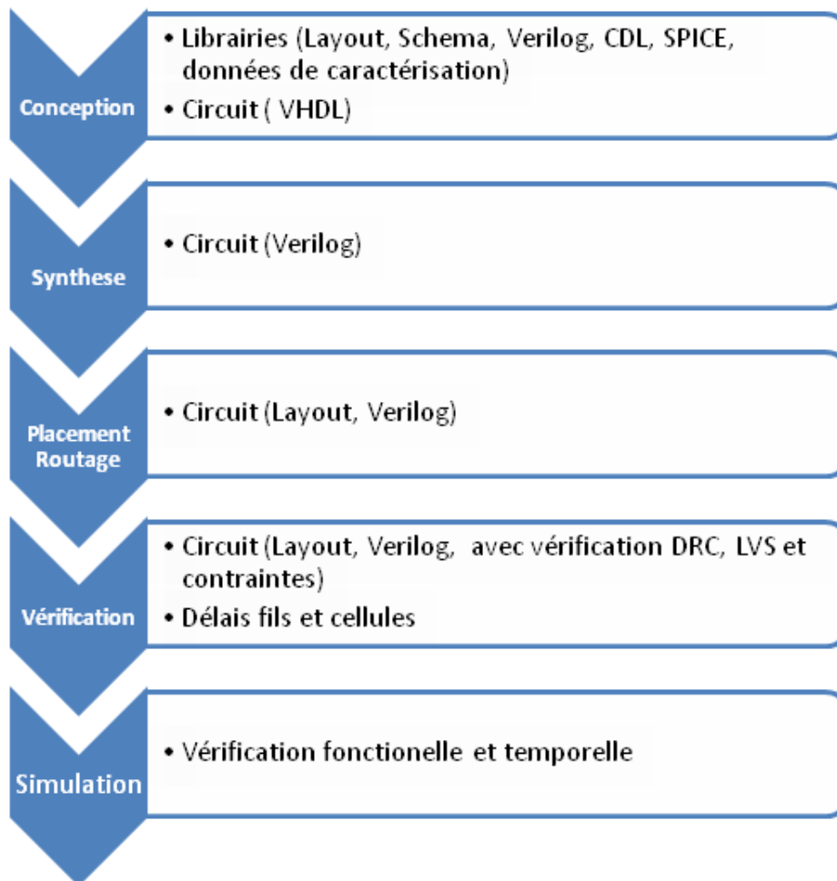
Figure 3.1 – Représentation du flot de conception d'un circuit numérique.
