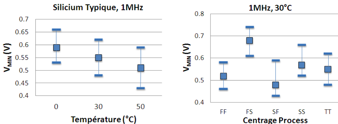
Figure 3.7 – Mesures sur silicium de V_{MIN} sur le QLIBD en fonction de la température (gauche) et en fonction du centrage process (droite).
