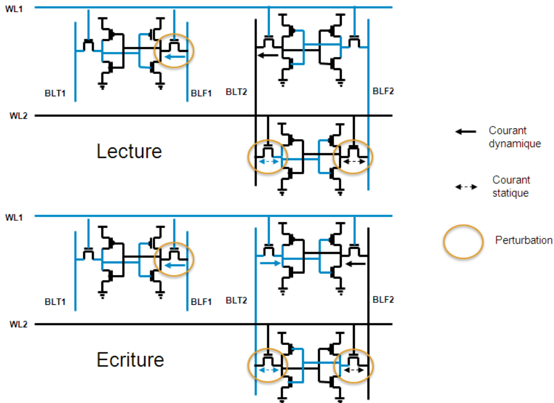
Figure 4.3 – Phénomènes de perturbation au voisinage de la cellule accédée.
