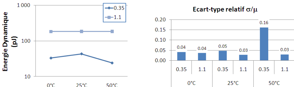
Figure 2.40 – Mesure sur silicium de l'énergie dynamique (gauche) et de la variabilité (droite) d'un oscillateur, en fonction de la température.
