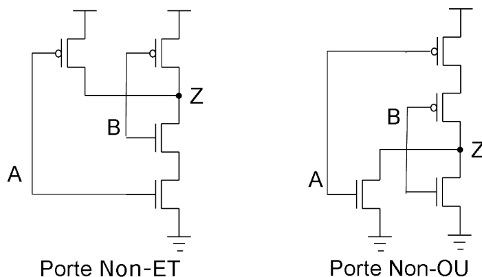
Figure 2.21 – Réseaux de transistors des portes logiques Non-ET et Non-OU.
