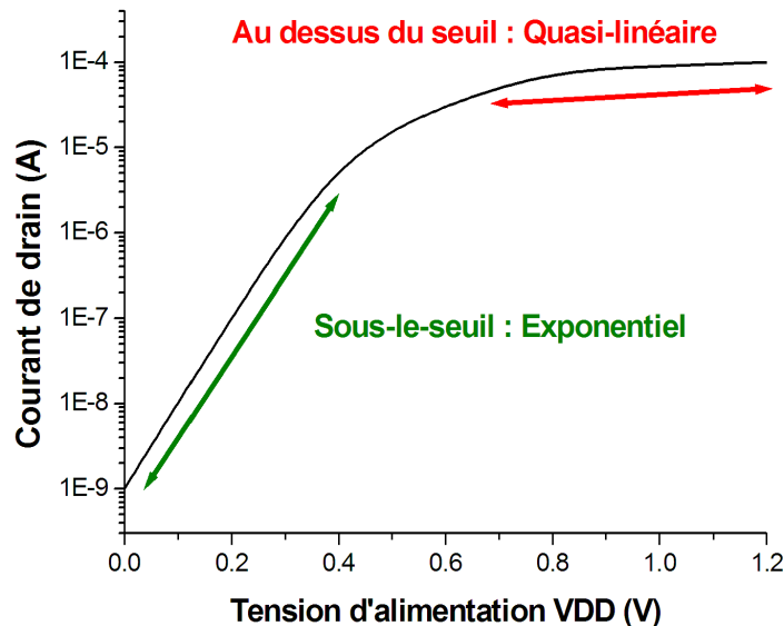
Figure 1.3 – Courant de drain en fonction de la tension V_{DD}
