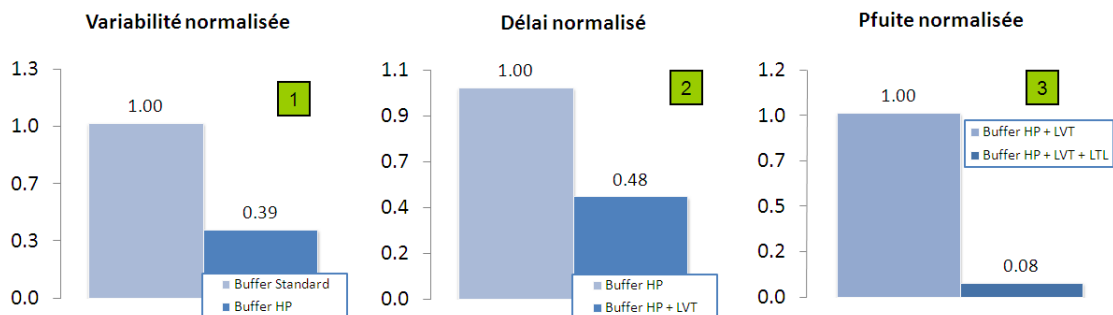
Figure 2.34 – Effet de chaque solution simulé à 350mV : HP = Hautement parallélisé, LTL = L Très Longue.
