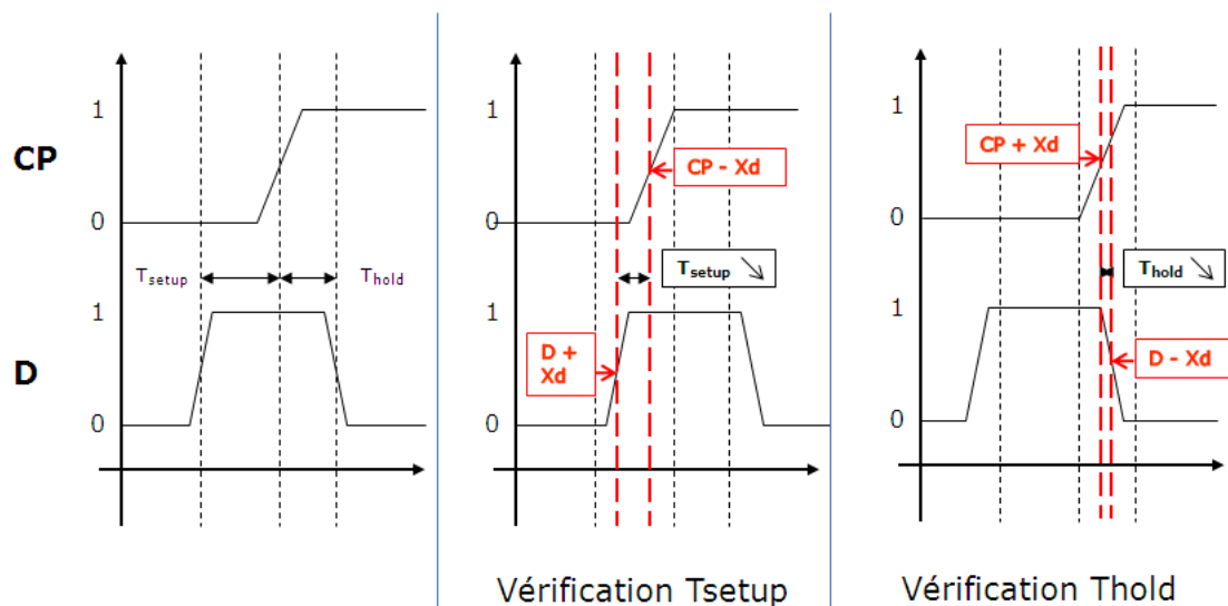
Figure 3.12 – Description du principe du facteur homothétique pour la vérification des contraintes.
