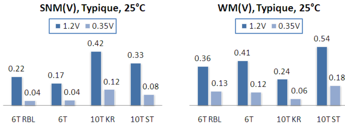
Figure 4.11 – Simulation de la SNM (gauche) et de la WM (droite).
