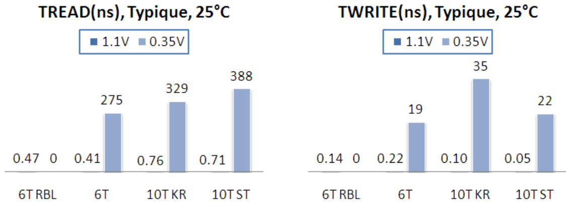
Figure 4.12 – Simulation de TREAD (gauche) et de TWRITE (droite).
