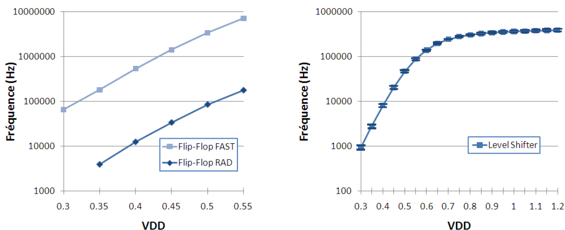
Figure 2.38 – Mesure sur silicium des oscillateurs de Flip-Flops (gauche) et de l’oscillateur composé de convertisseurs de tension (droite), à 25°C.
