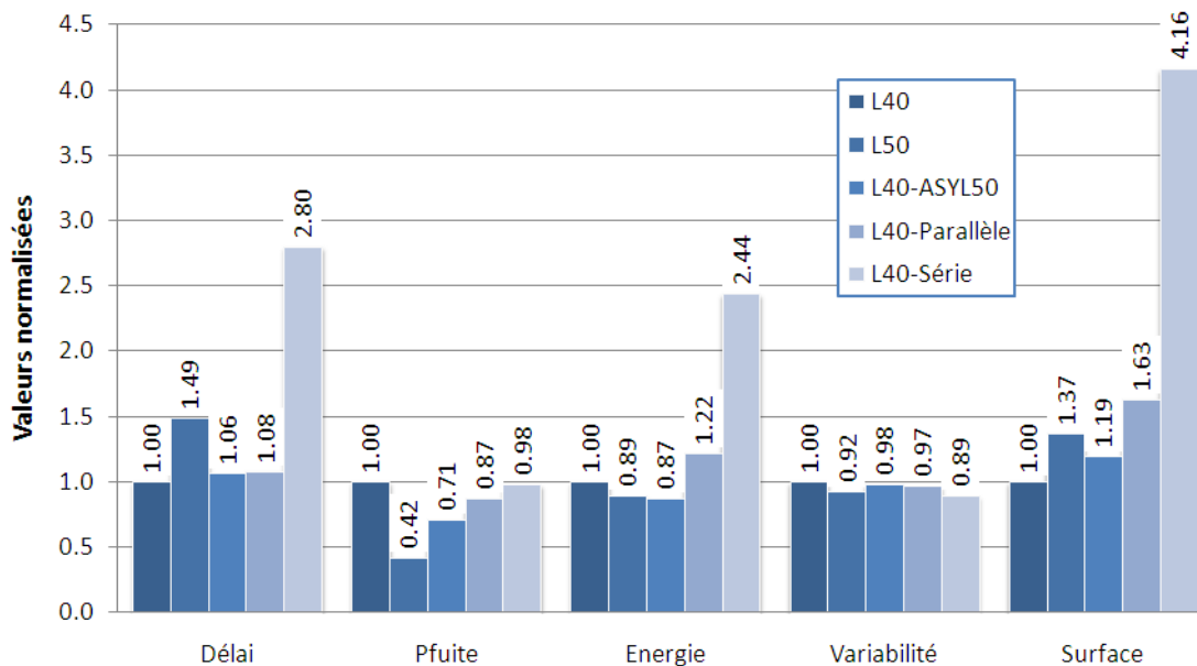
Figure 2.29 – Résultats de la simulation du qFO4 à 350mV pour les différentes stratégies.
