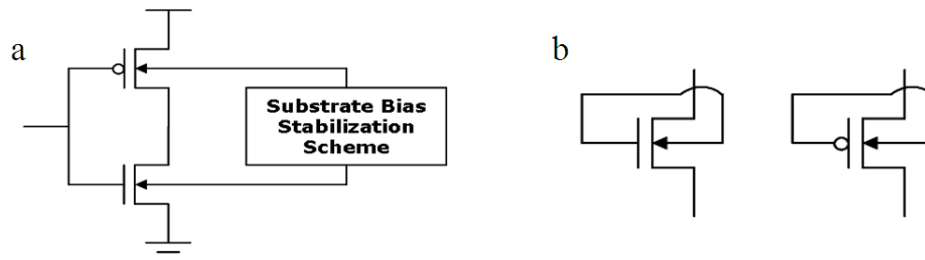
Figure 1.7 – Logique (a) VT-CMOS et (b) DT-CMOS
