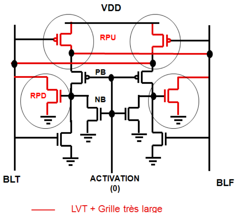
Figure 4.24 – Représentation schématique de la solution d’assistance à la lecture.
