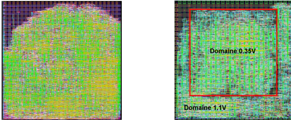
Figure 3.4 – Placement mono-domaine (gauche) et multi-domaines (droite).
