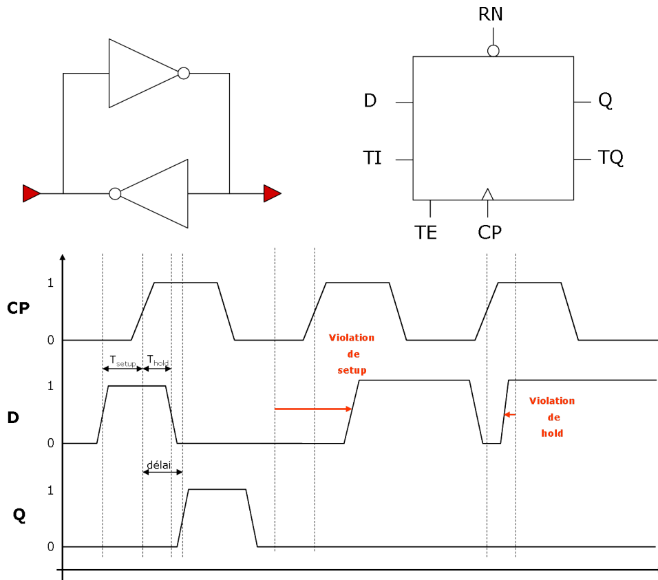
Figure 2.30 – Principe de la mémorisation (gauche), symbole d'une flip-flop (droite), et chronogramme de son fonctionnement.
