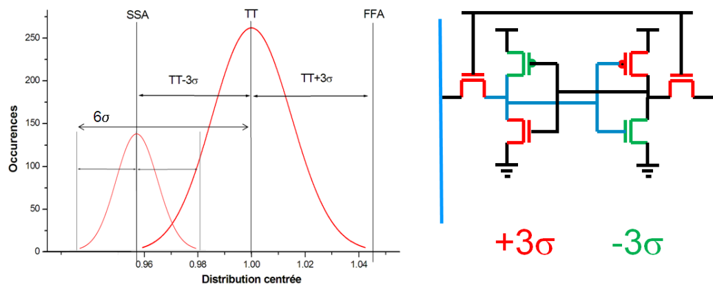
Figure 4.5 – Simulation Monte-Carlo de la SNM à 6\sigma (gauche), et application de la méthodologie paramétrique (droite).
