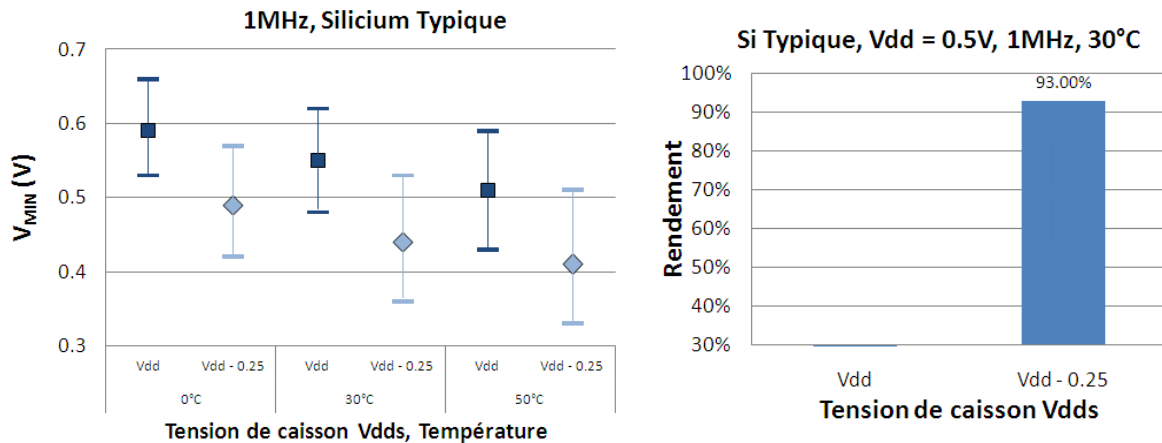
Figure 3.9 – Mesures sur silicium avec et sans Body-Biasing pour compenser les variations liées à la température (gauche), et observation de l'impact sur le rendement (droite).
