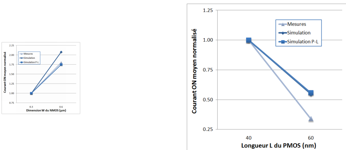
Figure 2.5 – Variation du courant dynamique en fonction de la dimension W des sources/drains et de la longueur de grille L. Mesurée à 350mV.
