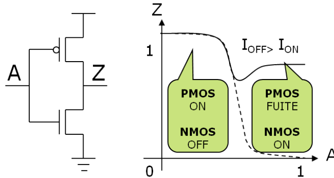
Figure 1.4 – Représentation de l'effet du rapport I_{ON}/I_{OFF} sur le fonctionnement d'un inverseur CMOS.
