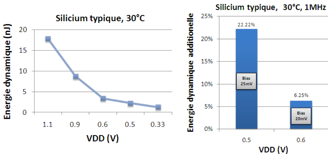
Figure 3.10 – Mesures sur silicium de l'énergie dynamique (gauche) et de l'impact du Body-Biasing (droite).
