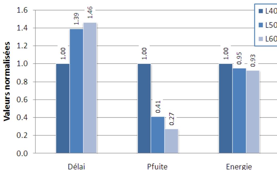
Figure 2.19 – Résultats de la simulation du qFO4 à 350mV pour plusieurs longueur de grille L.
