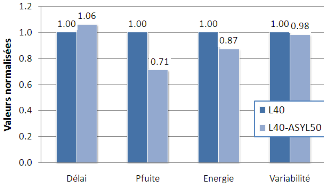
Figure 2.25 – Résultats de la simulation du qFO4 à 350mV pour les stratégies standards et asymétriques.
