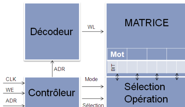
Figure 4.21 – Représentation schématique d'une mémoire SRAM. Le signal "Mode" décrit le type d'opération effectué, WE est l'horloge d'activation de l'écriture, CLK est l'horloge globale, ADR est l'adresse du mot.
