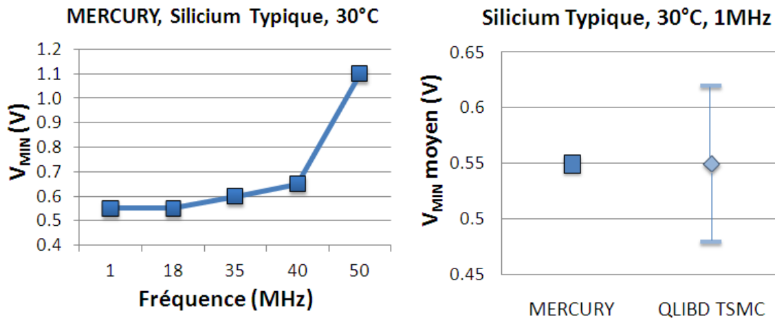
Figure 3.6 – Mesures des circuits MERCURY et QLIBD : Tension minimale en fonction de la fréquence (gauche) et Tension minimale à 1MHz (droite).
