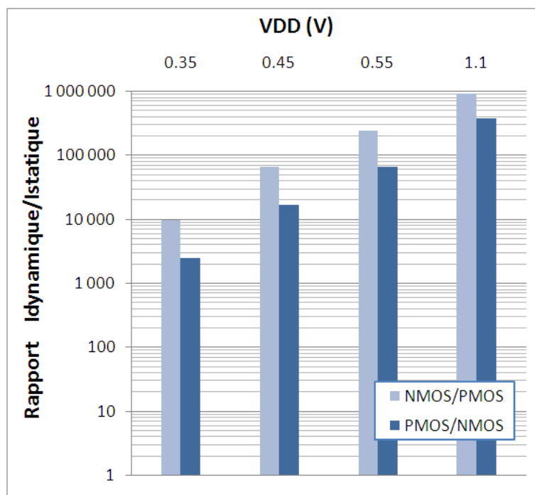
Figure 2.6 – Évolution du rapport I_{Dynamique}/I_{Statique} entre le NMOS et le PMOS en fonction de la tension d’alimentation.
