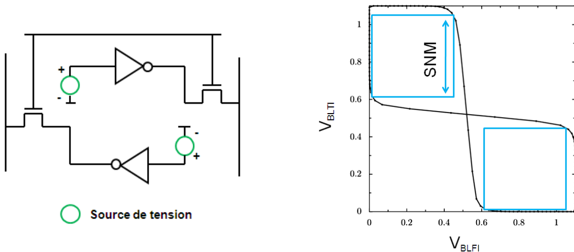
Figure 4.4 – Représentation schématique de la simulation (gauche) et de la figure en papillon (droite) permettant d'extraire la SNM.
