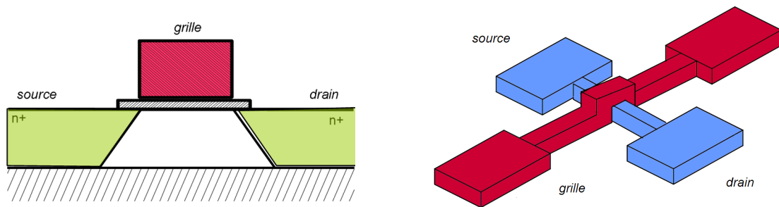
Figure 1.6 – Exemple d'un transistor sur substrat SOI (gauche) et FinFET (droite)
