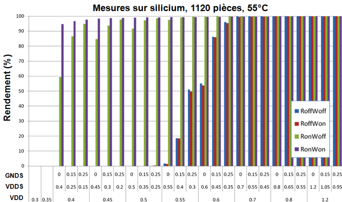
Figure 4.36 – Mesures sur silicium du rendement du démonstrateur à 55°C, en fonction de la tension d'alimentation, du Forward Body-Biasing appliqué, et de l'état d'activation des assistances.
