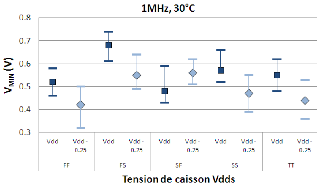
Figure 3.8 – Mesures sur silicium avec et sans Body-Biasing pour compenser les variations liées à la fabrication.
