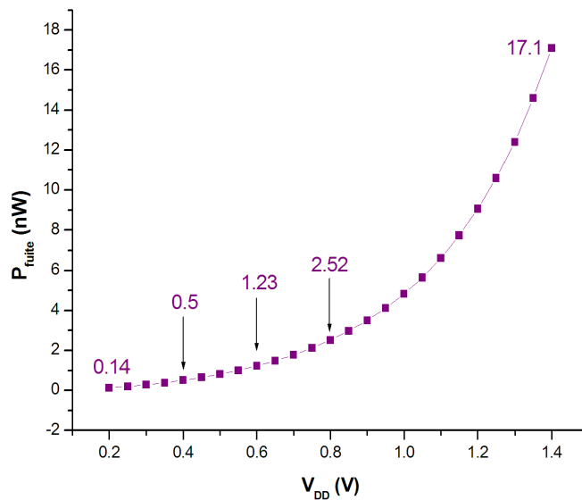
Figure 2.10 – Fuites de la chaîne qF04 en fonction de la tension d’alimentation.
