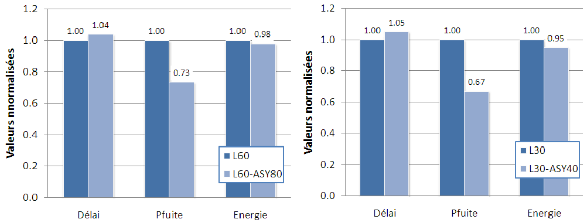
Figure 2.36 – Simulation du chemin logique qFO4 à 350mV, pour les technologies 65nm et 32nm.
