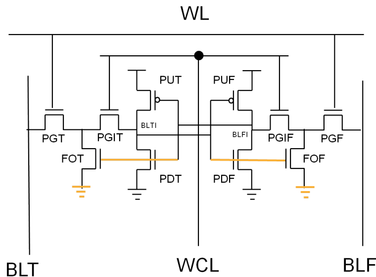
Figure 4.14 - Proposition d'une architecture à 10 transistors, SRAM10T_ULV.
