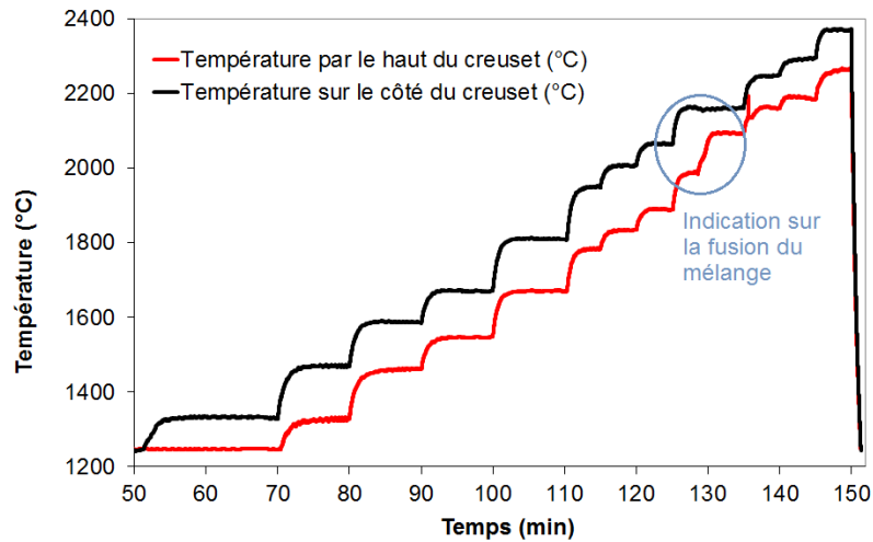
Figure 6-28 : Courbe de températures (température en fonction de la durée de l'essai) enregistrée au cours de l'essai CORSICCA 2_Eu_1e relatif à l'interaction 25% \text{UO}_2 – 75% \text{Eu}_2\text{O}_3 (composition massique) dans un creuset en tungstène, dans le but de retrouver l'eutectique reporté par L.N. Grossman et al. La température maximale de l'essai était de 2370 \pm 35^\circ\text{C} . Aucun palier de solidification n'est visible au refroidissement.
