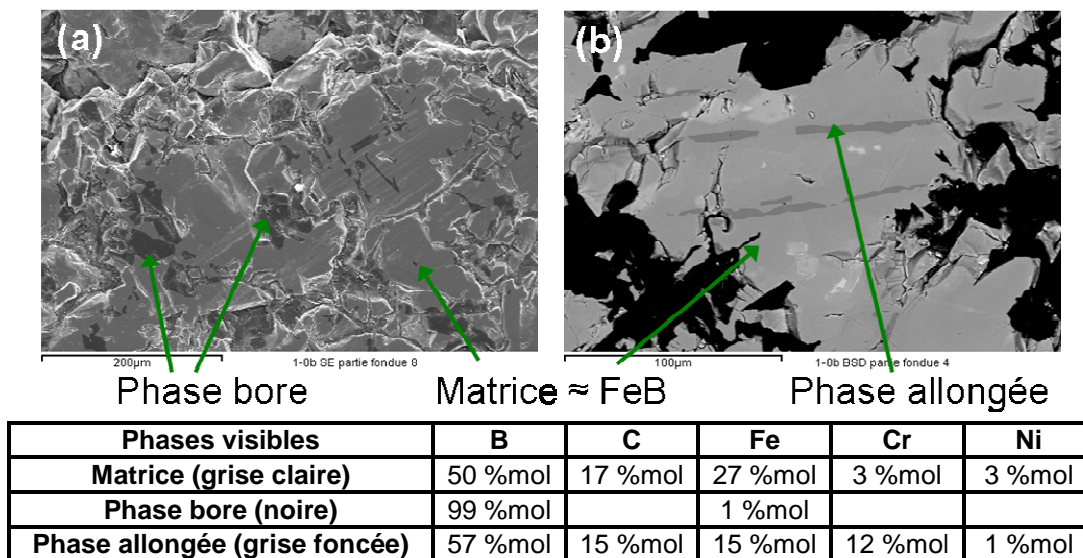
Figure 6-5 : Photos MEB de la charge fondue Acier inoxydable – B 4 C après le refroidissement avec l'analyse chimique EDX. Trois phases ont été révélées : la matrice contenant majoritairement du fer, du bore et du carbone (en gris clair), la phase bore pure (en noir sur l'image (a)) et la phase allongée enrichie en chrome, contenant du fer, du chrome, du bore et du carbone (en gris foncé sur l'image (b) en électrons rétrodiffusés)
