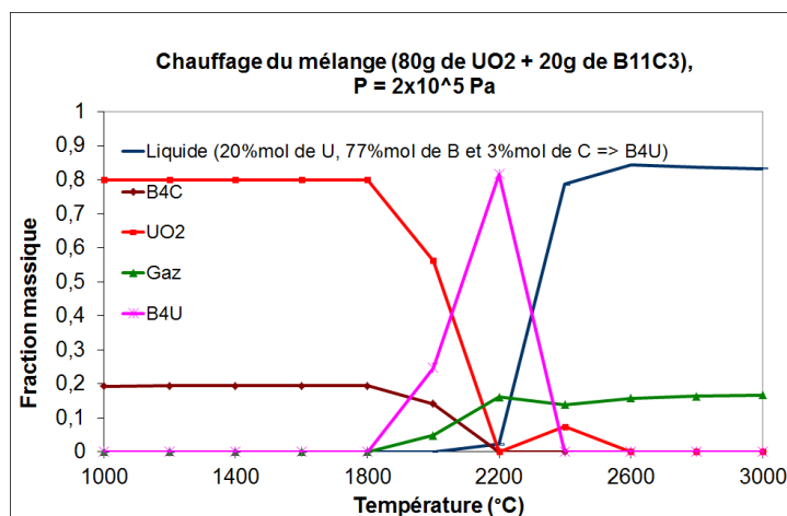
Figure 4-2: L'évolution des fractions massiques du système (20% B 11 C 3 – 80% UO 2 ) à l'équilibre, à 2·10 5 Pa, en fonction de la température du milieu
