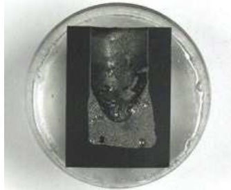
Figure 6-3 : Section longitudinale du creuset en graphite après refroidissement avec la charge fondue Acier inoxydable – B_4C . Le diamètre externe du creuset est de 25 \text{ mm} .
