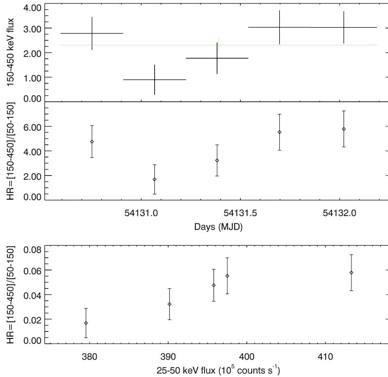
FIGURE 6.4 – Haut : Courbe de lumière SPI dans la bande 150 – 450 keV avec une échelle de temps de \sim 7 h. Le flux est donné en unités de 10^5 counts s^{-1} . La croix verte indique le flux moyen et son incertitude. Milieu : Rapport de dureté à haute énergie (i.e. [150 – 450]/[50 – 150] keV) en fonction du temps. Bas : Rapport de dureté à haute énergie en fonction du flux dans la bande 25 – 50 keV.
