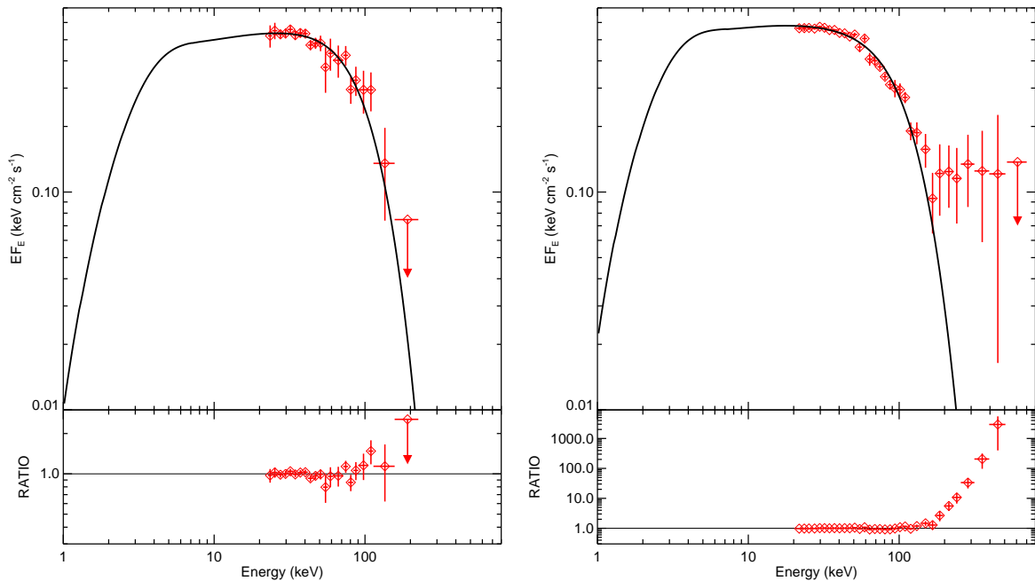
FIGURE 7.4 – Gauche : spectre de l'épisode 119–122 ajusté avec un modèle de Comptonisation thermique (COMPPT). Droite : spectre moyen ajustée avec le même modèle ; l'excès à haute énergie est clairement visible.
