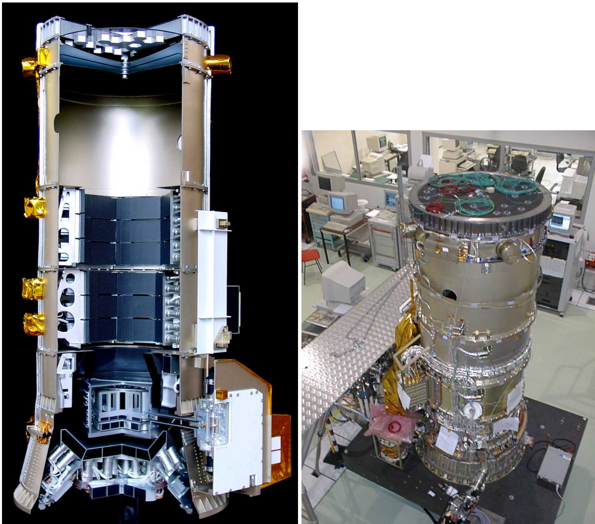
FIGURE 4.3 – Gauche : Vue détaillée de la structure du spectromètre SPI. Droite : Photo de l'instrument lors de la phase de calibration.
