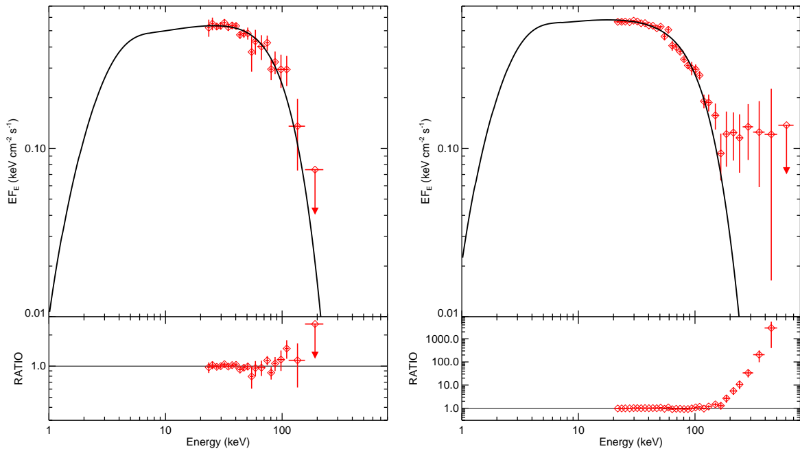
FIGURE 7.4 – Gauche : spectre de l'épisode 119–122 ajusté avec un modèle de Comptonisation thermique (COMPTR). Droite : spectre moyen ajustée avec le même modèle ; l'excès à haute énergie est clairement visible.
