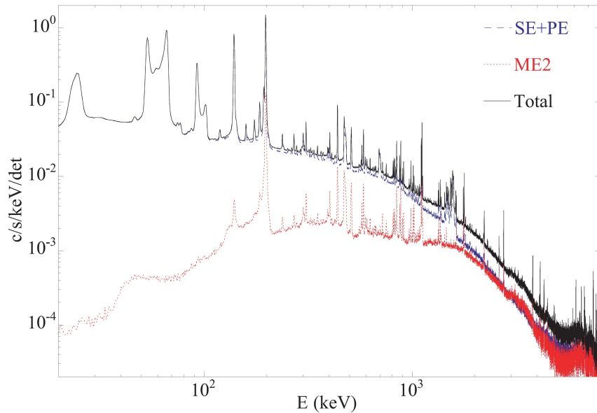
FIGURE 4.7 – Bruit de fond de l'instrument SPI. La courbe bleue correspond aux événements simples et inclut les PE, événements qui ont été discriminés par la PSD. La courbe rouge correspond aux événements doubles et la courbe noire représente le spectre moyen total des coups dues au bruit de fond. La figure est tirée de Jean et al. (2003).
