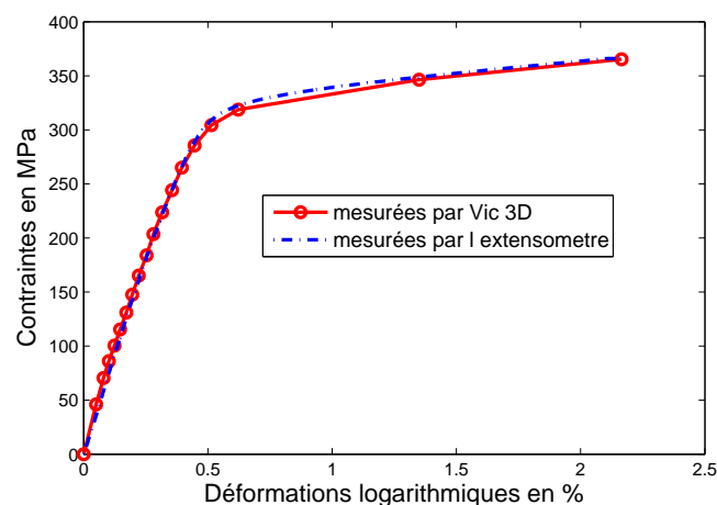
Figure 4.2 – Comparaison des déformations mesurées par Vic-3D et par l'extensomètre dans le domaine élasto-plastique lors d'un essai de traction sur l'alliage 2024-T3
