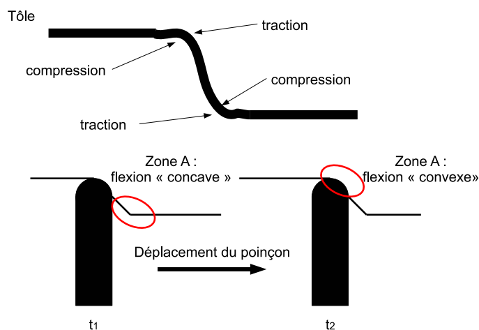
Figure 1.33 – Représentation des cycles de flexion subit par la tôle
