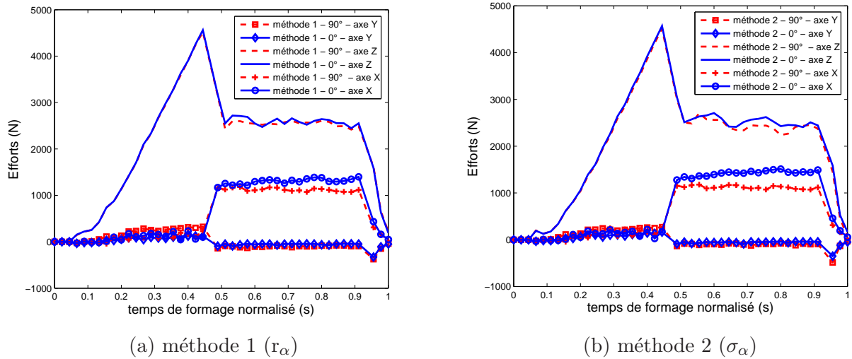
Figure 6.17 – Evolution des efforts lors de la simulation de la mise en forme de l'essai de référence à partir de deux jeux de paramètres du critère différents et dans les directions 0^\circ et 90^\circ
