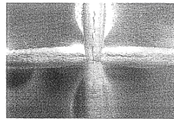
Figure 1.37 – Fissuration typique provenant d'un test B (vue arrière de la partie emboutie) [FIL 02]
