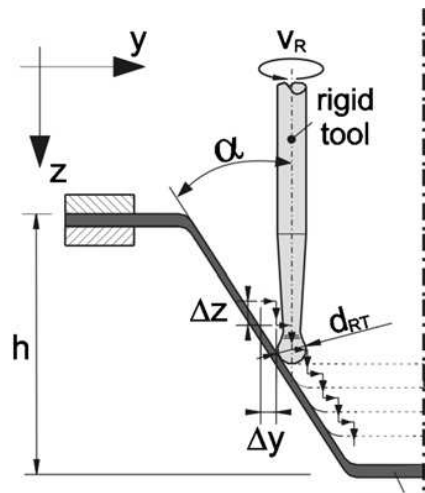
Figure 1.19 – Description des incréments verticaux et horizontaux [PET 09]
