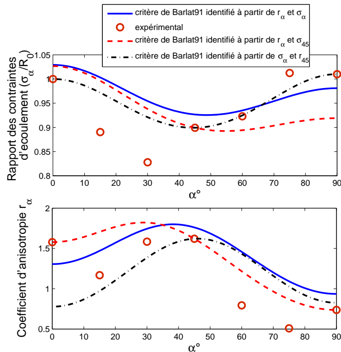
Figure 4.20 – Evolution du coefficient d'anisotropie et de la limite d'élasticité en fonction de l'angle \alpha pour l'alliage Al-Li
