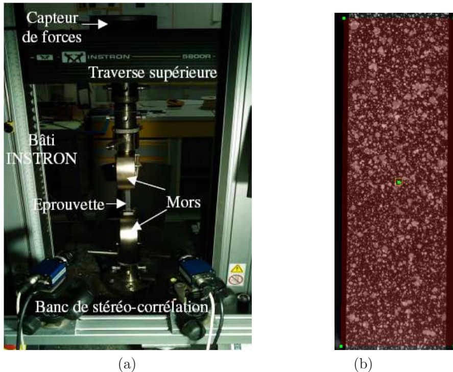
Figure 4.1 – Machine d'essais électromécanique de traction INSTRON 5800 (a), et présentation de l'AOI de l'éprouvette (b)
