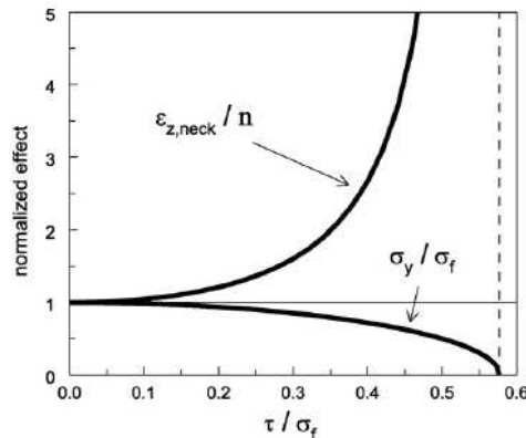
Figure 1.31 – Effets de l'ajout de contraintes de cisaillement sur la formabilité. Ligne du dessous : limite d'élasticité du matériau \sigma_y ; ligne du dessus : déformation limite normalisée pour l'apparition de la striction \epsilon_z . \sigma_f =contrainte équivalente, \tau =contrainte de cisaillement, n =coefficient d'écroûissage. [TEK 06]
