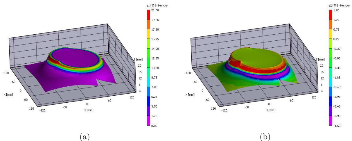
Figure 3.16 – Déformations principales d'Hencky (en %) maximales, \epsilon_1 (a) et minimales, \epsilon_2 (b)
