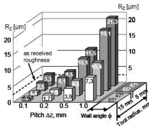
Figure 1.54 – Influence de l'incrément \Delta z , de l'angle de mise en forme et la taille du diamètre du poinçon sur la rugosité R_z [JUN 03]
