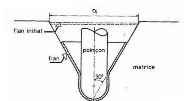
Figure 1.12 – Schéma de principe de l'essai Fukui [ARR 81]
