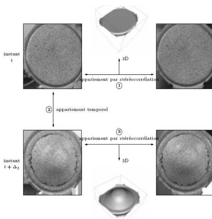
Figure 2.9 – Principe de la stéréo-corrélation [GAR 01]
