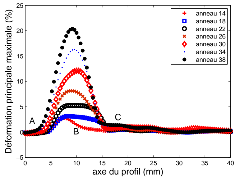
Figure 3.17 – Evolution de la déformation principale maximale le long du profil en formage positif
