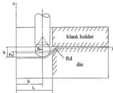
Figure 1.45 – Principe de la sphère libre au bout du poinçon [KIM 02]
