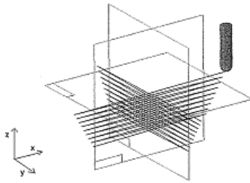
Figure 1.36 – Essai B, chemin du poinçon pour un étirement purement bi-axial [FIL 02]
