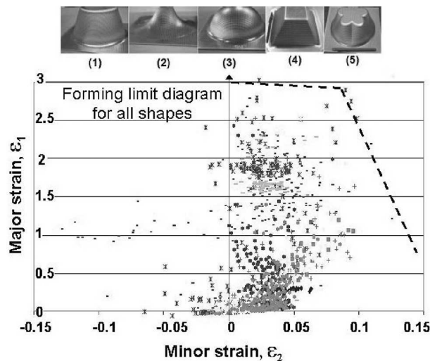
Figure 1.41 – Diagramme limite de formage pour les cinq formes [JES 05B]
