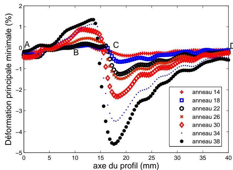
Figure 3.18 – Evolution de la déformation principale minimale le long du profil en formage positif
