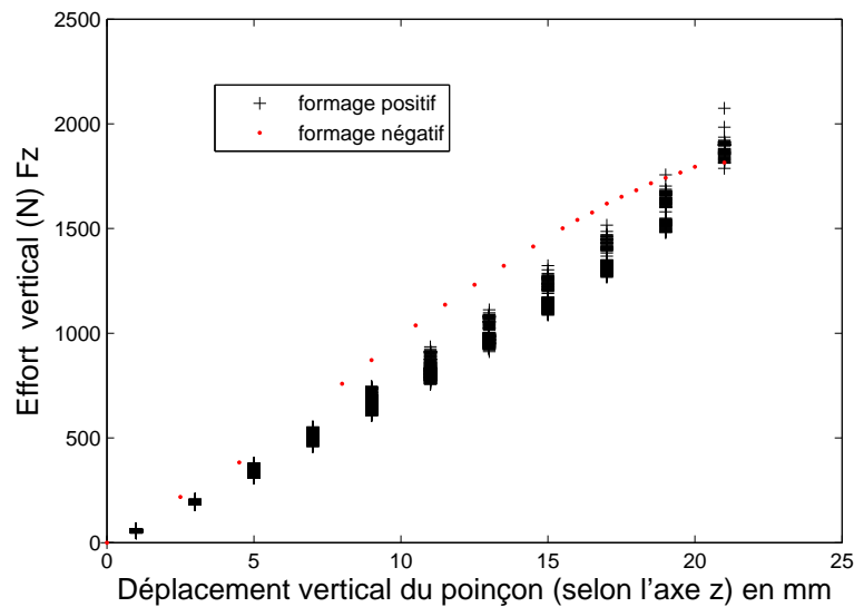
Figure 3.22 – Comparaison entre le formage positif et négatif de l'évolution de la force en fonction du déplacement vertical du poinçon
