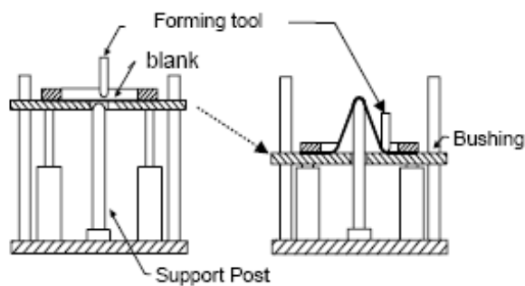
Figure 1.21 – Principe du formage incrémental deux points [MAT 94]
