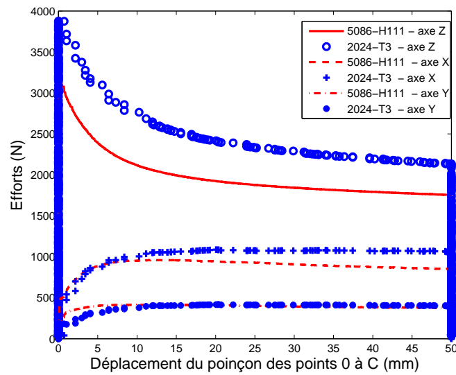
Figure 6.5 – Comparaison de l'évolution des efforts selon les axes Y, X et Z en fonction du déplacement du poinçon pour les alliages 5086-H111 et 2024-T3
