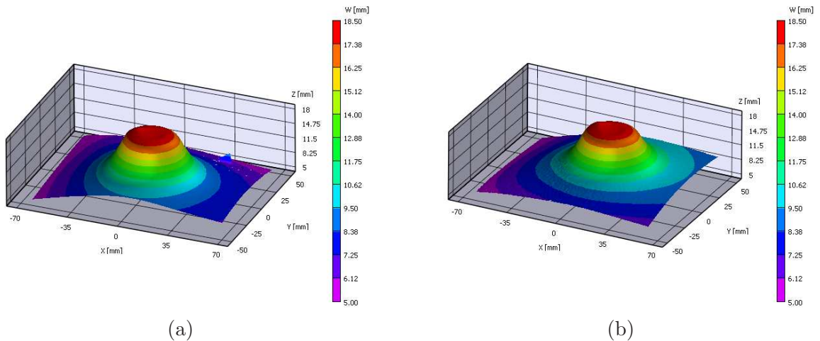
Figure 3.45 – Formes finales des deux pièces obtenues juste avant rupture pour les deux trajectoires du poinçon, circulaire sens horaire (a) circulaire alternée (b)
