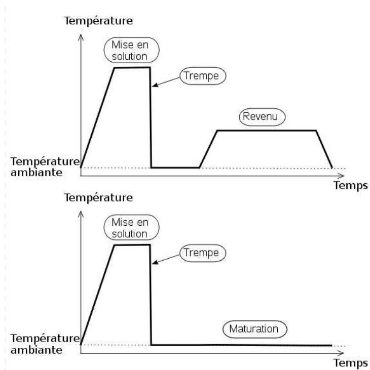
Figure 2.12 – Cycles de traitement thermique des alliages d'aluminium [BAI 00]
