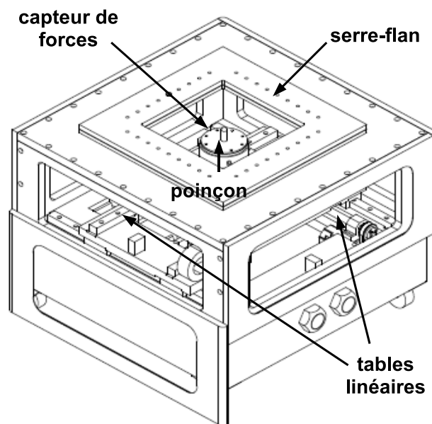
Figure 2.1 – Modèle CAO du pilote SPIF
