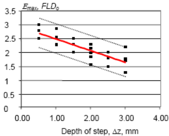
Figure 1.40 – \varepsilon_1 en fonction de \Delta z [MIC 04]
