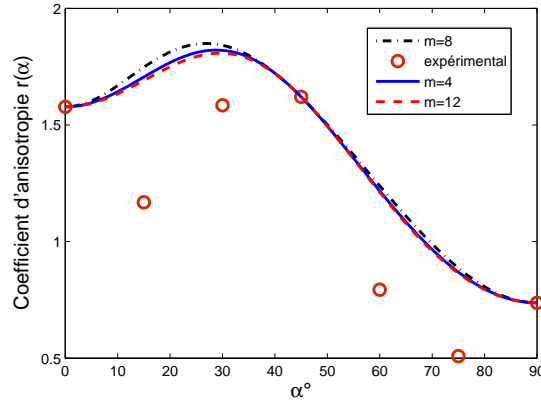
Figure 4.19 – Evolution du coefficient d'anisotropie identifié à partir des r_\alpha et de \sigma_{45} en fonction de l'angle \alpha pour l'alliage Al-Li pour différentes valeurs du paramètre m
