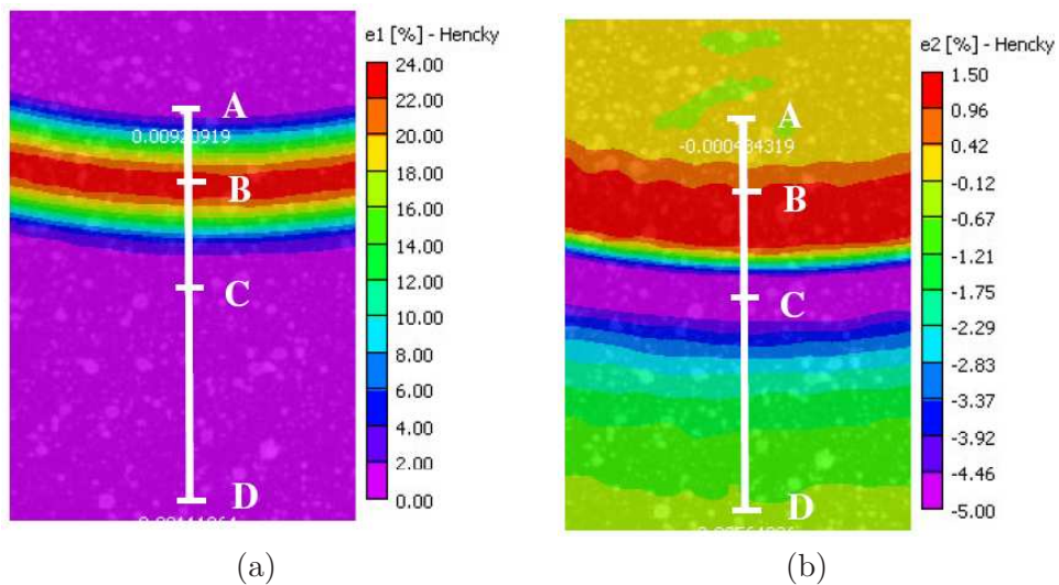
Figure 3.10 – Localisation du profil étudié sur les cartographies de déformations principales maximales (a) et minimales (b)
