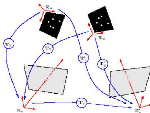
Figure 2.8 – Calibrage d'un capteur de stéréo-corrélation avec deux positions de mire [GAR 01]
