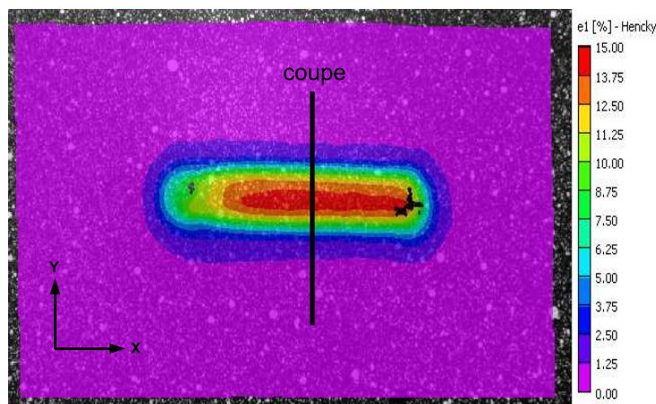
Figure 6.6 – Déformations principales maximales, AOI du deuxième banc stéréoscopique et localisation du profil étudié (point C, 5086-H111)
