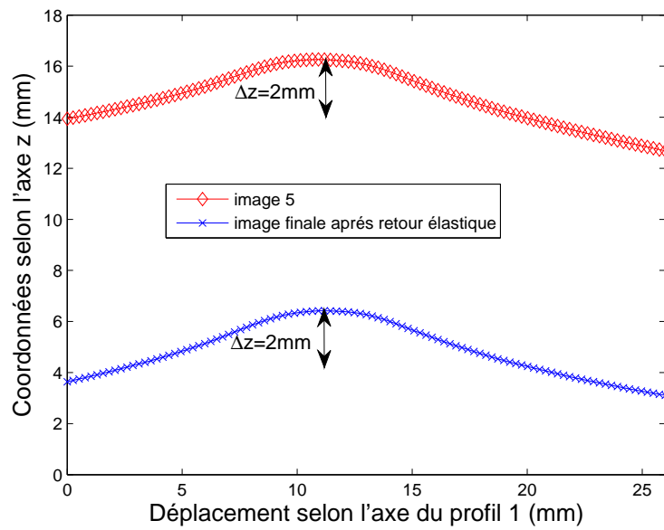
Figure 3.38 – Evolution des coordonnées selon l'axe z de la tôle le long du profil 1 au cours de la mise en forme de la pièce B
