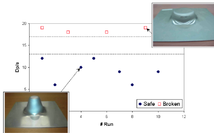
Figure 1.55 – Rapport diamètre du poinçon/épaisseur de la tôle pour chaque essai de formage incrémental [AMB 07]
