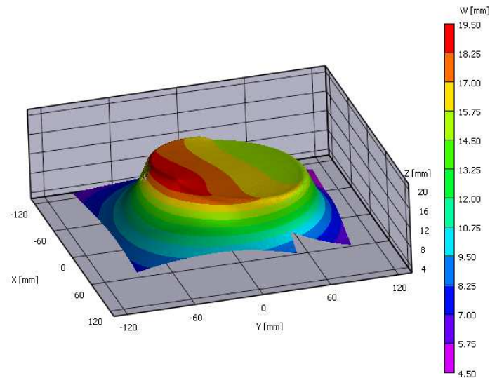
Figure 3.15 – Forme du tronc de cône mise en forme positivement
