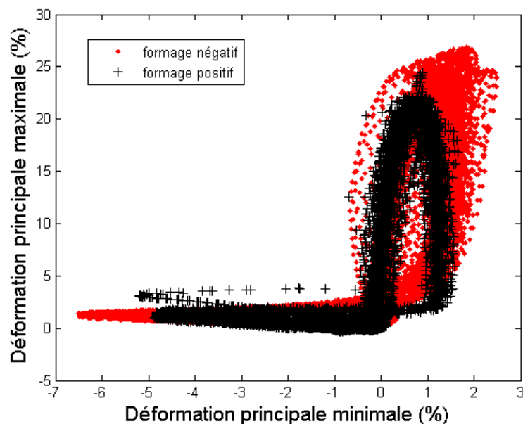
Figure 3.20 – Comparaison des déformations principales maximales en fonction des déformations principales minimales (%) entre le formage positif et négatif
