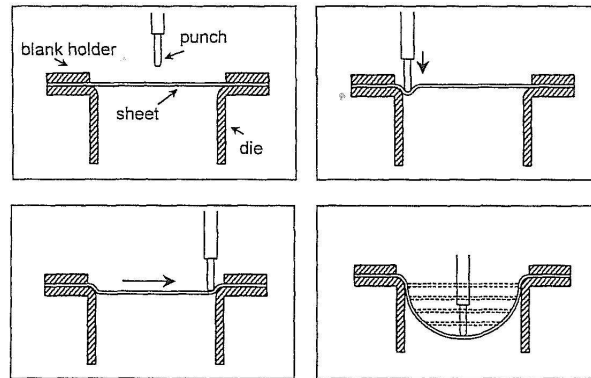
Figure 1.22 – Les différentes étapes du formage incrémental un point pour des trajectoires circulaires [KIM 00]
