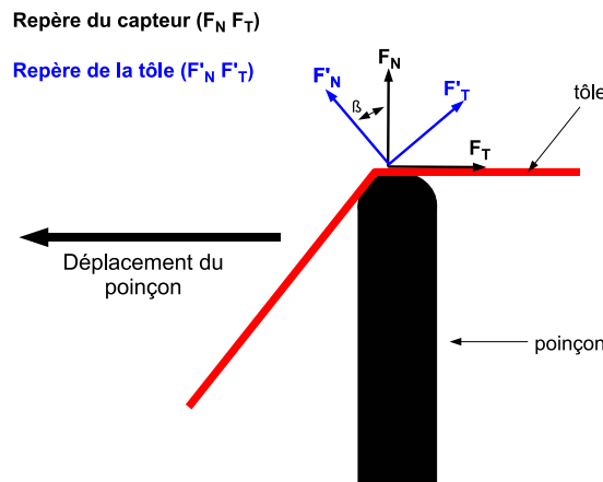
Figure 2.4 – Représentation des efforts normaux et tangentiels de la tôle lors de la mise en forme par rapport aux efforts mesurés par le capteur de force
