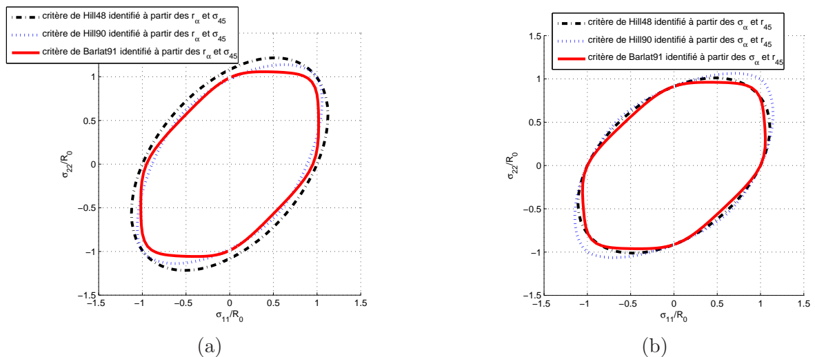
Figure 4.24 – Comparaison des surfaces de charge pour les critères de Hill48, Hill90 et Barlat91 identifiés à partir des r_\alpha (a) ou des \sigma_\alpha (b) pour l'alliage 2024-T3 pour un cisaillement nul ( \frac{\sigma_{12}}{R_0} )
