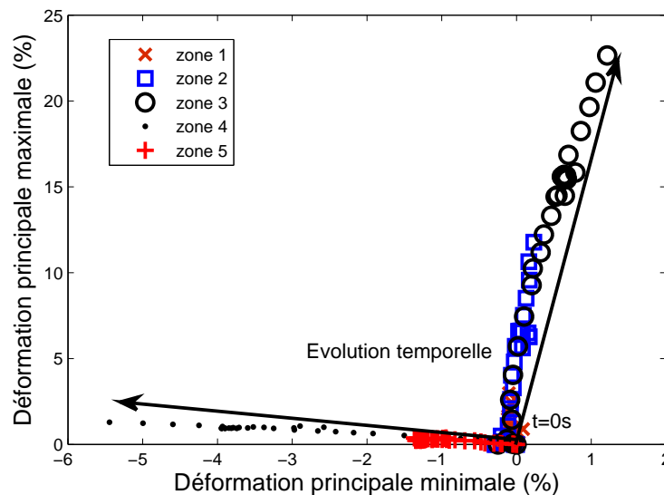
Figure 3.14 – Evolution des déformations au cours de la mise en forme négative du tronc de cône
