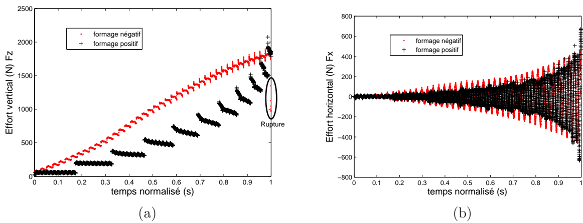
Figure 3.21 – Comparaison des efforts verticaux (a) et horizontaux (b) pour les mises en forme positives et négatives.
