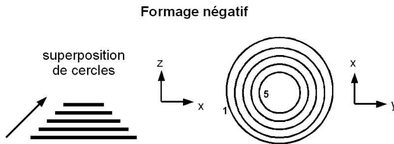
Figure 3.4 – Principe du formage négatif
