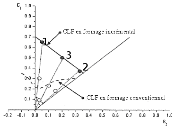
Figure 3.49 – Comparaison des courbes limites de formage obtenues par formage conventionnel et incrémental [FIL 02]
