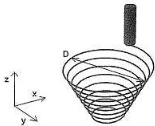
Figure 1.38 – Essai C, chemin du poinçon en spire 3-D [FIL 02]
