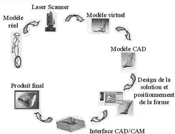
Figure 1.56 – Cycle de fabrication d'un support de cheville [FIL 05]
