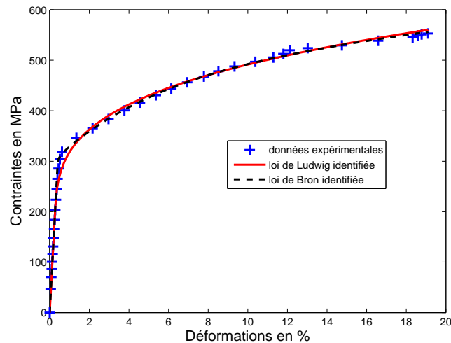
Figure 4.8 – Représentation des lois d'écroutissage de Ludwig et de Bron pour l'alliage 2024-T3 dans la direction 0^\circ
