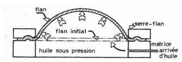
Figure 1.11 – Schéma de principe de l'essai Jovignot [ARR 81]
