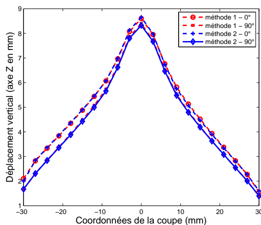
Figure 6.18 – Forme finale de la pièce après mise en forme de la tôle le long de la coupe perpendiculaire au déplacement horizontal du poinçon
