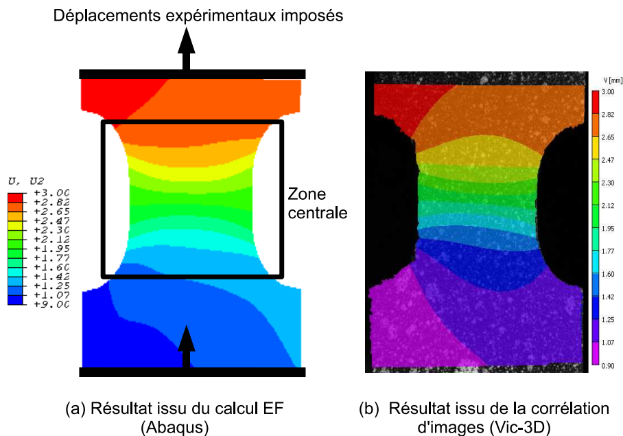
Figure 5.19 – Cartographie des champs de déplacements selon l'axe de traction simulée (a) et expérimentale (b) pour l'éprouvette Haddadi (image finale)
