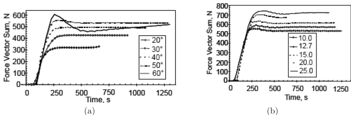
Figure 1.50 – Influence de l'angle de mise en forme et de la taille du diamètre du poinçon sur les efforts [DUF 05C]
