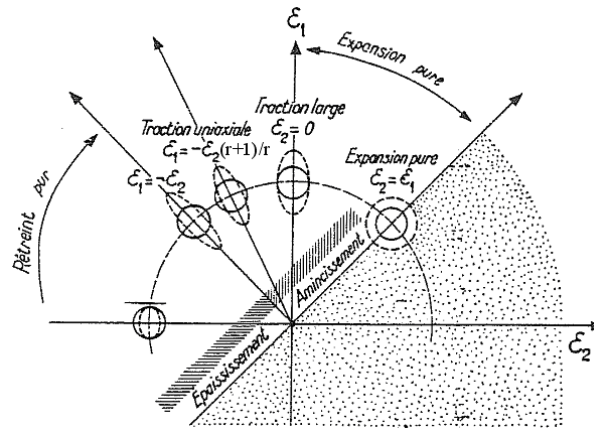
Figure 1.1 – Diagramme des déformations rencontrées en mise en forme des tôles [MAR 95]
