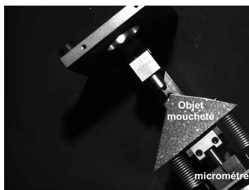
Figure 2.11 – Objet moucheté fixé au micromètre
