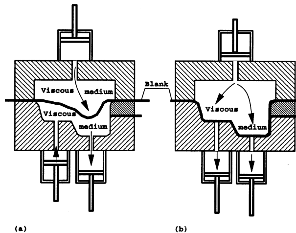
Figure 1.2 – Principe du procédé d'hydroformage, état initial (a) et état final (b) [ZHA 99]
