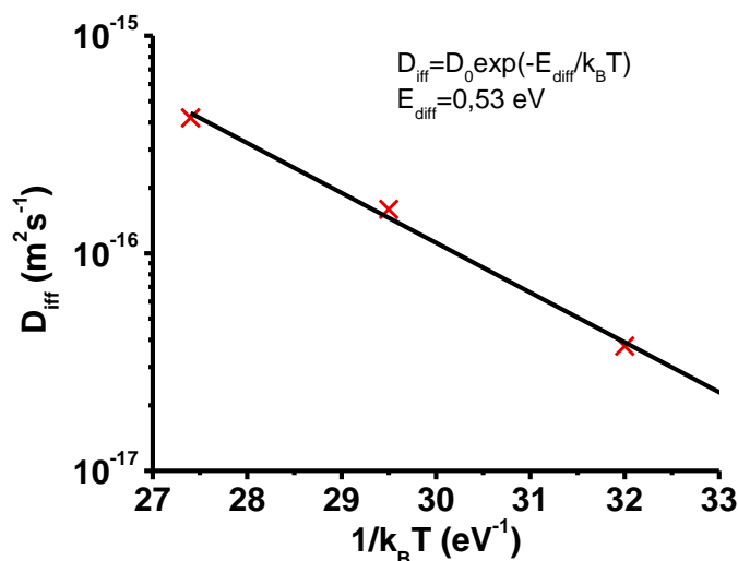
Figure IV-28 : Coefficient de diffusion extrait par le modèle du dipôle macroscopique et extraction de l'énergie d'activation E_{\text{diff}}=0,53 eV.
