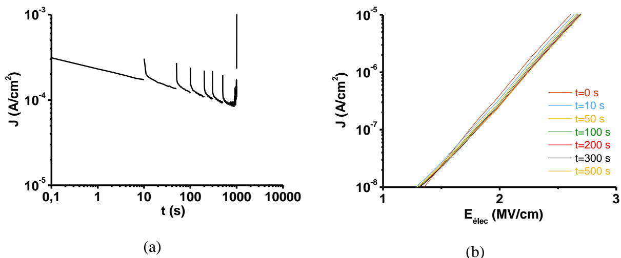
Figure V-29 : Mesure du courant au cours d'un vieillissement à 22 V (correspondant à un champ électrique de 3,33 MV/cm) et 125°C (a) et courbes J(E_{\text{élec}}) obtenues à différents temps t du vieillissement (b) ( s=70 nm).
