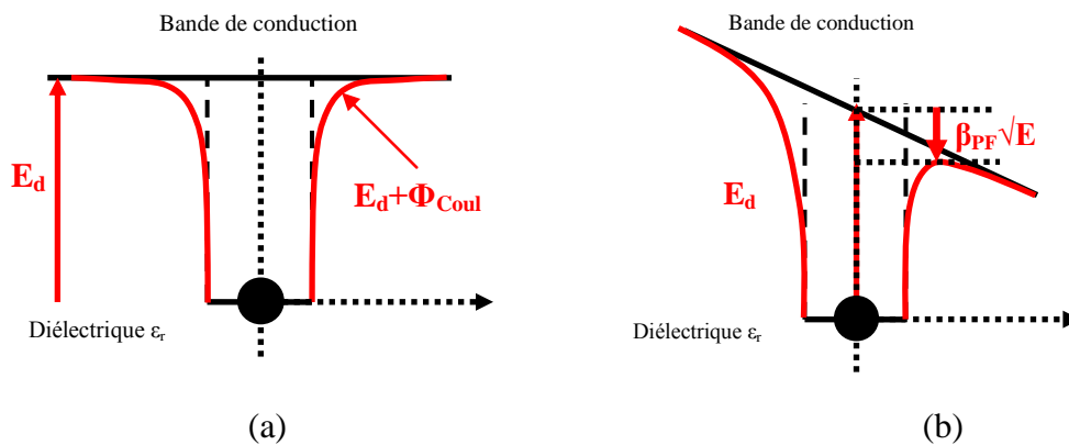
Figure II-16 : Effet de l'interaction Coulombienne entre l'électron et le piège sur le potentiel du piège : (a) en l'absence de champ, (b) en présence de champ.
