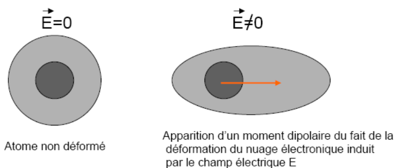
Figure II-1 : Polarisation électronique.
