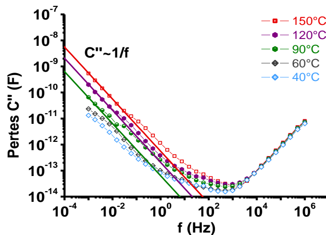
Figure IV-20 : Modélisation de l'augmentation des pertes diélectriques en 1/f ( s=140 nm).
