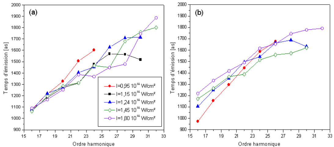
FIG. 6.16: Temps d'émission mesurés (a) dans l'azote et (b) dans l'argon pour différents éclairagements de génération (cercles rouges : I=0,95 \cdot 10^{14} \text{ W/cm}^2 , carrés noirs : I=1,15 \cdot 10^{14} \text{ W/cm}^2 , triangles bleus : I=1,24 \cdot 10^{14} \text{ W/cm}^2 , losanges verts : I=1,45 \cdot 10^{14} \text{ W/cm}^2 , hexagones violets : I=1,8 \cdot 10^{14} \text{ W/cm}^2 ).
