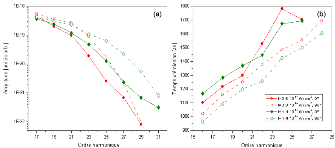
FIG. 6.20: (a) Spectre et (b) temps d'émission mesurés dans le CO_2 pour deux orientations (courbes pleines : 0^\circ , tirets : 90^\circ ) et deux éclairements de génération (cercles rouges : 0.8 \cdot 10^{14} \text{ W/cm}^2 et losanges verts : 1.4 \cdot 10^{14} \text{ W/cm}^2 ).
