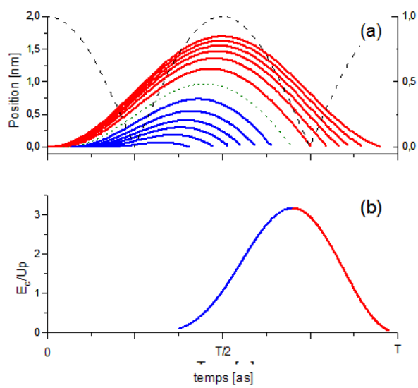
FIG. 4.2: (a) Trajectoires classiques des électrons en fonction du continuum. La courbe en pointillée représente l'évolution de la valeur absolue du champ infrarouge en fonction du temps. (b) Énergie cinétique des électrons (en unité de U_p ) en fonction de l'instant de recombinaison. Dans les deux cas, les courbes bleues (noires) représentent les trajectoires courtes, les courbes rouges (grises) les trajectoires longues. Les calculs ont été effectués pour un éclairement de 1 \cdot 10^{14} \text{ W/cm}^2 dans l'argon.
