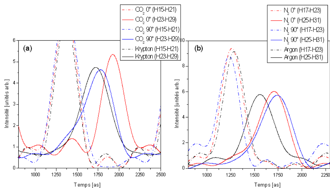
FIG. 6.11: Profil temporel de l'émission harmonique dans CO_2 (a) et N_2 (b).
