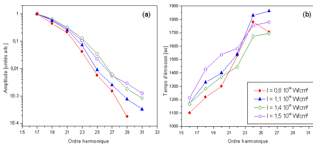
FIG. 6.18: Spectres (a) et temps d'émission (b) mesurés dans CO_2 pour différents éclairagements de génération (cercles rouges : I = 0,8 \cdot 10^{14} \text{ W/cm}^2 , triangles bleus : I = 1,1 \cdot 10^{14} \text{ W/cm}^2 , losanges verts : I = 1,4 \cdot 10^{14} \text{ W/cm}^2 , hexagones violets : I = 1,5 \cdot 10^{14} \text{ W/cm}^2 ).
