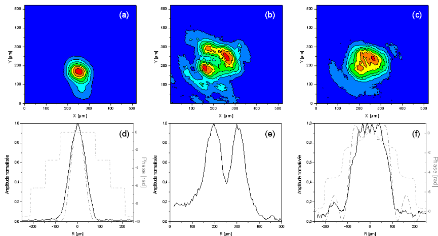
FIG. 2.5: Effet des lames de phase de taille intermédiaire sur le faisceau du laser LUCA. En (a), (b) et (c) les distributions spatiales au foyer ( z=0 ) du champ laser dans trois configurations (déphasage \Phi = 0, \pi radians et 0.8\pi radians). En (d), (e) et (f) les coupes de chacun des profils. La ligne pointillée grise correspond au profil d'intensité calculé, la ligne pointillée claire à la phase calculée.
