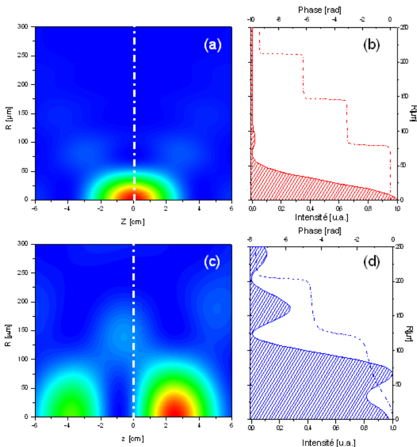
FIG. 1.18: Comparaison de la propagation d'un faisceau mis en forme (c) ou non (a). (a) et (c) : Intensité infrarouge dans le plan (x;z) . (b) et (d) : Profil radial d'intensité (ligne continue) et phase (tirets) en z=0 .
