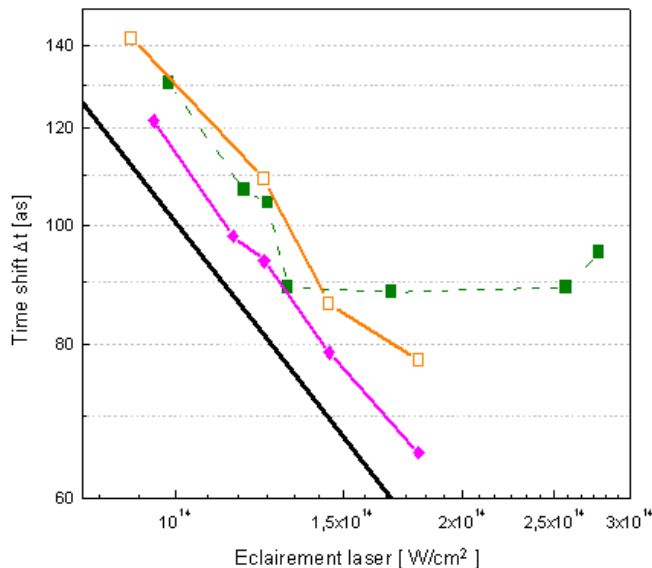
FIG. 6.17: Dérive de fréquence attoseconde \Delta t_e en fonction de l'éclairement de génération. Valeurs théoriques (ligne noire), mesures dans l'argon (carrés) extraites de Mairesse et al. (2003). Mesures dans l'argon (carrés creux) et l'azote (losanges) lors de la présente campagne expérimentale.
