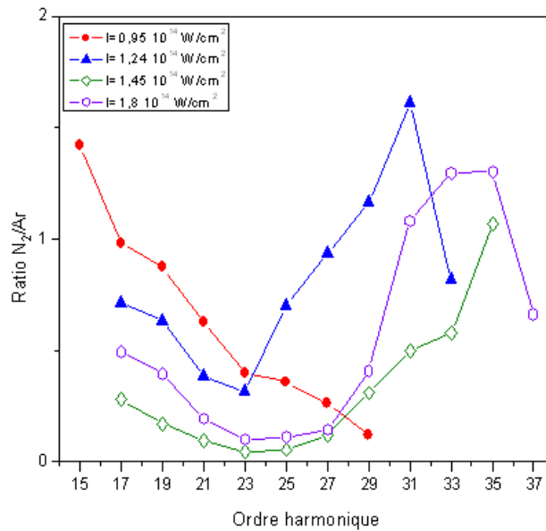
FIG. 6.15: Spectres générés dans l'azote à différents éclairagements de génération normalisés par les spectres générés dans l'argon aux mêmes éclairagements. (cercles rouges : I=0,95 \cdot 10^{14} \text{ W/cm}^2 , triangles bleus : I=1,24 \cdot 10^{14} \text{ W/cm}^2 , losanges verts : I=1,45 \cdot 10^{14} \text{ W/cm}^2 , hexagones violets : I=1,8 \cdot 10^{14} \text{ W/cm}^2 ).
