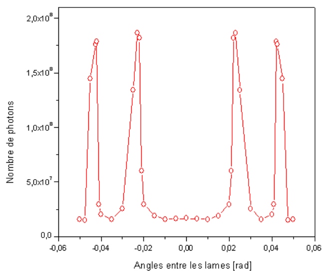
FIG. 1.22: Evolution du signal harmonique (H19) généré dans l'argon en fonction de l'angle \theta_1 entre les lames de phase.
