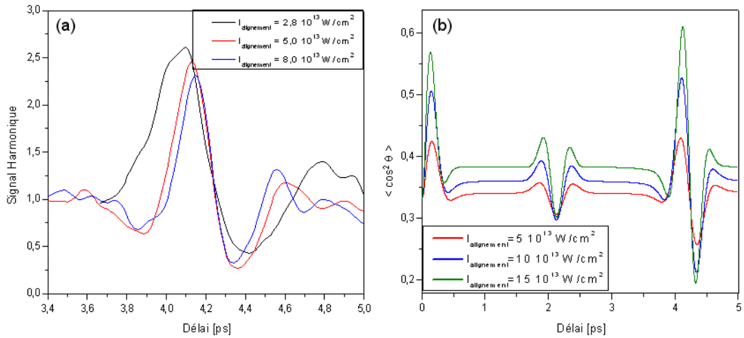
FIG. 5.3: Effet de l'éclairement du faisceau d'alignement sur l'évolution du signal harmonique généré par N_2 . (a) Signal mesuré (raie satellite 22) pour trois éclairements (noir : 2.8 \cdot 10^{13} \text{ W/cm}^2 , rouge : 5 \cdot 10^{13} \text{ W/cm}^2 , bleu : 8 \cdot 10^{13} \text{ W/cm}^2 ). (b) Évolution de \langle \cos^2 \theta \rangle pour trois éclairements (rouge : 5 \cdot 10^{13} \text{ W/cm}^2 , bleu : 10 \cdot 10^{13} \text{ W/cm}^2 , vert : 15 \cdot 10^{13} \text{ W/cm}^2 ).
