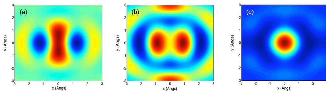
FIG. 7.3: Influence de la phase spectrale pour la reconstruction tomographique. (a), (b) et (c) : reconstructions de l'orbitale HOMO de l'azote (voir texte pour les paramètres).
