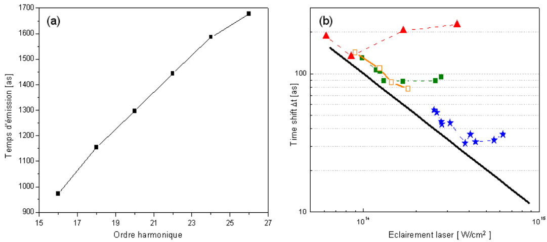
FIG. 5.11: (a) Temps d'émission mesurés dans l'argon pour un éclairement de 0.9 \cdot 10^{14} W/cm^2 . (b) Dérive de fréquence attoseconde \Delta t_e en fonction de l'éclairement laser. Valeurs théoriques (ligne noire), mesures dans le xénon (triangles), l'argon (carrés) et le néon (étoiles) extraites de Mairesse et al. (2003) . Mesures dans l'argon (carrés creux) lors de la présente campagne expérimentale.
