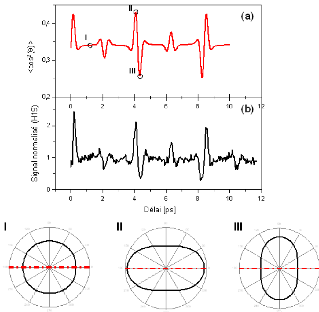
FIG. 5.1: (a) Évolution de \langle \cos^2 \theta \rangle calculé. (b) Évolution expérimentale du signal harmonique (H19) généré dans l'azote en fonction du délai entre les faisceaux d'alignement et de génération. (I), (II) et (III) : distributions angulaires pour différents délais (respectivement 1ps, 4.1 ps et 4.3 ps). L'axe pointillé correspond à la direction de polarisation du laser d'alignement.
