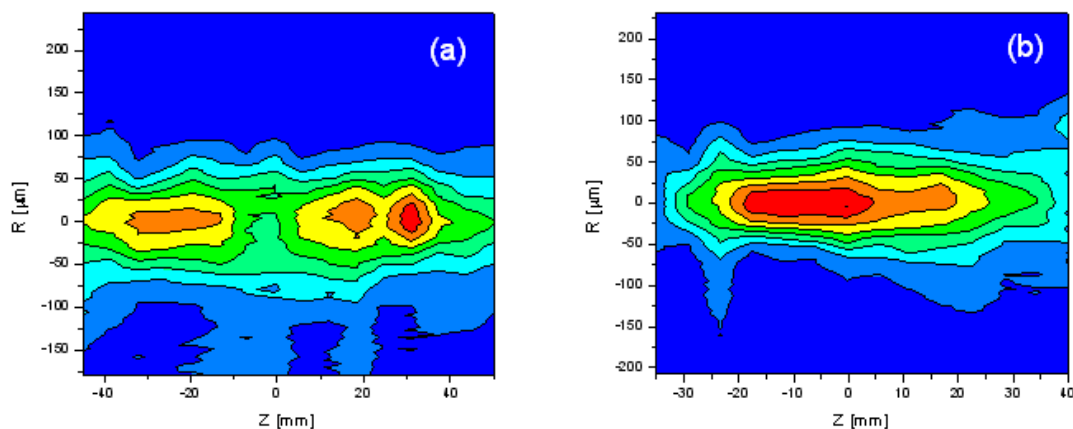
FIG. 2.7: Mesure du profil infrarouge autour du foyer dans le cas des faisceaux mis en forme (a) et gaussien (b). Le laser se propage de la gauche vers la droite suivant l'axe Oz.
