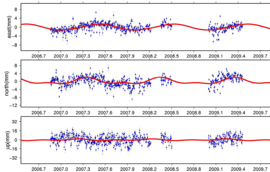
CRLM_GPS
