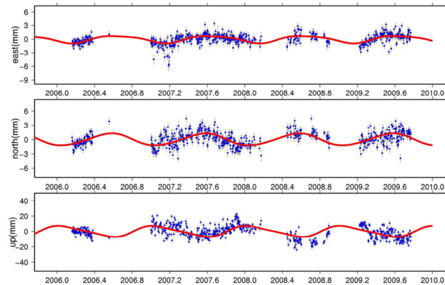
VEAR_GPS
