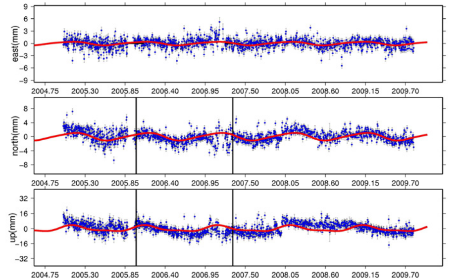
ENAV_GPS
