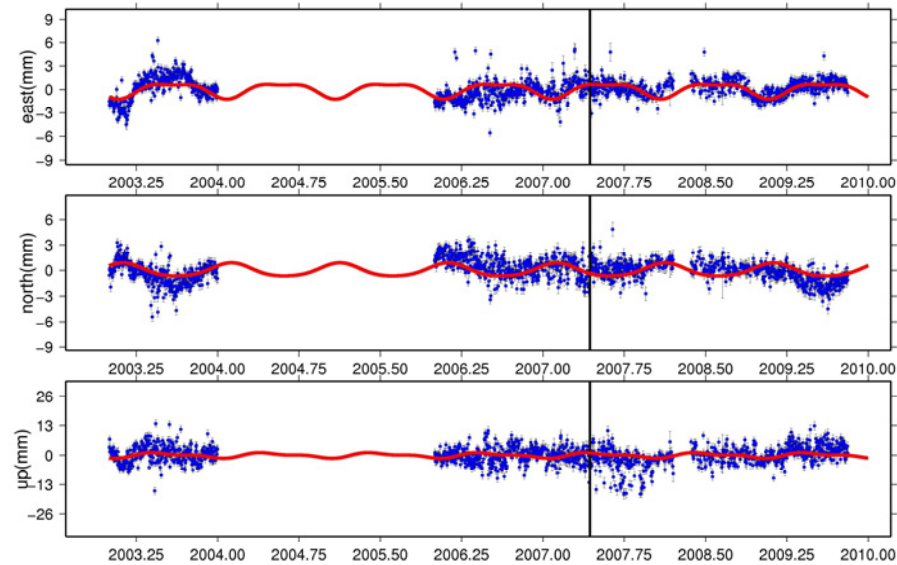
OROS_GPS
