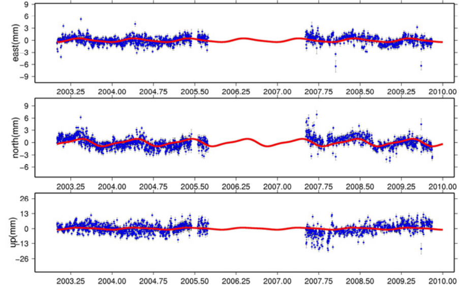
OSJE_GPS
