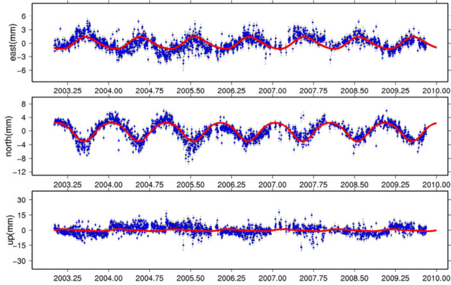
PADO_GPS
