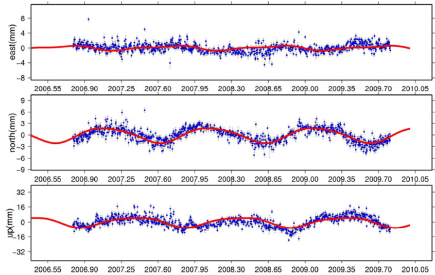
PARM_GPS
