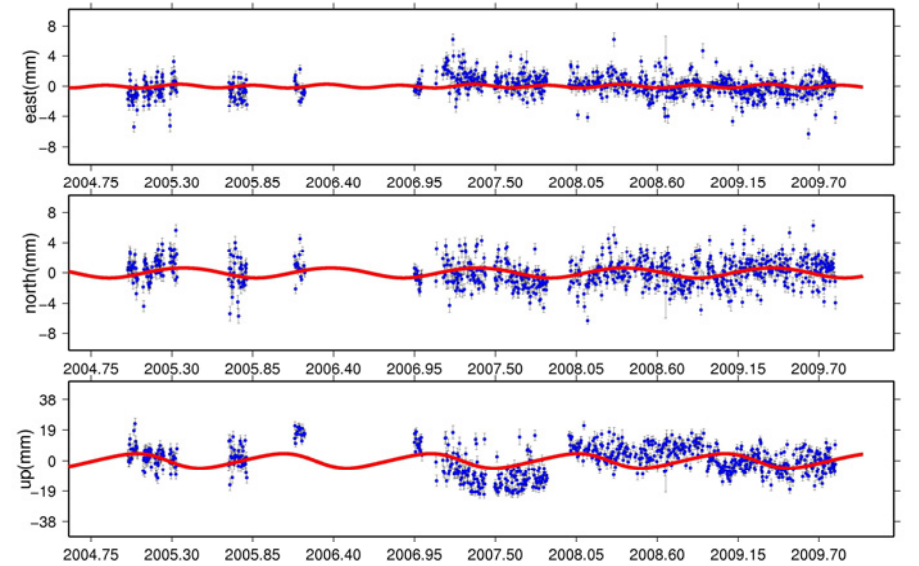
PACA_GPS
