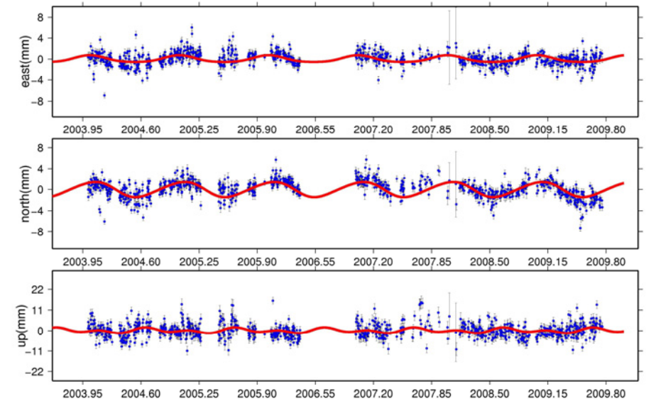
NOVA_GPS
