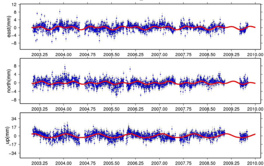
LAMP_GPS
