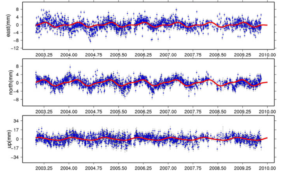
NOT1_GPS
