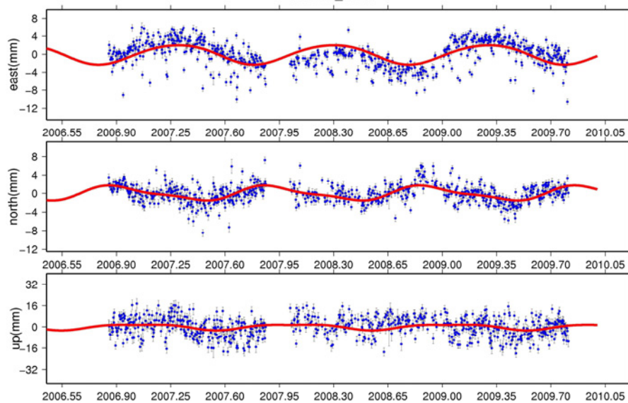
LATT_GPS
