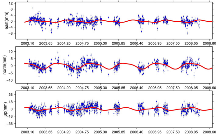
EYPA_GPS
