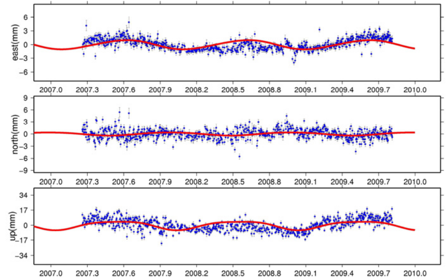
MOPS_GPS
