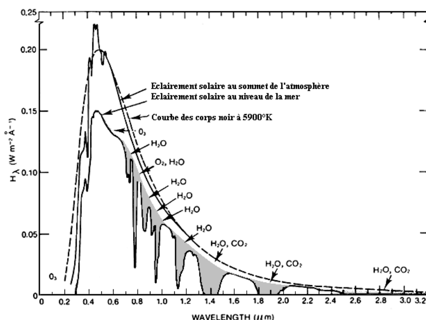
Figure II-3: Courbes d'éclairement solaire modifié par les absorptions atmosphériques dans le visible et le proche infrarouge. Les zones grisées correspondent aux domaines de longueurs d'ondes où se produit une absorption du rayonnement par l'atmosphère et où aucune information spectrale n'est disponible lors de mesures in situ ou par télédétection.
