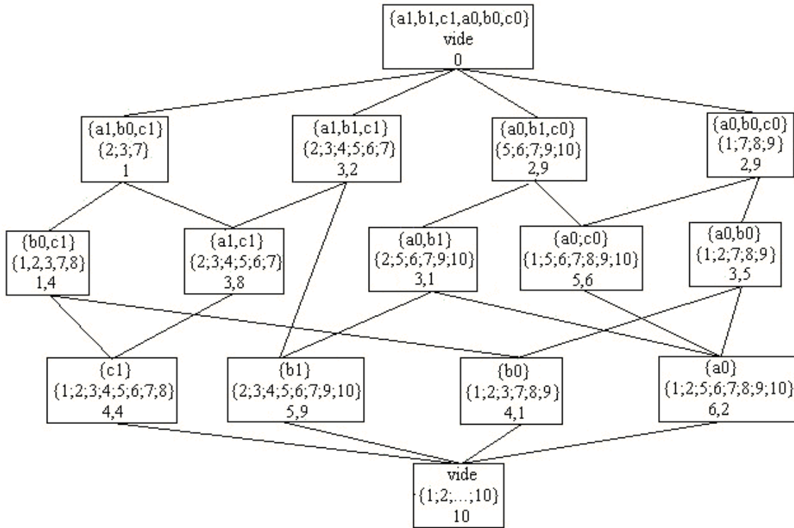
FIG. A.1 – Le treillis flou des motifs associés aux 3 propriétés du tableau 9.3, et à leurs négations.
