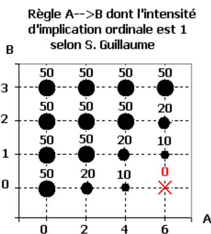
FIG. 9.8 – Une règle d'implication ordinale
