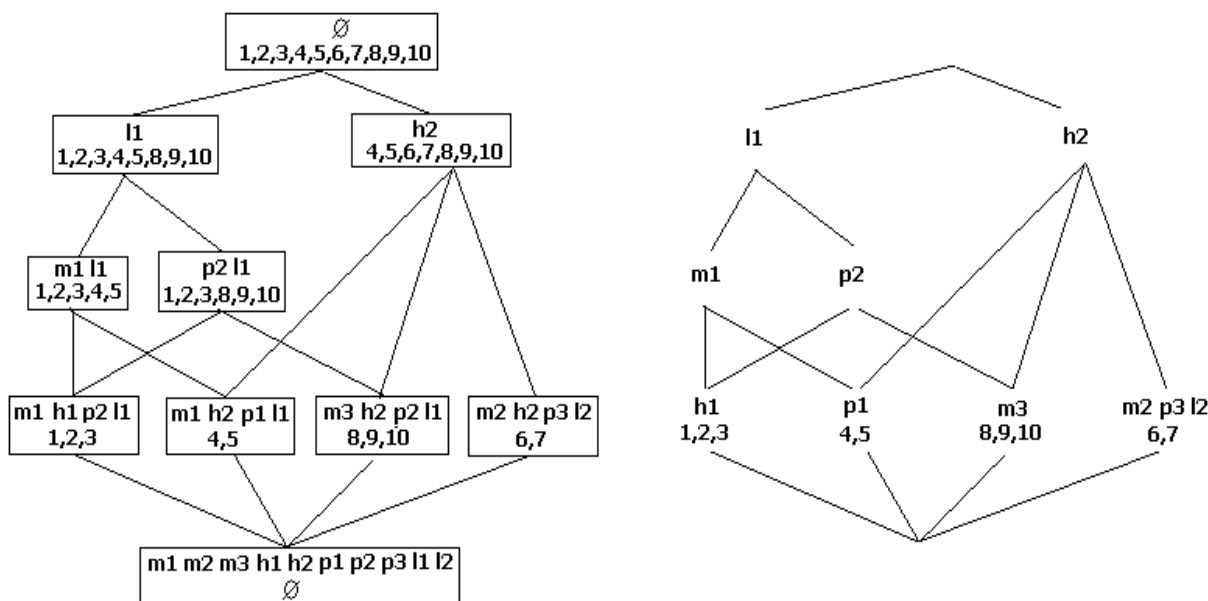
FIG. 4.7 – Diagramme de Hasse et diagramme simplifié du treillis des concepts du tableau T'
