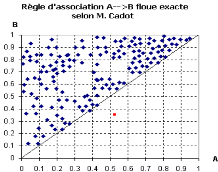
FIG. 9.9 – Une règle d'association floue A \rightarrow B de confiance 1
