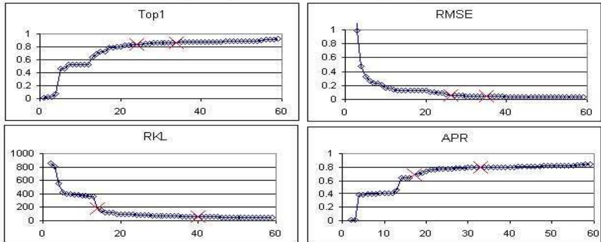
KDDCup 2004 - Résultats pour les données "bio" des 59 participants Les deux croix rouges représentent les résultats des deux techniques développées par Martine Cadot*, Joseph di Martino*, Laurent Pierron** * UHP-LORIA, Nancy, France ** LORIA, Nancy, France
