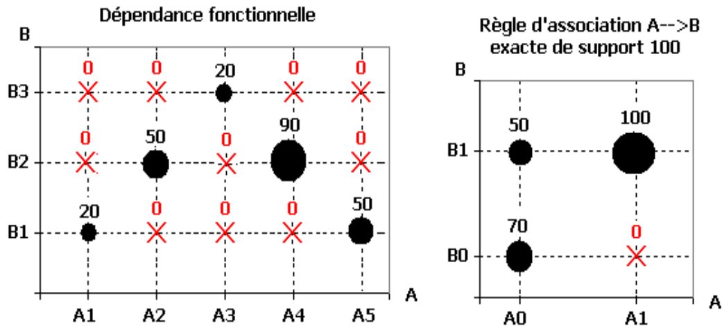
FIG. 4.8 – Une dépendance fonctionnelle et une règle d'association exacte
