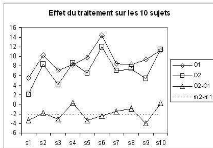
FIG. 2.3 – Les différences de mesure pour chacun des 10 sujets
