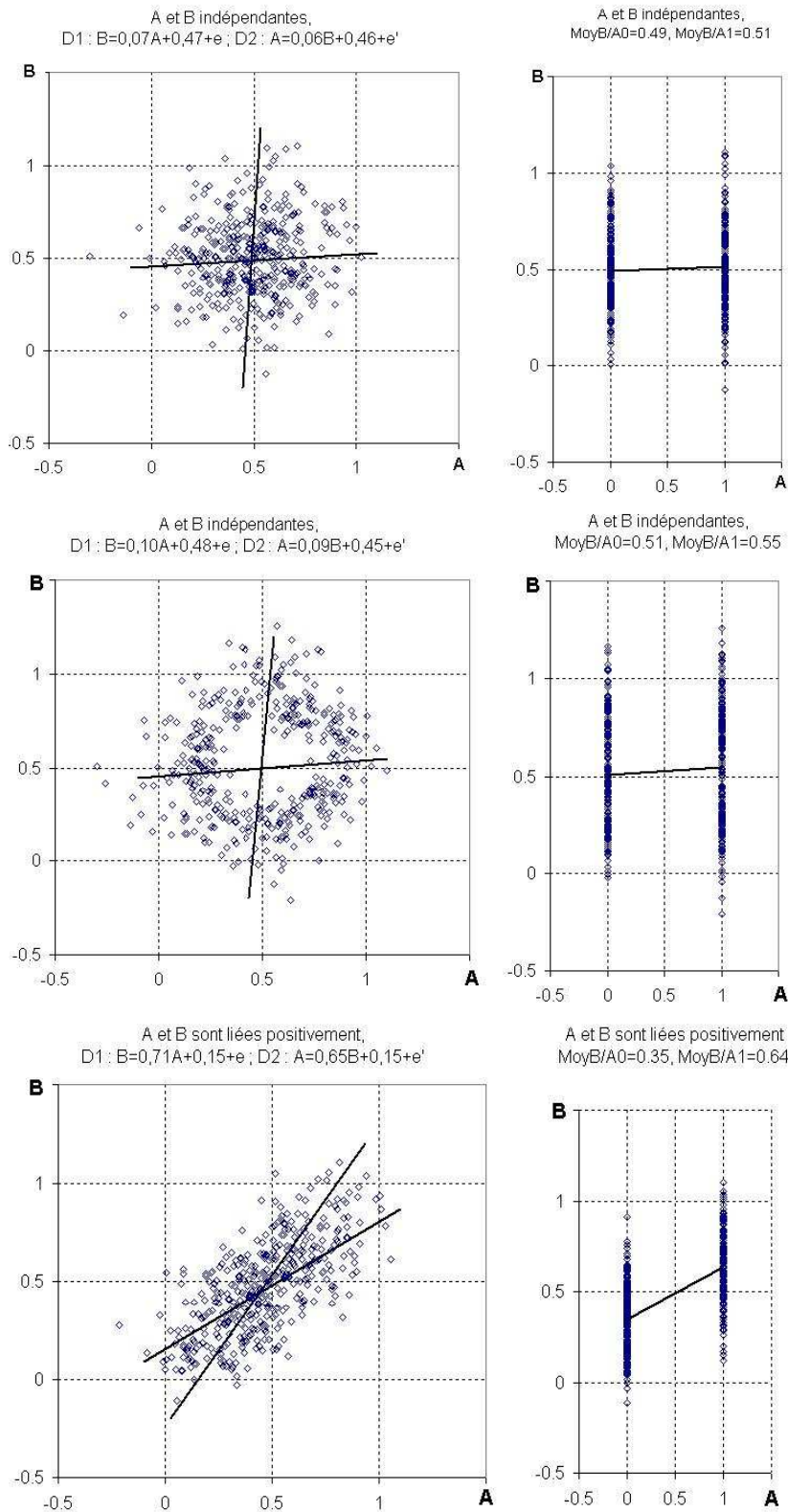
FIG. 7.1 – En haut, l'indépendance "vraie", en dessous, l'indépendance "fausse", en bas une "vraie" liaison positive.
