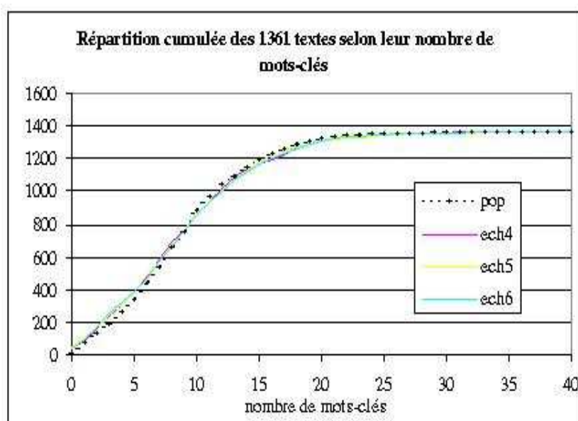
FIG. 5.5 – Fréquences cumulées de la répartition des textes selon leur nombre de mots-clés pour 3 simulations de type 2.
