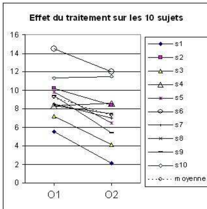
FIG. 2.2 – Les évolutions de chacun des 10 sujets
