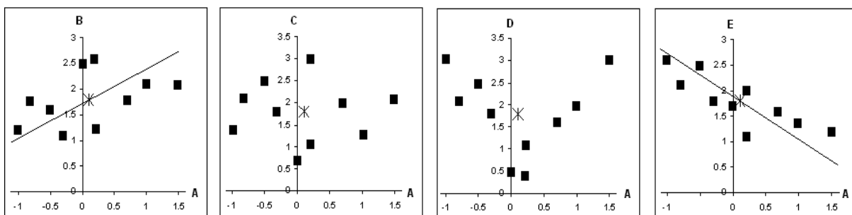
FIG. 2.17 – Nuages de points correspondants au tableau de la figure 2.16
