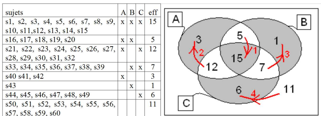
FIG. 10.3 – Répartition de 60 sujets selon 3 propriétés.
