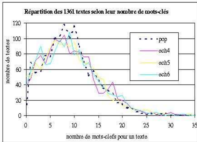
FIG. 5.4 – histogramme de la répartition des textes selon leur nombre de mots-clés pour 3 simulations de type 2.
