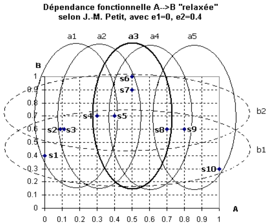
FIG. 9.6 – Les 10 sujets de la relation R du tableau U dans le plan AxB et leur répartition dans les classes selon A et B avec e_1 = 0 et e_2 = 0,4
