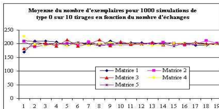
FIG. 6.3 – Le nombre moyen d'exemplaires de la matrice du tableau 1 obtenus par des simulations de type 0.
