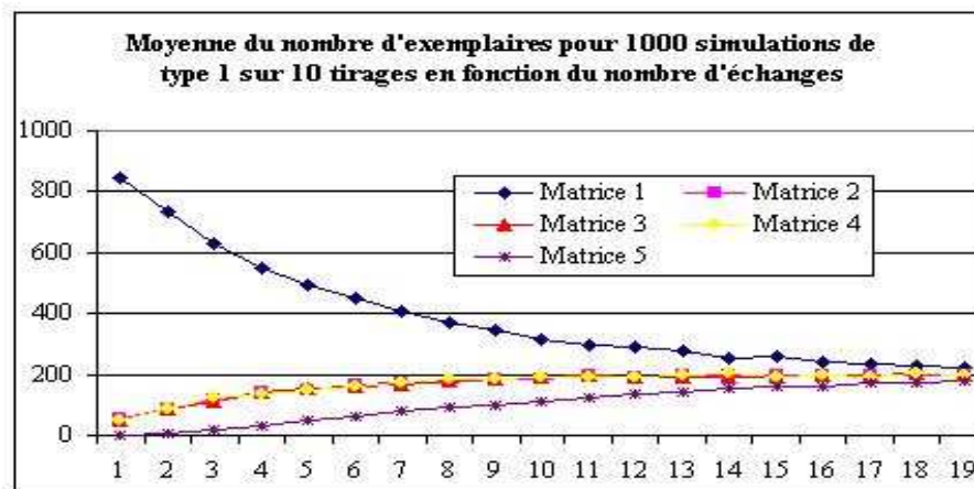
FIG. 6.1 – Le nombre moyen d'exemplaires de la matrice du tableau 1 obtenus par des simulations de type 1.
