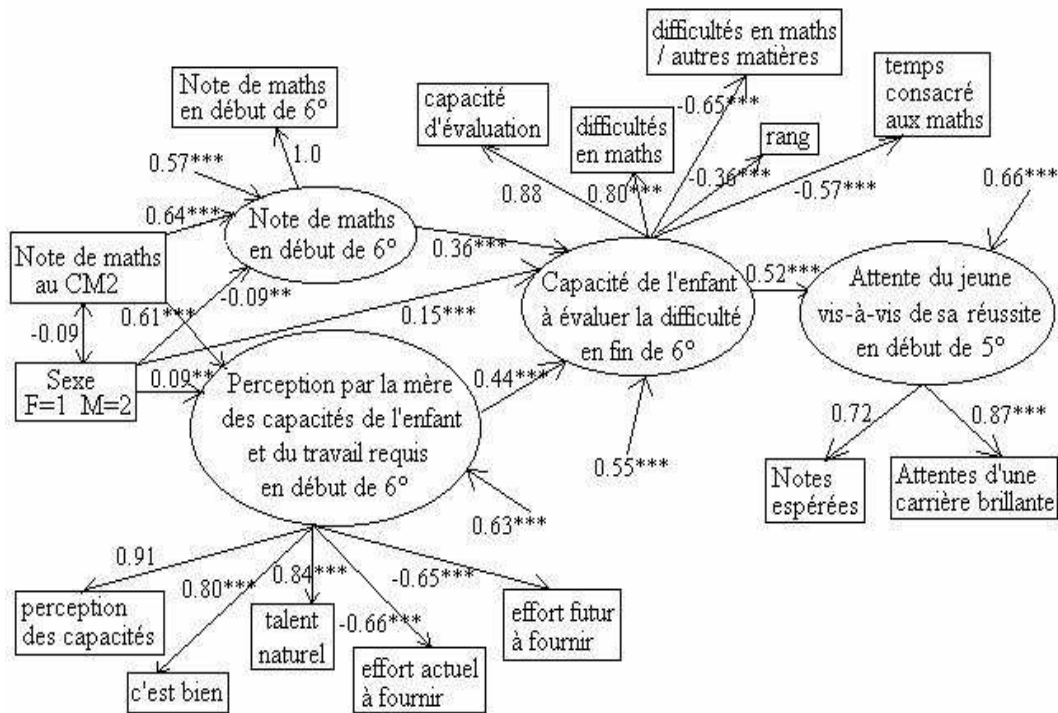
FIG. 2.13 – Un modèle explicatif scolaire
