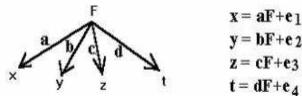
FIG. 2.14 – Une variable latente F obtenue à partir de quatre variables manifestes, toutes ces variables ainsi que les erreurs constituent des vecteurs
