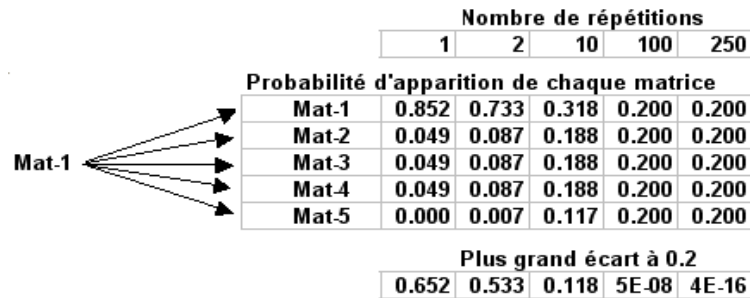
FIG. 6.2 – Les probabilités associées aux différentes matrices pour des simulations de type 1.
