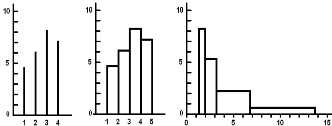
FIG. 1.2 – Diagramme à bâtons à gauche, histogrammes au milieu et à droite
