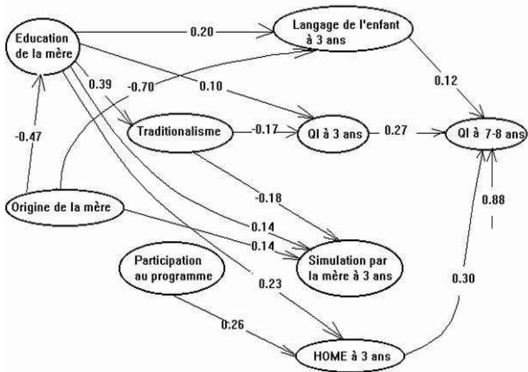
FIG. 2.12 – Un modèle explicatif du QI bâti sur un questionnaire.
