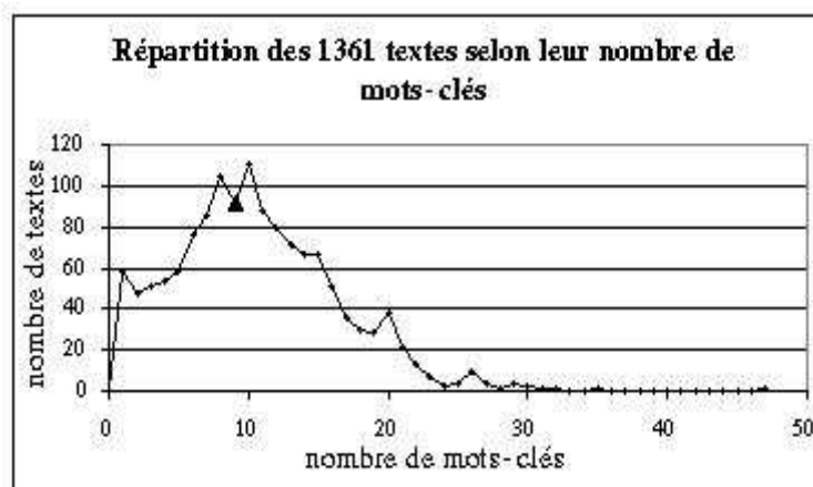
FIG. 5.1 – Les 1 361 textes répartis selon leur nombre de mots-clés.
