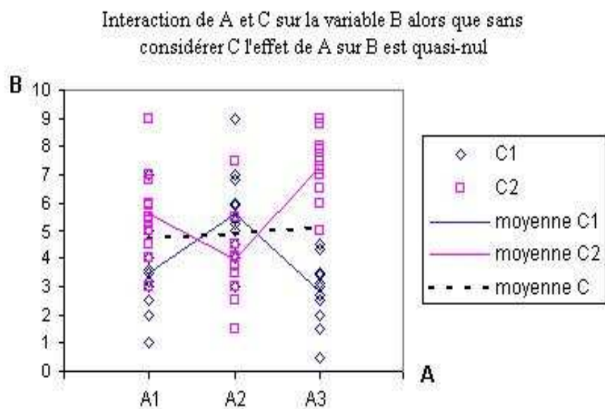
FIG. 2.20 – Les moyennes de B selon A sont 3,48, 5,61 et 2,82 pour C1, 5,61, 3,98 et 7,32 pour C2 et 4,64, 4,87 et 5,07 pour C1 et C2.
