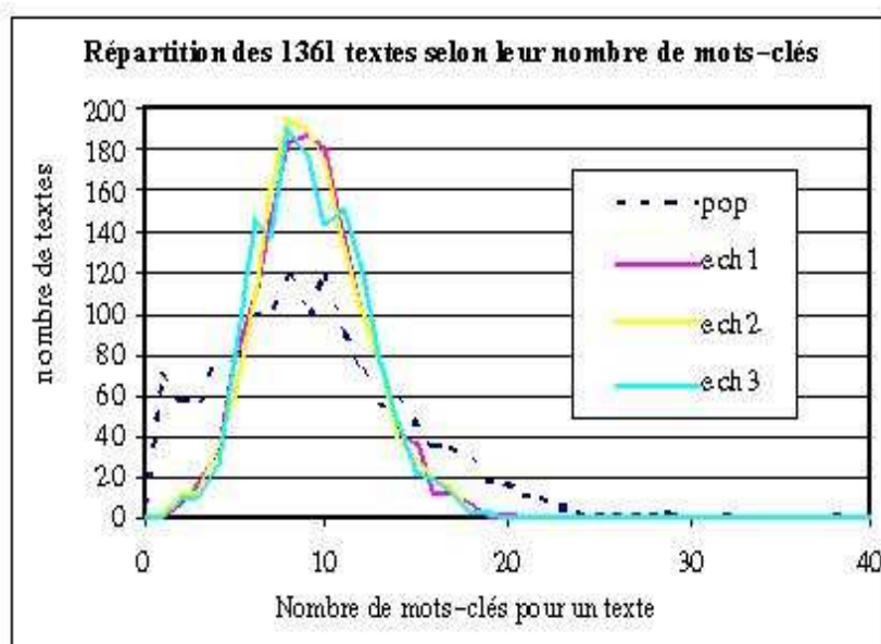
FIG. 5.3 – Histogramme de répartition des textes selon leur nombre de mots-clés pour 3 simulations de type 1.
