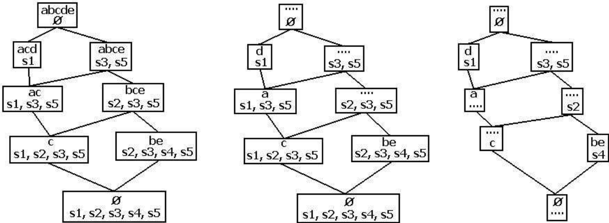
FIG. 4.1 – Treillis des concepts de l'exemple du tableau 4.1
