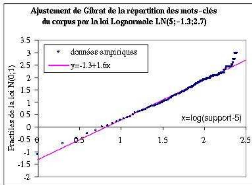
FIG. 5.6 – La loi Lognormale LN(5;-1,3;2,7) pourrait être une bonne approximation de la distribution des mots-clés.
