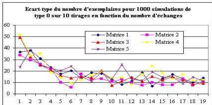
FIG. 6.4 – L'écart-type du nombre d'exemplaires de la matrice du tableau 6 obtenus par des simulations de type 0.
