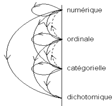
FIG. 1.3 – Les changements possibles entre types élémentaires de données
