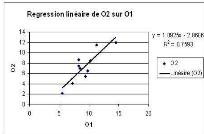
FIG. 2.6 – La droite de régression de O2 sur O1
