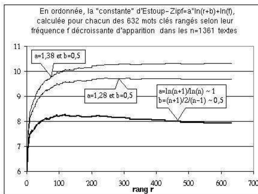
FIG. 5.7 – La répartition des mots-clés dans les textes ne suit pas exactement une loi d'Estoup-Zipf ( a=1 ), mais plutôt une loi "Zipf-like" ( 1,28 \leq a \leq 1,38 ).
