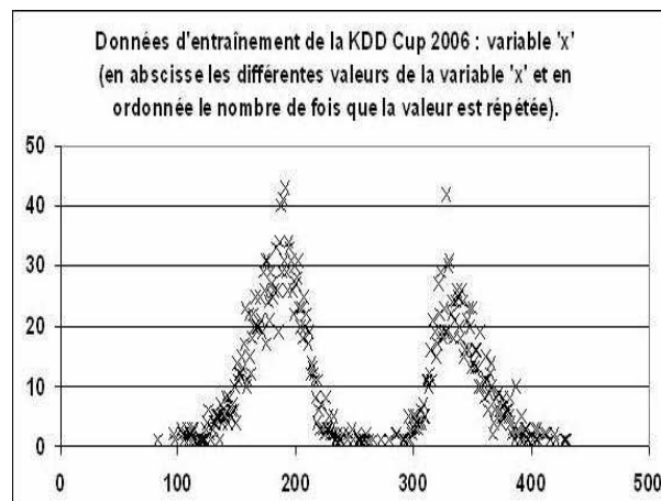
FIG. 1.6 – Répartition des valeurs de la variable "x" de la Kdd Cup 2006 pour les données d’entraînement
