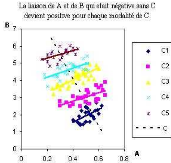
FIG. 2.19 – La corrélation entre A et B est de -0.41 pour l'ensemble, et elle varie de 0,58 à 0,83 à Ci fixé.
