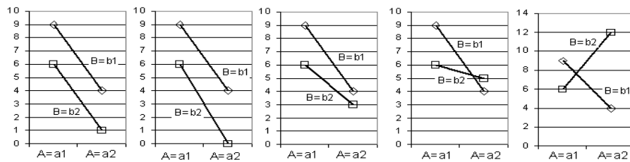
FIG. 2.15 – Interaction de B avec A , nulle à gauche puis en allant vers la droite augmentant l'effet de A , le diminuant, le faisant presque disparaître, le faisant changer de sens.
