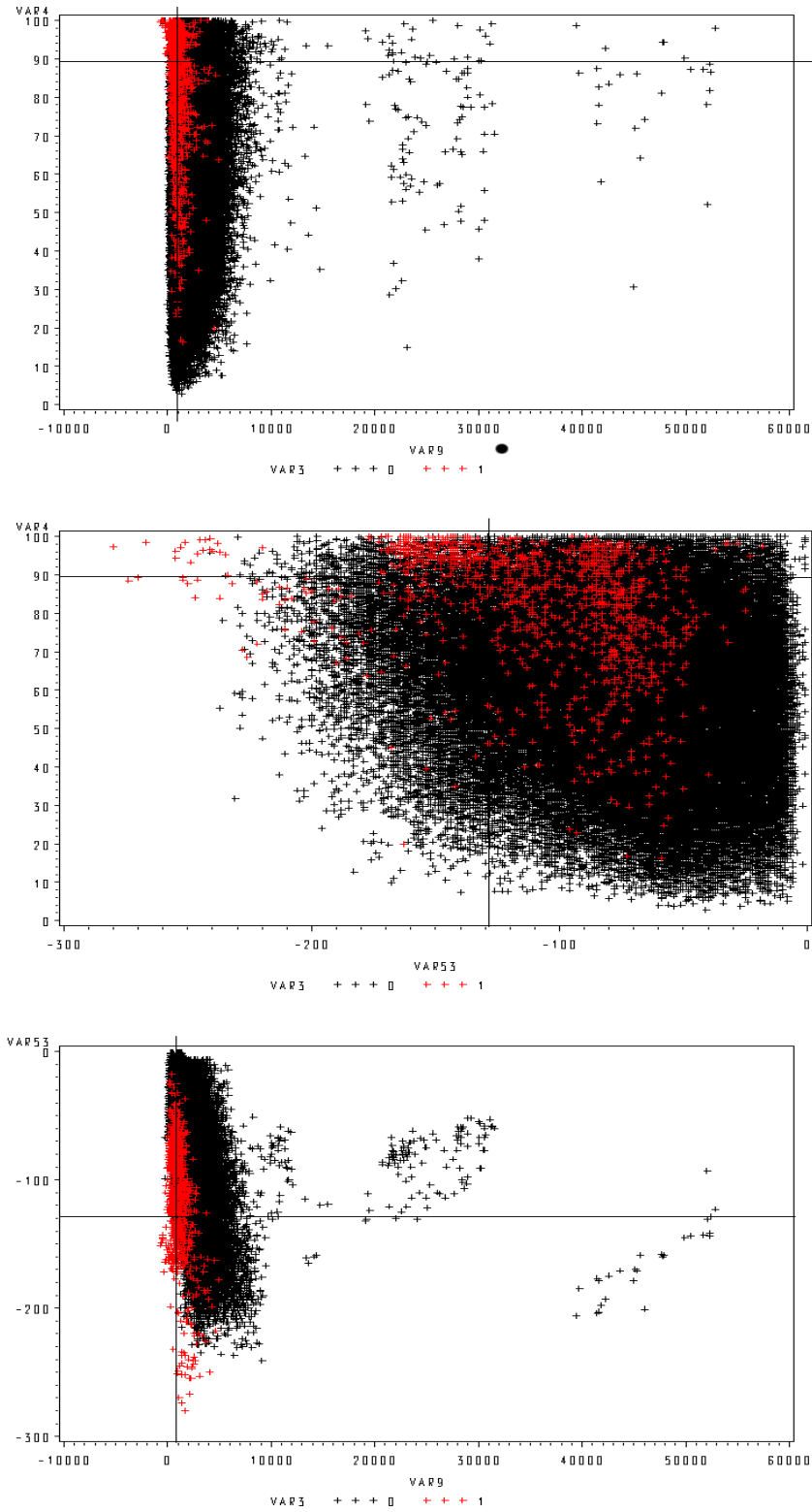
FIG. 10.1 – Les variables V4, V9 et V53.
