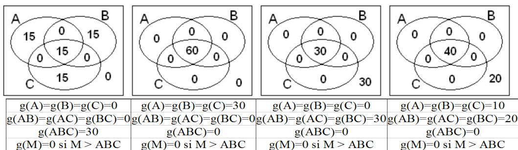
FIG. 10.4 – Valeurs remarquables du gain pour des cas particuliers
