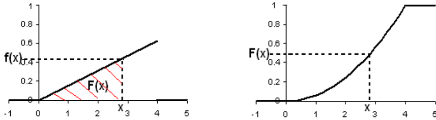
FIG. 3.2 – Les éléments caractéristiques de la loi de probabilité de X : f sa densité, F sa fonction de répartition
