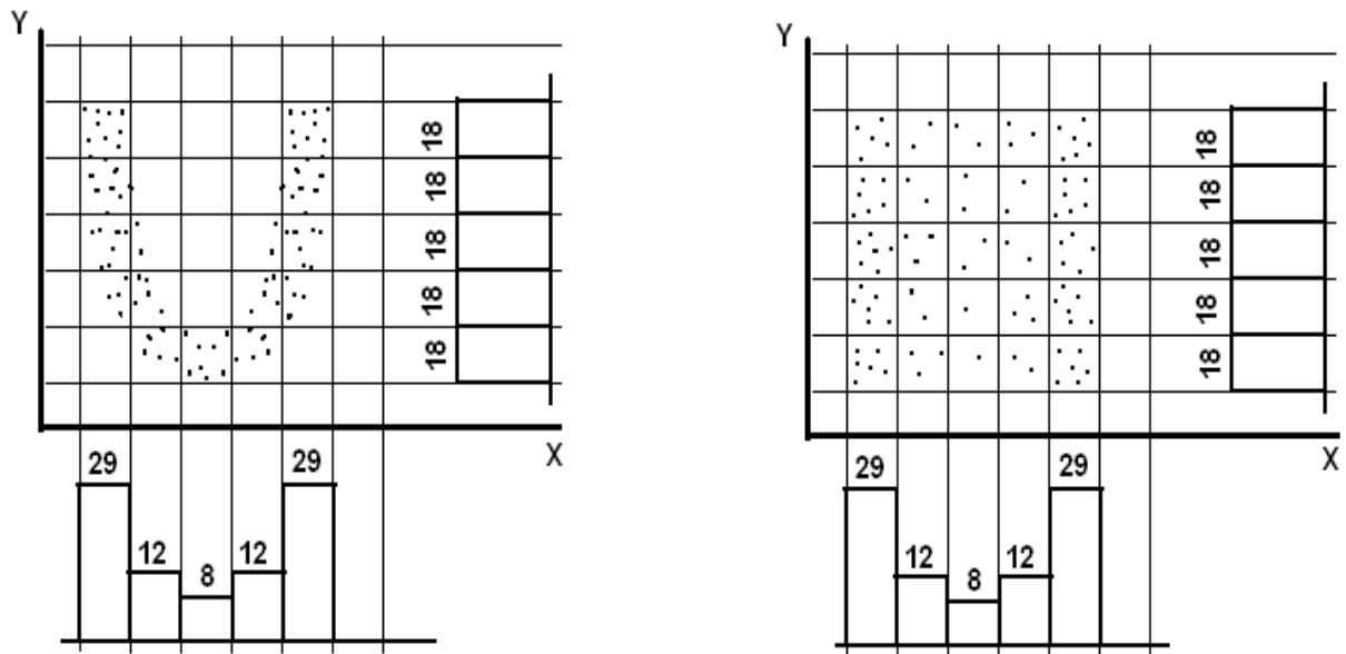
FIG. 2.18 – A gauche une liaison parabolique, à droite indépendance, à distributions marginales égales
