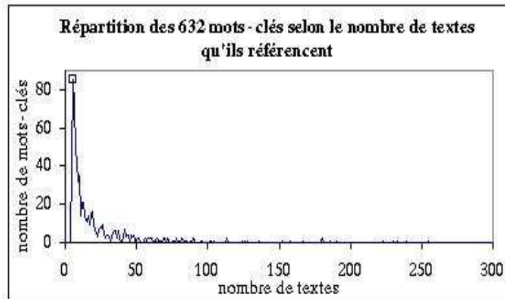
FIG. 5.2 – Les 632 mots-clés répartis selon le nombre de textes qu'ils référencent.
