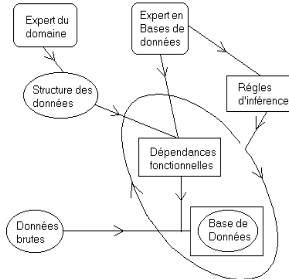
FIG. 4.5 – Production d'une base de données à l'aide de dépendances fonctionnelles
