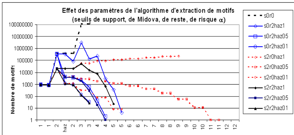
FIG. 10.9 – Comparaison des efficacités respectives de l'utilisation combinée de Midova et du test d'échanges en cascade avec la méthode classique de type A Priori, avec seuil de support
