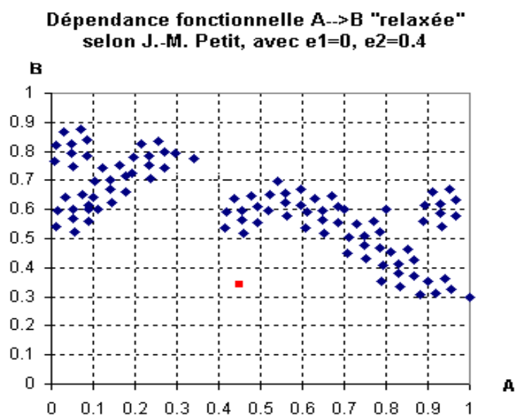
FIG. 9.7 – Une dépendance fonctionnelle A \rightarrow B avec \epsilon_1 = 0 et \epsilon_2 = 0,4
