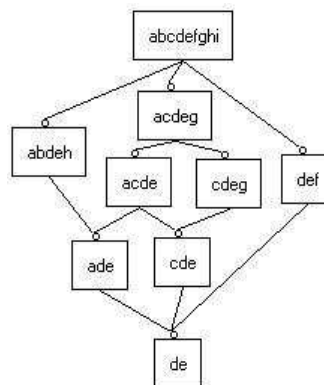
FIG. 9.5 – Le treillis des motifs fermés du tableau 5 avec \gamma=2 et \delta=3 .
