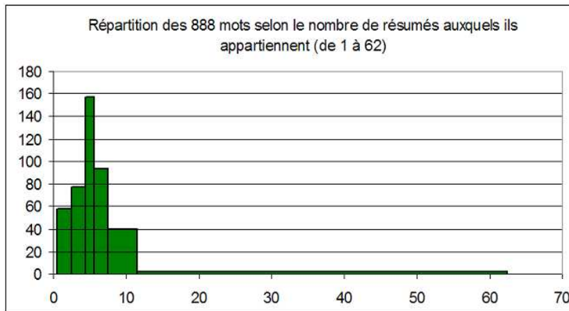
FIG. 10.6 – Répartition des mots et des résumés (2/2)
