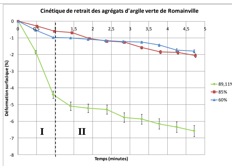
Figure 110: Evolution de la déformation surfacique en fonction du temps. Courbe de retrait de l'argile verte de Romainville sur agrégats de 50 \mu\text{m} . Courbes « cumulatives » en haut ; courbes « individuelles » en bas.
