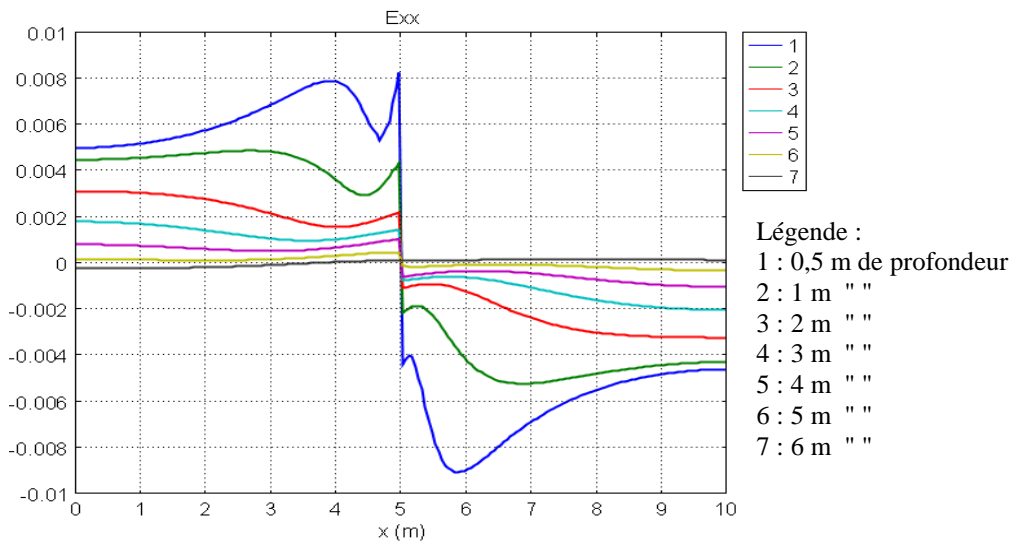
Figure 164 : Distribution de la déformation horizontale à différentes profondeur du sol (cas du gonflement).
