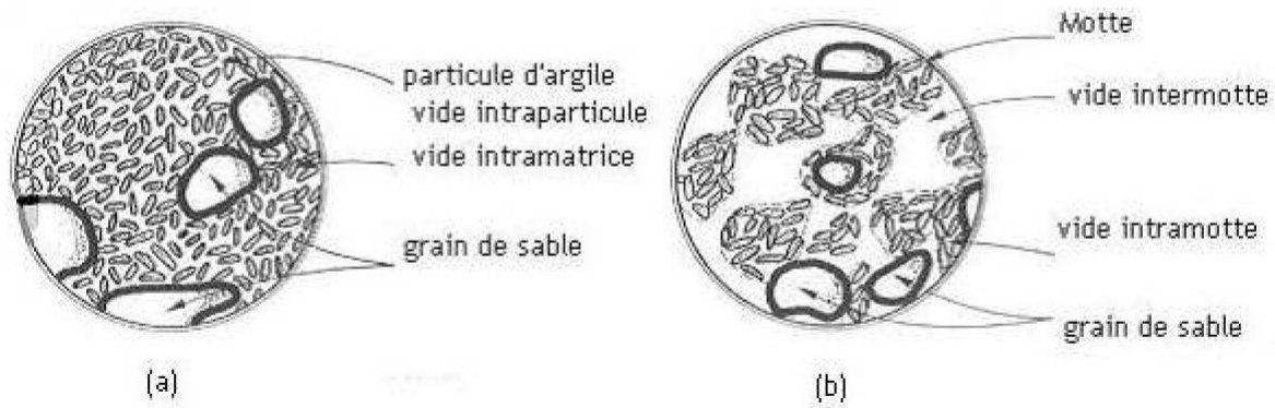
Figure 6: Texture des sols gonflants (d'après Gens & Alonso, 1992)
