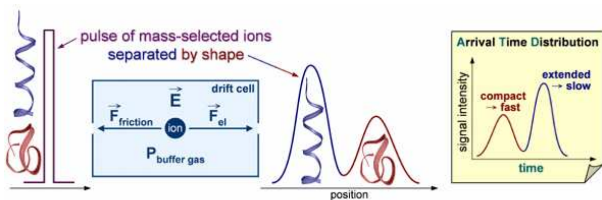
Figure I-1 : Principe de la mesure de mobilité ionique
