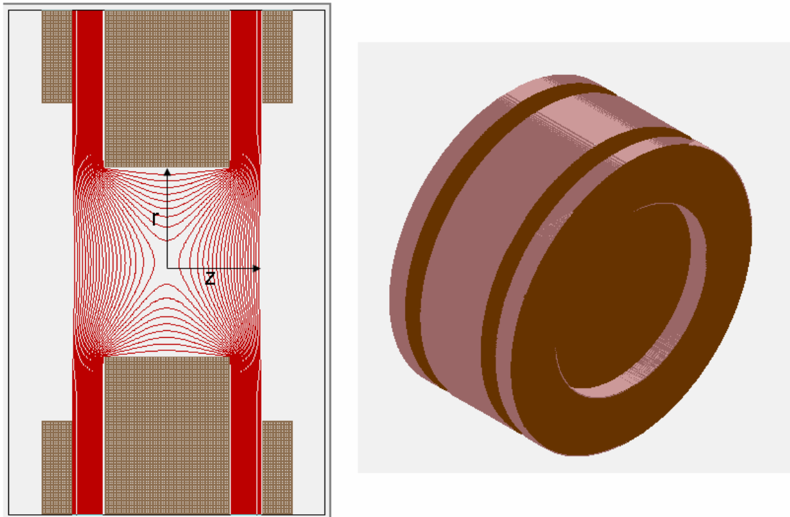
Figure III-8 : Piège ionique cylindrique. Vue avec les lignes d'isopotential (gauche), vue 3D (à droite). Les images proviennent du logiciel Simion.
