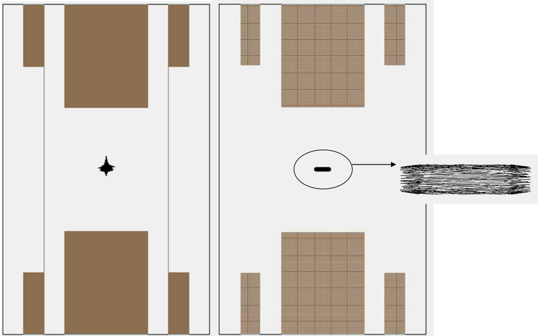
Figure III-11 : Trajectoire d'un ion dans le piège ionique cylindrique. A gauche pour une pression de 10 Torr et a droite dans le vide.
