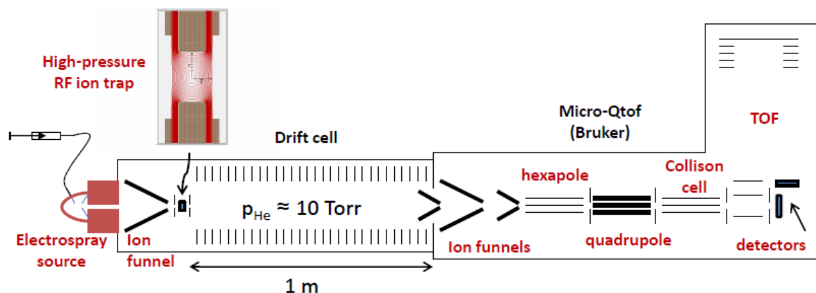
Figure I-1 : Expérience MS+ : Schéma des éléments constituant le couplage IMS/MS.
