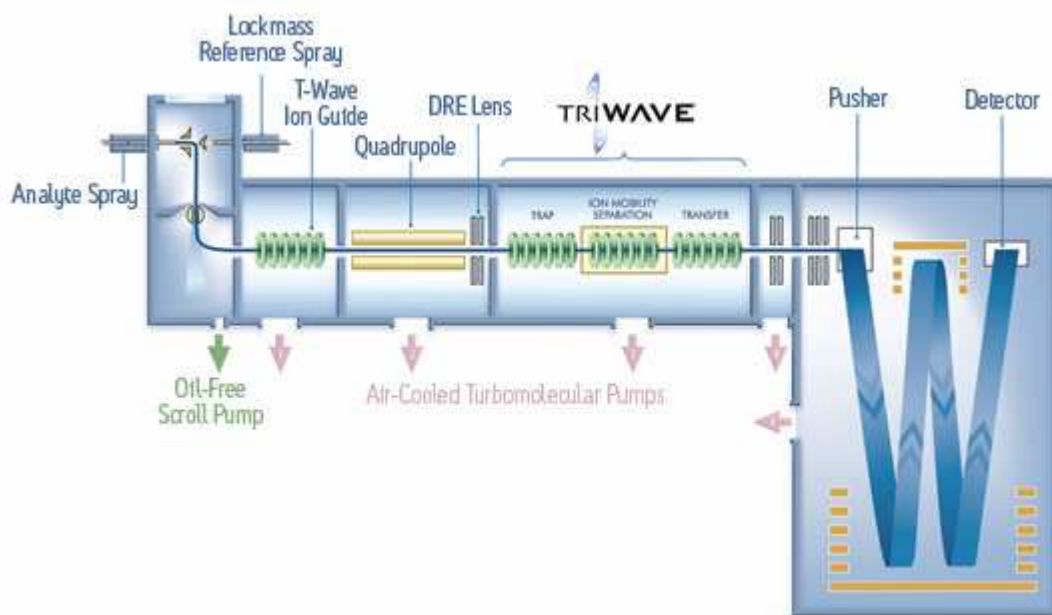
Figure III-11 : Schéma du dispositif Synapt
