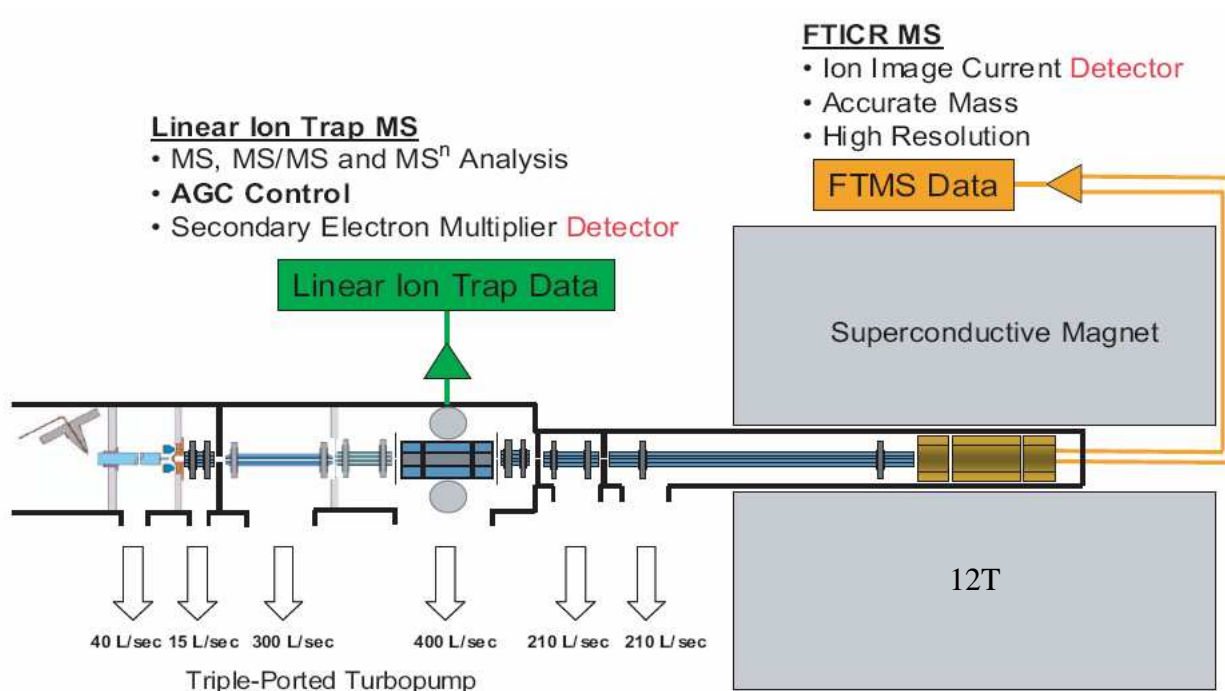
Figure III-1 : Schéma de l'expérience LTQ-FTICR.
