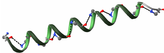
Figure I-2 : Structure du monomère M2TMP déterminée par RMN liquide et solide (PDB 11 : 1NY).
