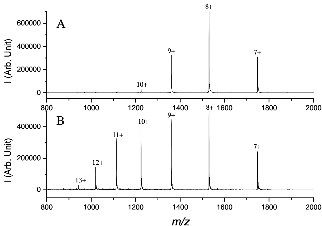
Figure II-2 : Spectre de masse du Cytochrome C de cœur de bœuf en fonction du solvant. A) 100% eau. B) 50/50 eau/methanol.
