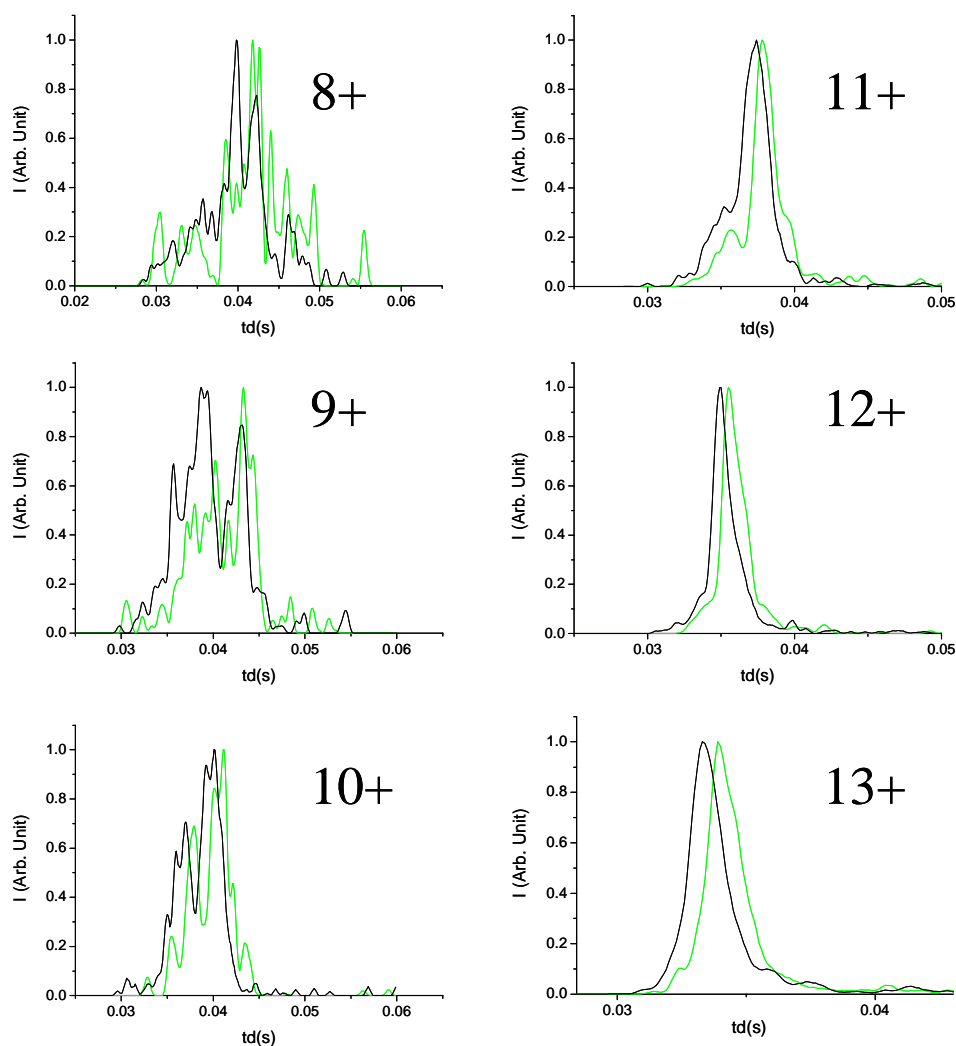
Figure II-5 : Comparaison des profils de temps d'arrivé avec (vert) et sans base (noir) pour le cytochrome C.
