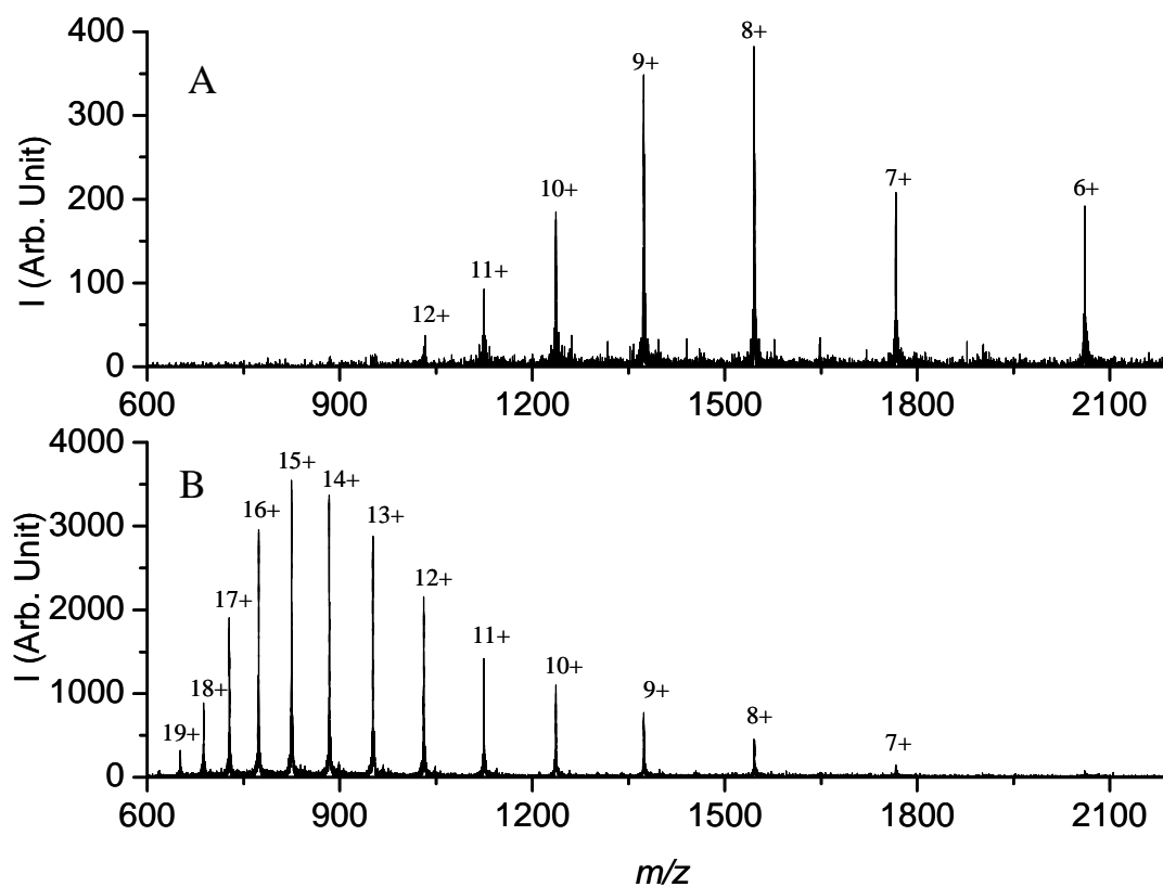
Figure II-4 : Comparaison des spectres de masse pour le cytochrome C sans base (B) et avec base (A).
