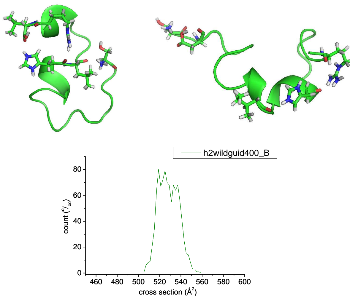
Figure V-3 : Profil de section efficace de diffusion calculé pour une contrainte à 400 \text{ \AA}^2 et structures représentatives des simulations, 518 \text{ \AA}^2 pour la structure de gauche et 540 \text{ \AA}^2 pour la structure de droite.
