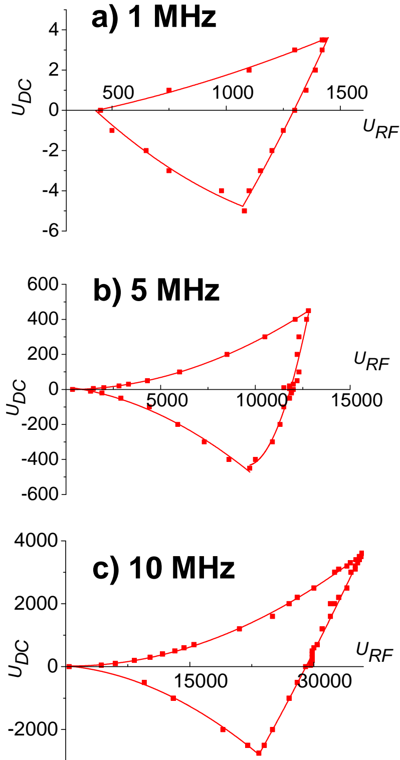
Figure III-12 : Diagramme de stabilité pour différentes fréquences
