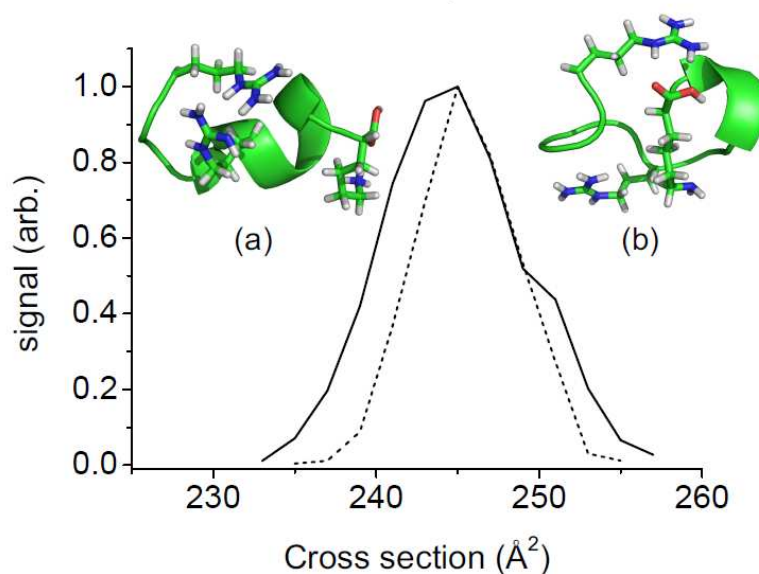
Figure III-5 : Comparaison des structures et des sections efficaces de diffusion pour le peptide [RA_4RA_4K+2H]^{2+} avec les charges en position 1 et 11 (ligne noire) et 1 et 6 (pointillés noirs).
