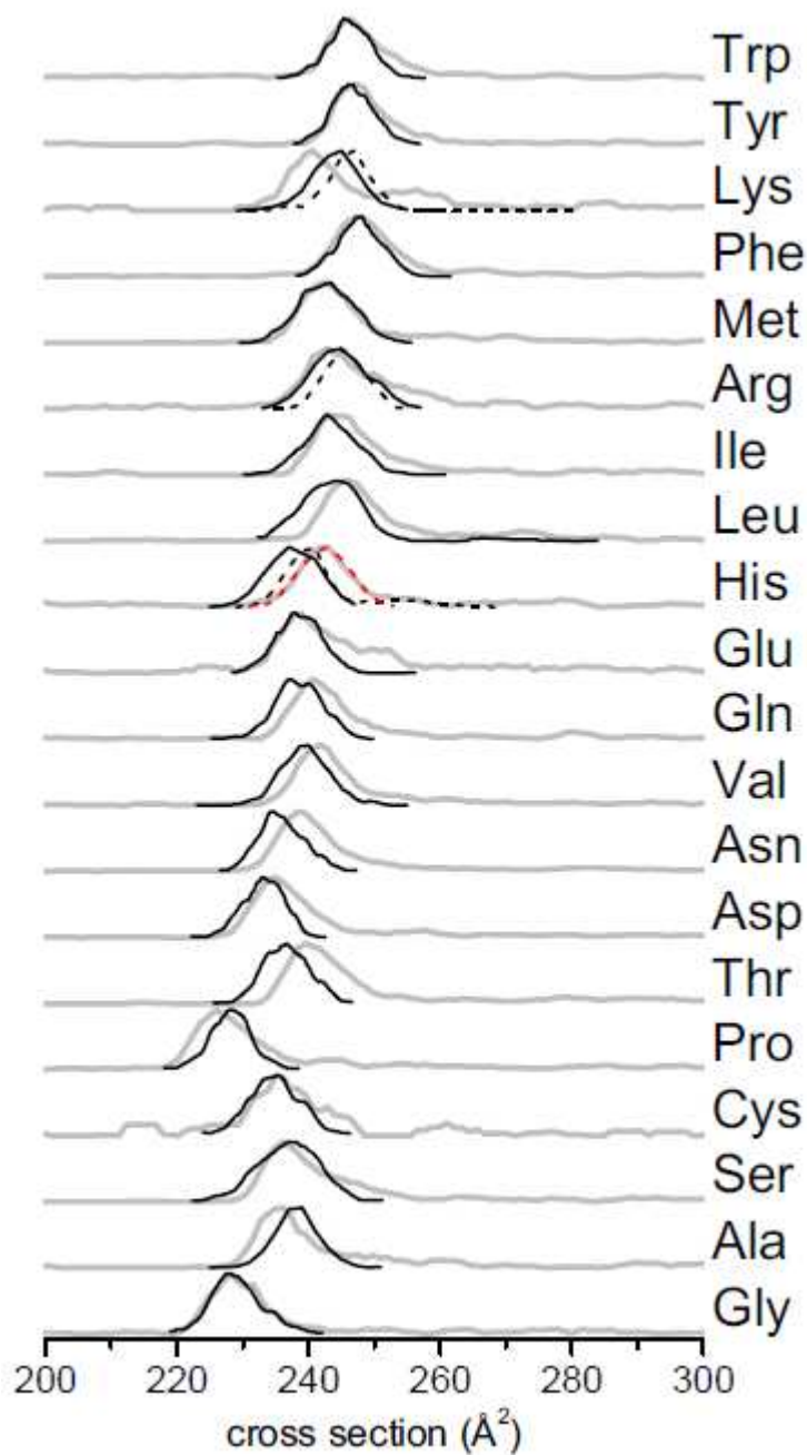
Figure III-2 : Profils des sections efficaces de diffusion expérimentales (gris) et théoriques (noir) pour la série des polyalanines. Les profils en noir représentent les distributions calculées pour une protonation sur l'arginine 1 et la lysine 11. Les profils en pointillés correspondent à une protonation sur l'arginine en position 1 et sur le résidu X en position 6 (pour les résidus basiques, avec X=His, Lys et Arg). Pour X=His les distributions correspondant aux deux formes tautomères de l'histidine centrale neutre sont représentées en trait noir et en pointillés rouges.
