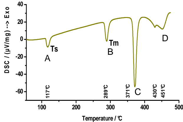
Figure 1. Courbe de DSC du composite MgH_2-2LiBH_4 (sous argon 100\text{ ml}\cdot\text{min}^{-1} , chauffe 5\text{ K}\cdot\text{min}^{-1} )
