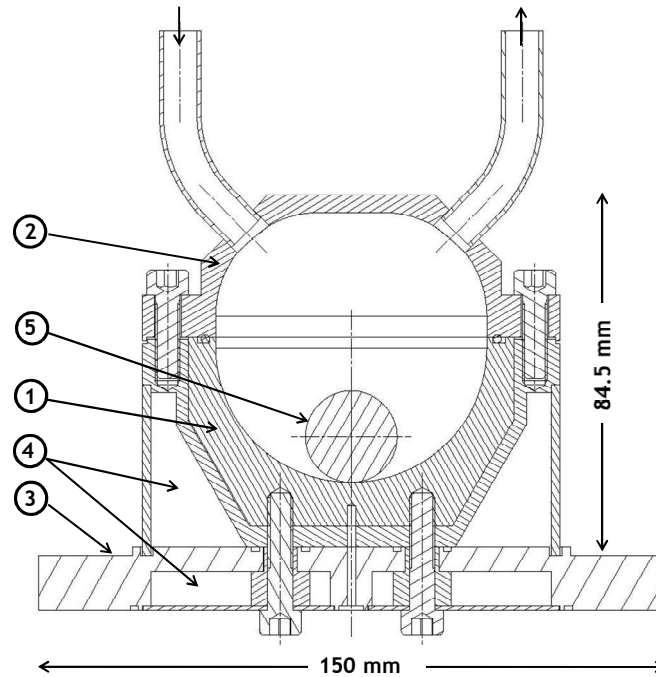
Figure 14. Coupe transversale du dispositif de broyage. (1) bol; (2) couvercle étanche muni d'un joint "Viton ® "; (3) plaque support; (4) espace creux pour la circulation d'air chaud; (5) bille \varnothing 20-30 mm.
