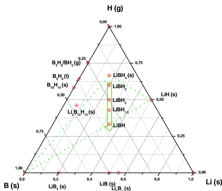
Figure 8. Diagramme de phase du system Li-B-H incluant les composés hypothétiques \text{LiBH}_{4-\epsilon}
