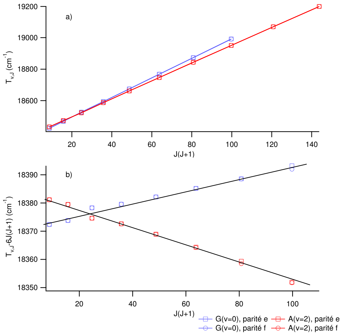
FIGURE III.2 – Un agrandissement de la zone 18400\text{-}19200\text{ cm}^{-1} illustrant une perturbation rotationnelle localisée à J = 4\frac{1}{2} entre 2 états électroniques \Omega' = 5/2 très proches en énergie : l'état G(v' = 0) et l'état A(v' = 2) . Le graphique b représente des termes d'énergie réduite en prenant B_{\text{eff}} = 6\text{ cm}^{-1} .
