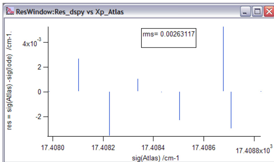
FIGURE II.23 – Résultat de la calibration. La déviation standard de chaque raie du spectre de référence de I 2 enregistré en même temps est représentée graphiquement en cm -1 .
