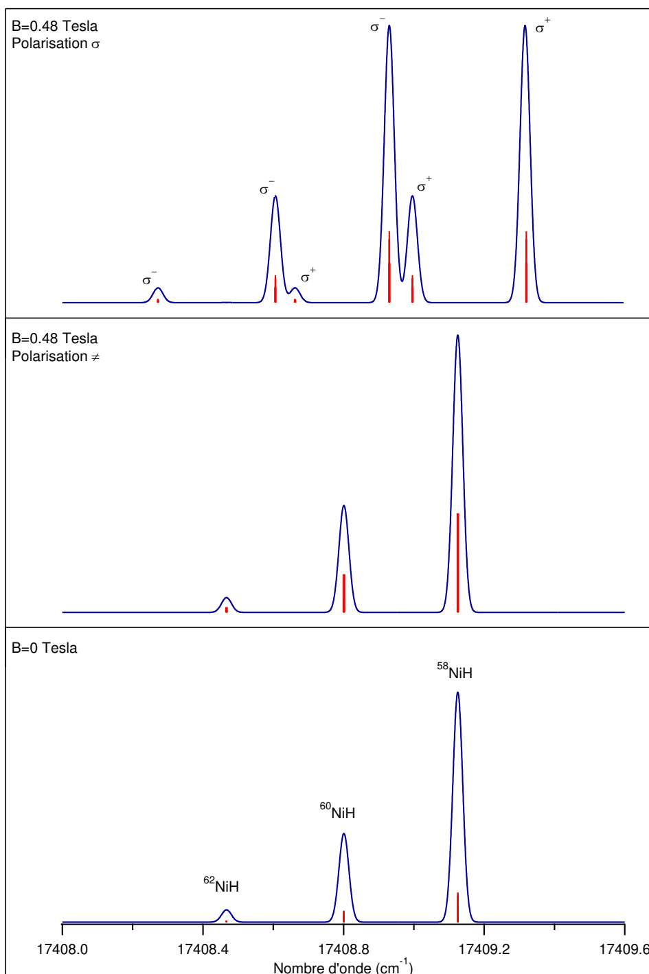
FIGURE I.14 – Modélisation de la raie Q(2^{1/2}) de la transition B \leftarrow X_1(2^2_{5/2})(1-0) en champ nul et soumise à un champ magnétique de 0.48 T. La séparation des composantes n'est pas observable, cependant celle-ci reste inférieure à la résolution de nos mesures. On peut donc faire l'approximation que toutes les composantes des sous-niveaux Zeeman ont la même fréquence afin de déterminer les valeurs des facteurs de Landé.
