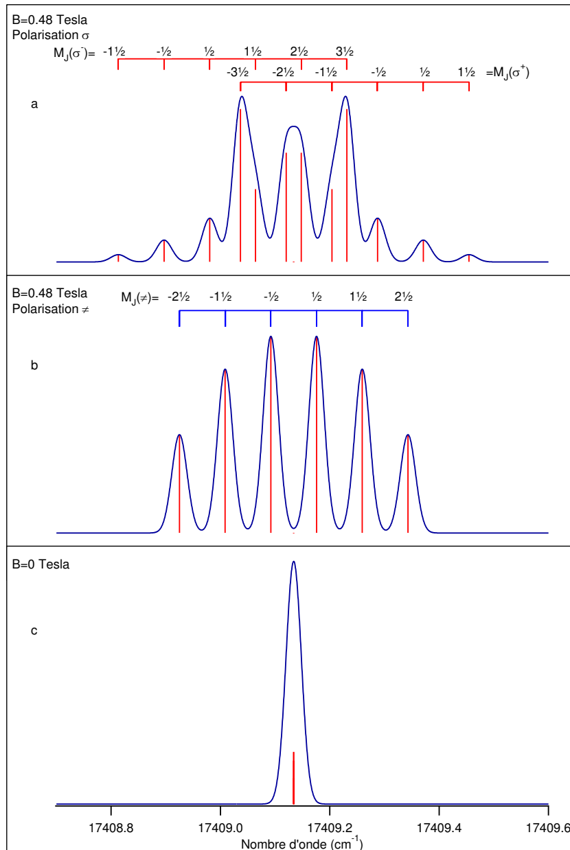
FIGURE I.10 – Modélisation de la raie P(3^{1/2}) de la transition B \leftarrow X_1 ({}^2\Delta_{5/2}) (1 - 0) . Le contour est obtenu à partir des transitions du spectre bâton (rouge) convolués avec un profil gaussien. La largeur à mi-hauteur ( fwhm ) choisie ici est de 0.033 \text{ cm}^{-1} .
