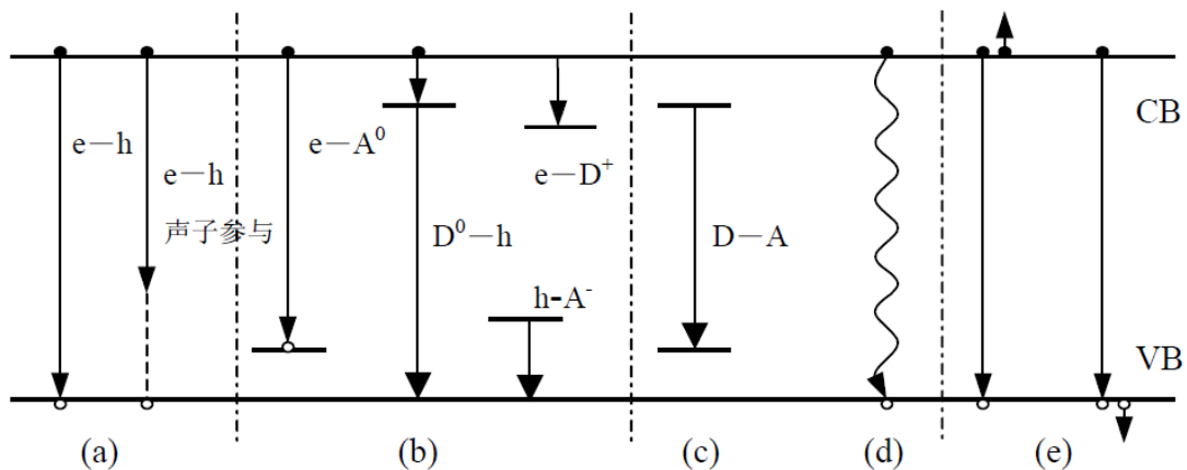
图 3-5. 半导体材料中几种常见的辐射复合过程。
