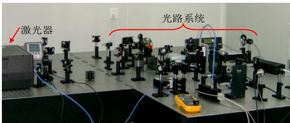
图 5-3. 光路系统实物图。
