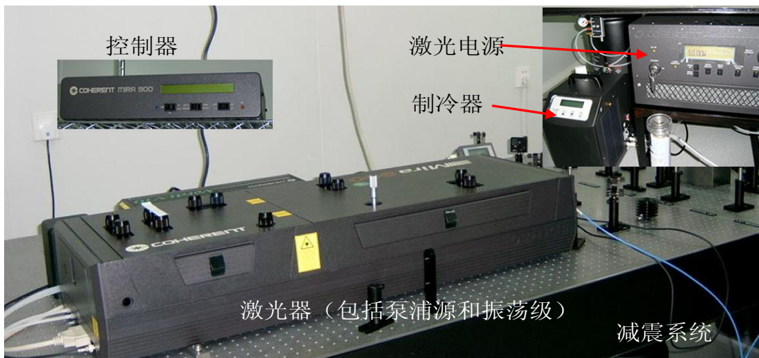
图 5-2. 脉冲光源激光器系统实物图。
