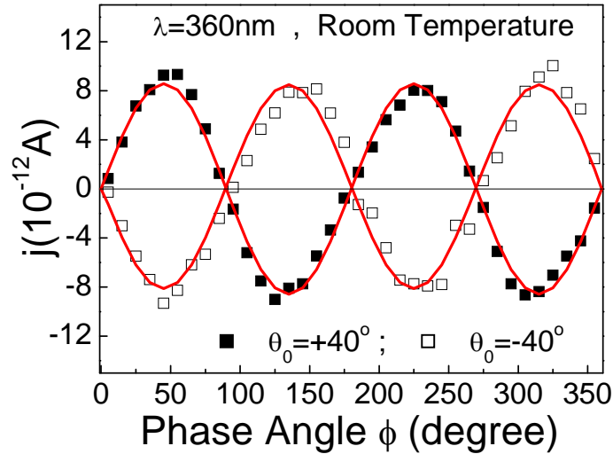
图 7-6. GaN/AlGaN 二维电子气样品面内光电流与入射光位相角 \phi 的关系（入射角 \theta_0 = \pm 40^\circ ），激发功率为 70mW。
