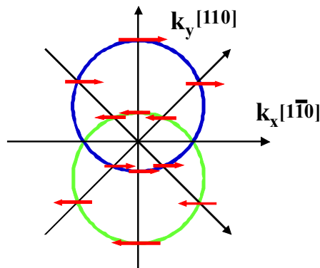
图 6-2. (001) 晶向生长的 GaAs/AlGaAs 二维电子气中 k 空间内电子自旋的定向分布示意图。
