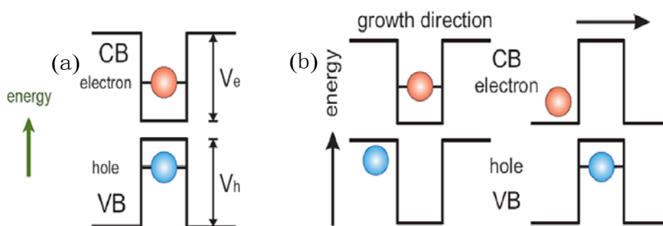
图 9-1. (a) I 型能带结构; (b) II 型能带结构。
