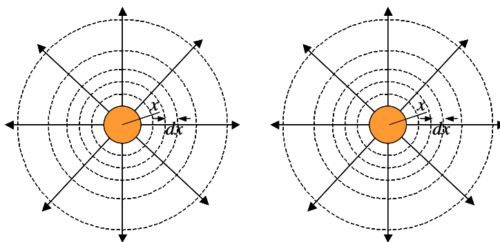
Figure IV-16 Cas où les équipotentielles circulaires sont centrées sur les contacts. En traits discontinus sont représentées les équipotentielles cylindriques et en traits continus les lignes de courant.
