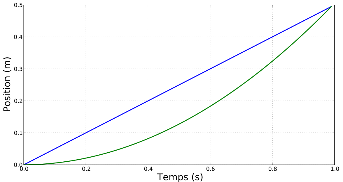
Figure 2.1 – En bleu, trajectoire interpolée d'un solide en mouvement uniformément accéléré. En rouge, trajectoire réelle.
