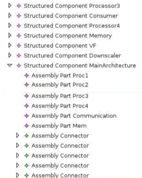
Figure 8.9: Exemple d'architecture d'un modèle downscaler , conforme au métamodèle Marte.
