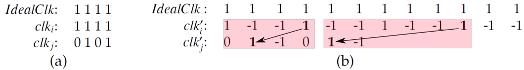
Figure 7.9: Légende: (a) une trace de deux horloges binaires finies clk_i et clk_j et (b), une trace de deux horloges étendues clk'_i et clk'_j résultantes de l'expansion de clk_i et clk_j avec c_i = 3 et c_j = 2 et ayant les contraintes de dépendances violées.
