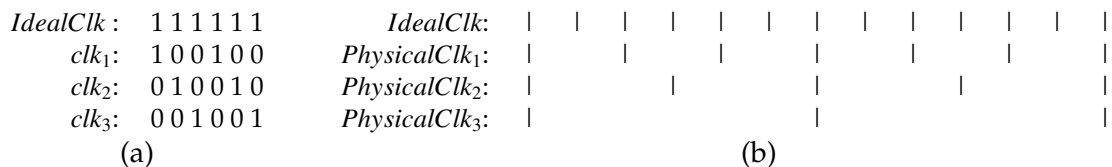
Figure 6.6: Légende: (a) une trace de trois horloges abstraites fonctionnelles et (b), une trace de trois horloges abstraites physiques selon une horloge de référence.
