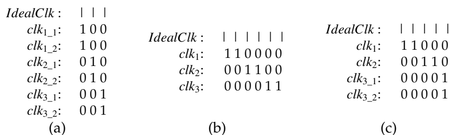
Figure 5.6: Légende: (a) une trace d'horloges fonctionnelles selon le modèle d'exécution parallèle, (b) une trace d'horloges fonctionnelles selon le modèle d'exécution pipeline et (c) une trace d'horloges fonctionnelles selon le modèle d'exécution pipeline pour clk_1 et clk_2 et parallèle pour clk_3 .
