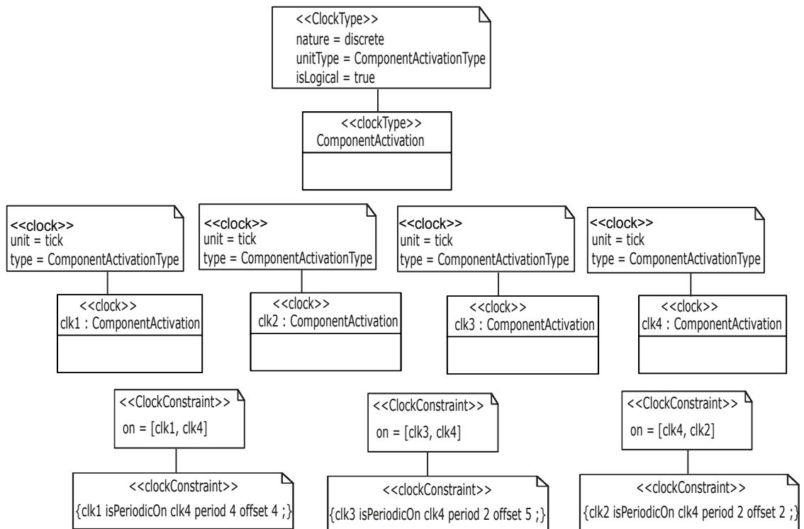
Figure 5.8: Contraintes temporelles spécifiées en Marte.
