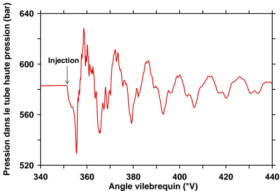
Figure IV-24: Exemple d'oscillations de pression dans le tube haute pression pour une injection telle que \phi_{inj} = 350^\circ , P_{inj} = 600\text{ bar} , \Delta T_i = 270\ \mu\text{s}
