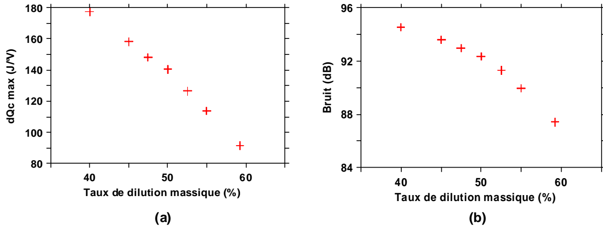
Figure V-27: Évolution du pic de taux de dégagement de chaleur (a) et du bruit (b) en fonction du taux de dilution massique, diluant: N_2
