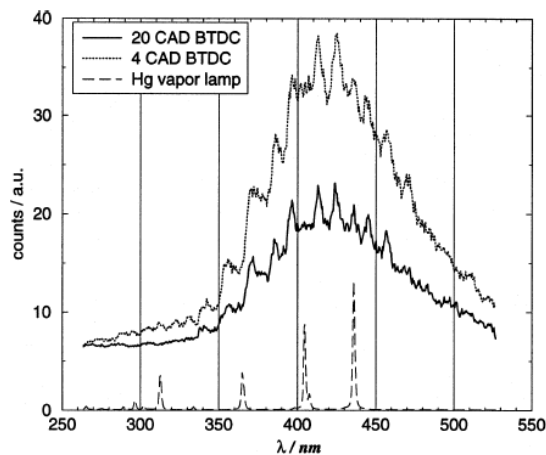
Figure II-3: Spectre d'émission du formaldéhyde, PRF 35, \Phi = 0.3 , d'après [56]
