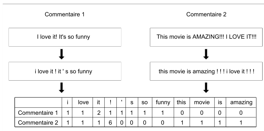
FIGURE 5.2 – Exemples de vectorisation de textes
