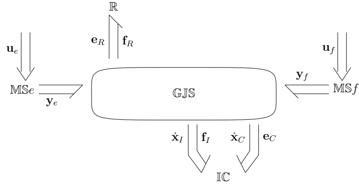
FIGURE 4.1 – Modèle bond graph générique (cas linéaire)
