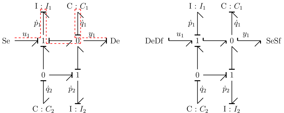
(b) Sous-modèle bond graph bicausal associé au chemin ①
