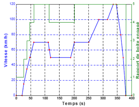
FIGURE 2.24 – Cycle normalisé EUDC [Laf04]
