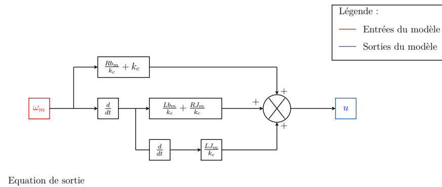
(b) Modèle inverse correspondant au système d'équations (2.6)
