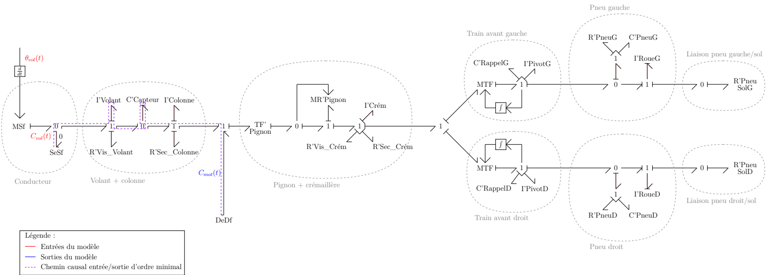
FIGURE 2.16 – Dimensionnement d'une direction assistée électrique : étape d'adéquation (suite)
