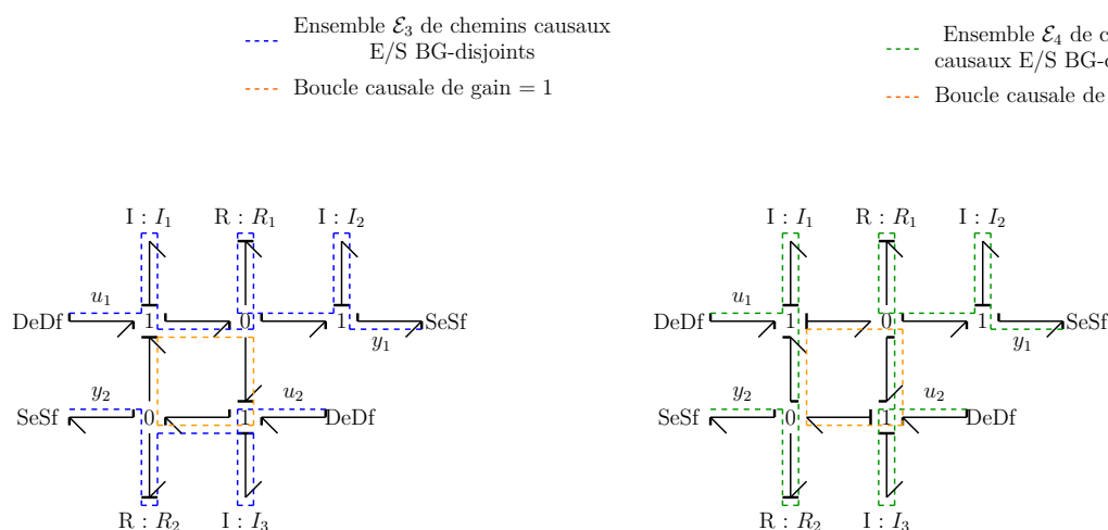
(a) Modèle bond graph bicausal n°1 (b) Modèle bond graph bicausal n°2
