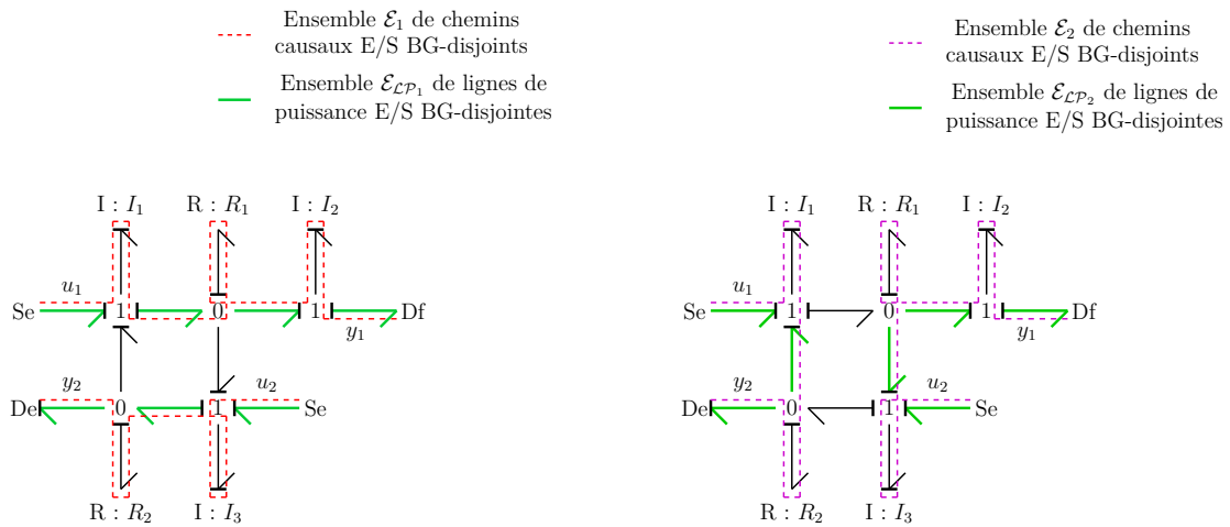
(a) Modèle bond graph causal (b) Modèle bond graph causal
