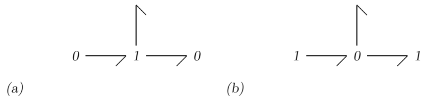
FIGURE A.4 – Jonctions et liens de puissance faisant apparaître (a) les différences de potentiels et de pressions, (b) les différences de vitesses [Fav97]
