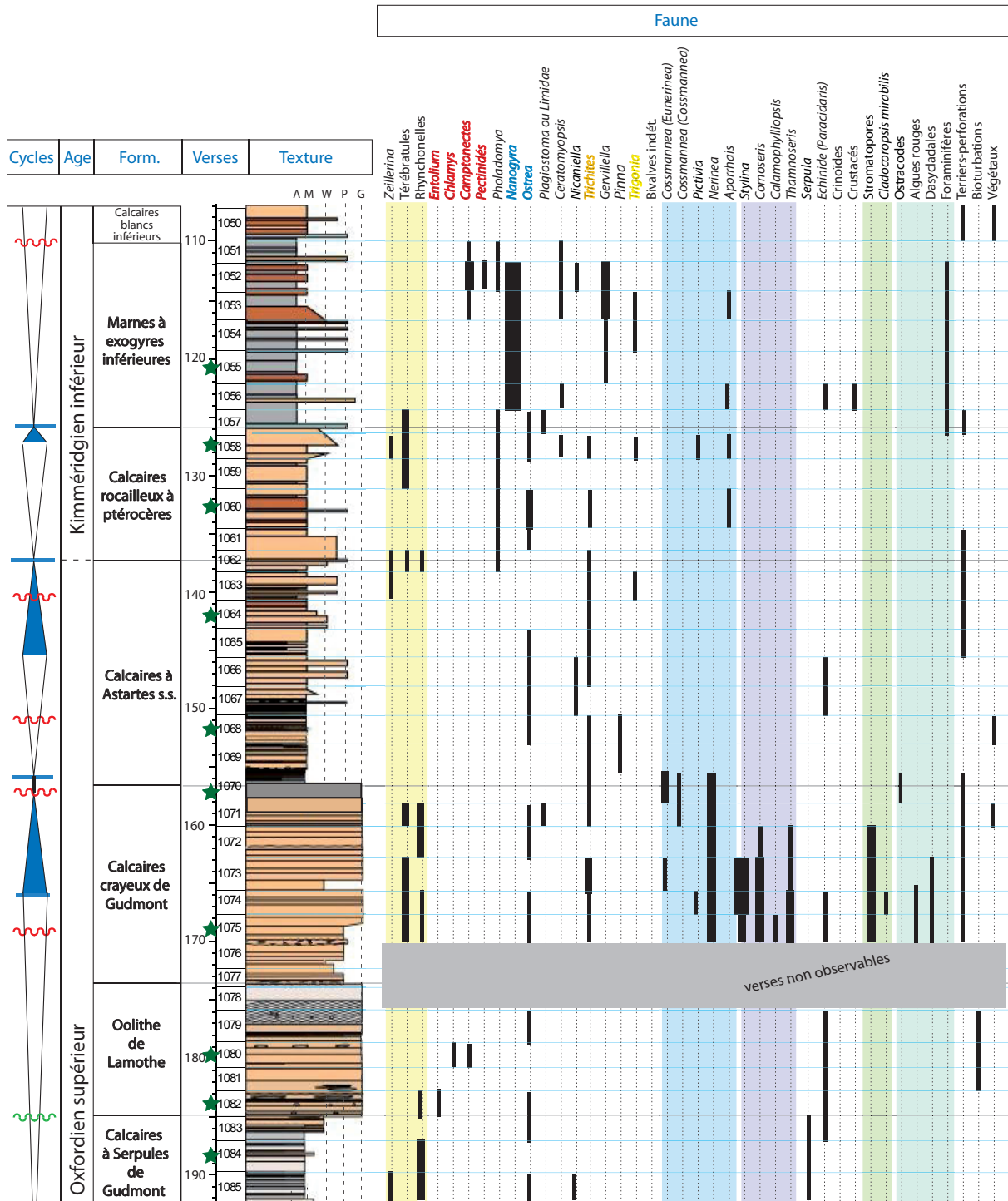
Figure 3.16. Coupe lithologique du puits principal d'accès de Bure, distribution des macrofossiles d'après Lathuilière et al. (2006) et cadre séquentiel. Les étoiles vertes indiquent les verses qui ont été échantillonnées pour l'analyse de la matière organique soluble.
