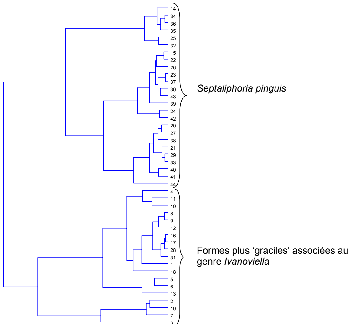
Figure 3.27. Classification hiérarchique issue d'une analyse statistique (avec le logiciel PAST) constituant 2 groupes distincts d'un point de vue morphologique au sein de la population de rhynchonelles du niveau G1B de la coupe de Gudmont-Villiers
