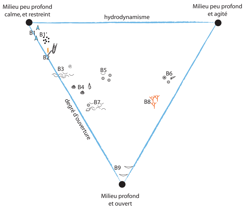
Figure 4.22. Modèle de dépôt schématisant plaçant les 9 faciès (B1 à B9) définis dans le tableau 4.1. Les échantillons sont distribués suivant 3 pôles caractérisant les milieux extrêmes de la plate-forme carbonatée du Berry : un pôle caractérisant des environnements peu profonds, restreints et calmes, un pôle caractérisant des environnements moins protégés et/ou plus profonds et un pôle caractérisant des environnements peu profonds, restreints mais calmes.
