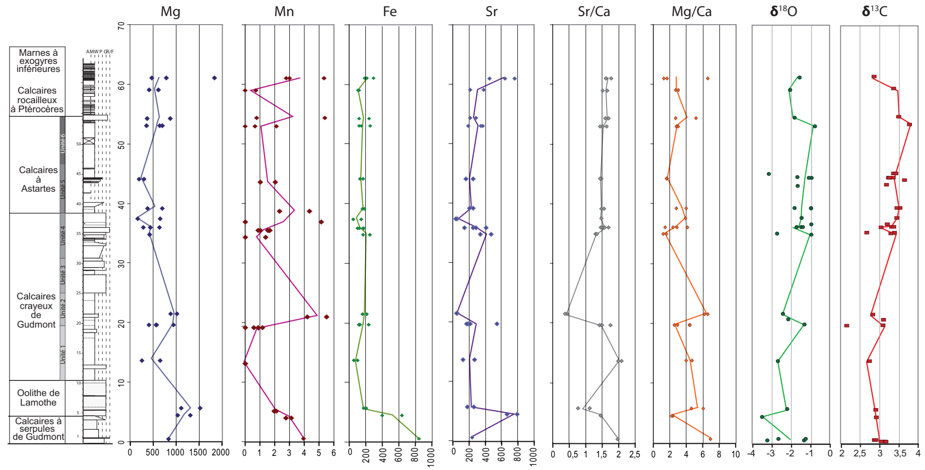
Fig. 3.11. Comparaison de l'évolution des éléments majeurs (Mg, Mn, Fe) et trace (Sr), des rapports Mg/Ca et des valeurs \delta^{18}\text{O} et \delta^{13}\text{C} des coquilles sur la coupe de Gudmont-Villiers. Les courbes passent par la moyenne des points pour un banc.
