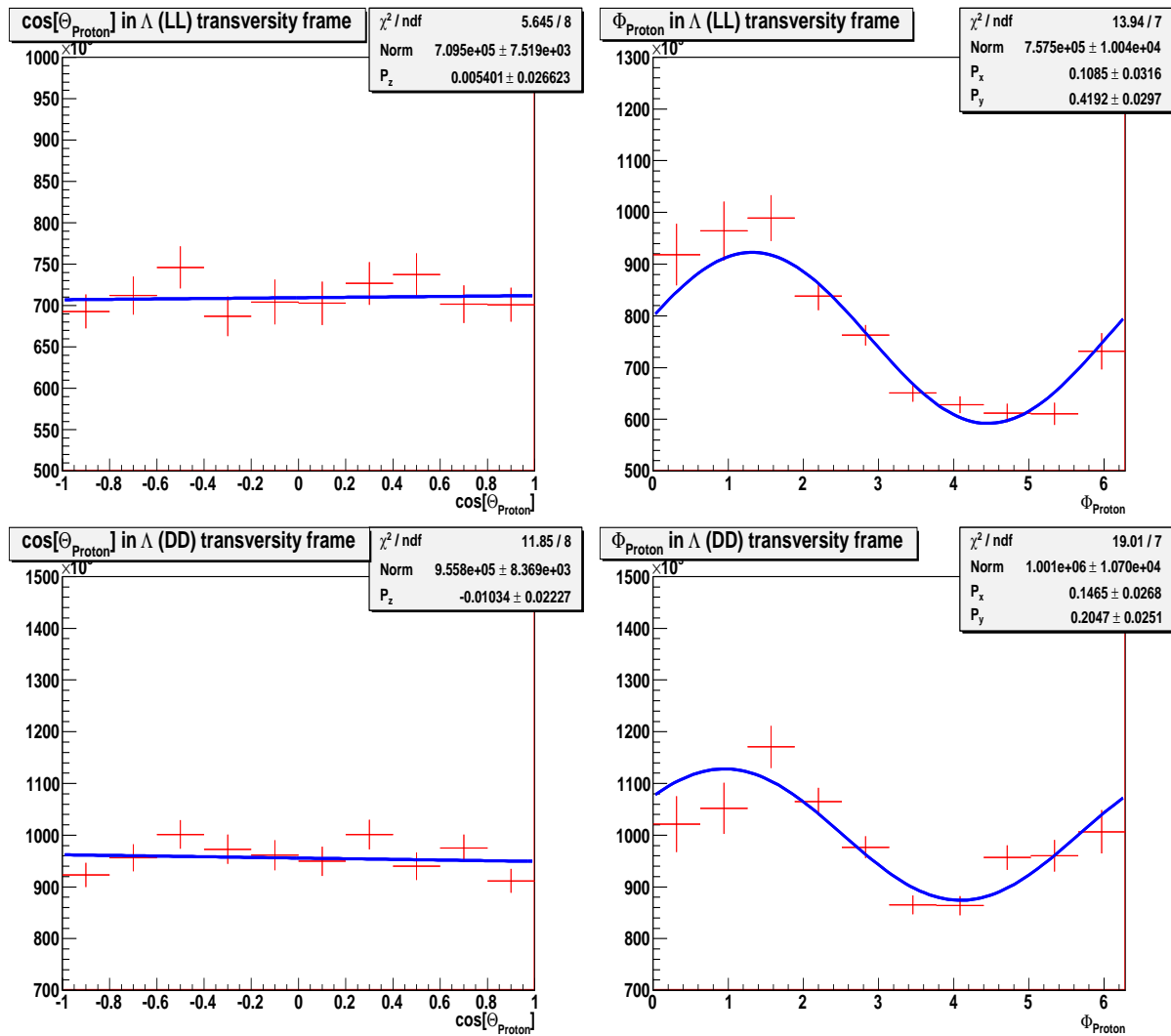
FIGURE 6.10 – Distributions angulaires en \cos \theta et \phi pour les candidats \bar{\Lambda} (LL) et (DD) dans le repère de transversité du \bar{\Lambda} .
