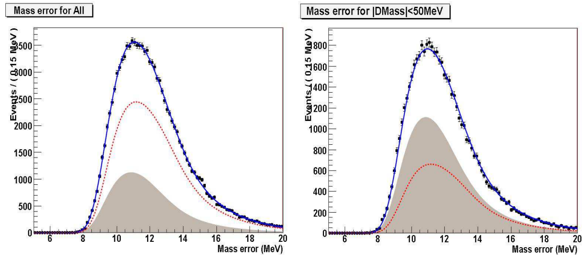
FIGURE 4.22 – Deux projections de la résolution sur la masse reconstruite \sigma^m pour les candidats B_d^0 \rightarrow J/\psi K_s^0 : la première pour une fenêtre de masse de [-120, 250] MeV et l’autre en se limitant à \pm 50 MeV. La courbe bleue est le résultat d’un ajustement global. La courbe en tiret rouge et la partie grise correspondent à la contribution du bruit de fond et à celle du signal respectivement.
