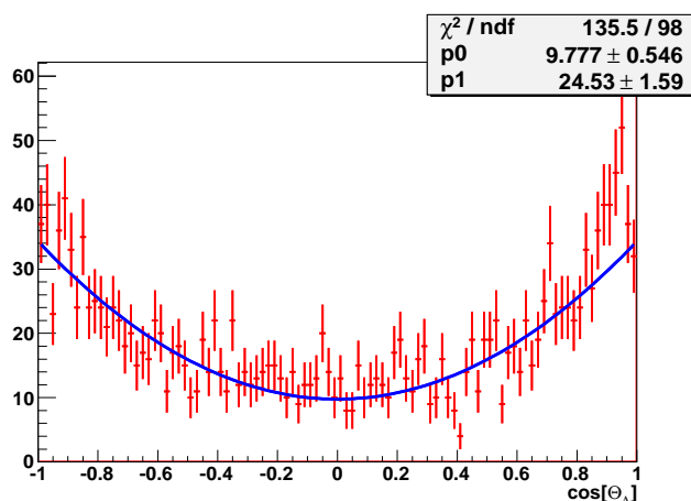
FIGURE 5.18 – Distribution en \cos\theta_\Lambda du \Lambda dans le repère propre du \Lambda_b calculé à partir des événements \Lambda_b \rightarrow \Lambda J/\psi sélectionnés à partir d'un échantillon de polarisation \Lambda_b nulle.
