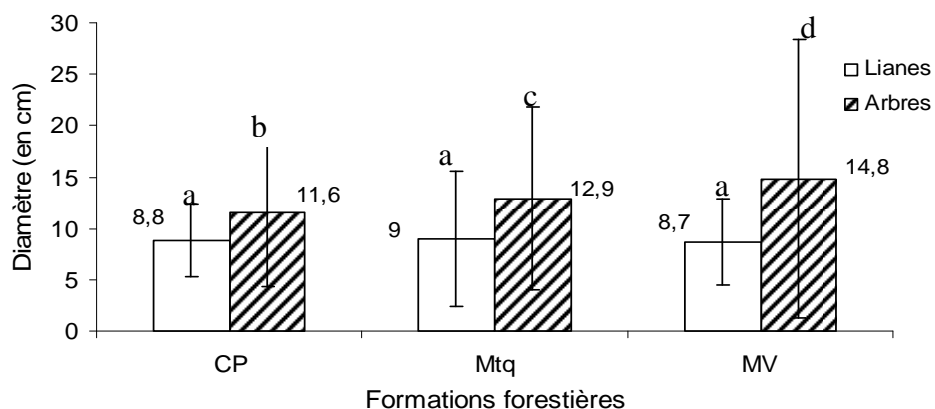
Figure 16 Diamètre moyen des arbres et écart-type ( n=2395 tiges) et des lianes ( n=108 tiges) dans les formations forestières (CP= capoeira, Mtq= mata queimada, MV=mata virgem). Des lettres différentes sont attribuées lorsque les moyennes sont significativement différentes. Test de Student pour les arbres : t(MV-CP)=-5,99 , ddl=1485 , P<0,01 ; t(Mtq-CP)=-2,92 , ddl=1430 , P<0,01 ; t(MV-Mtq)=3,63 , ddl=1666 , P<0,01 . Anova pour les lianes : F=0,05 , ddl=108 et P>0,05 .
