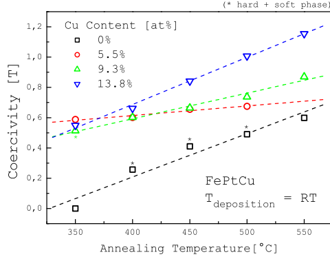
(a) Coercivité en fonction de T_{\text{Recuit}} pour des dépôts à T_{\text{Substrat}} = \text{RT}
