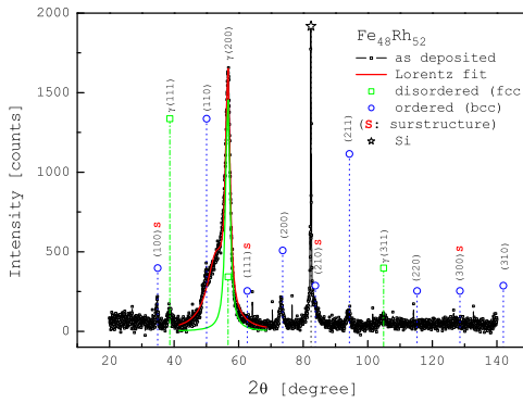
(e) DRX pour la couche de 52%Rh
