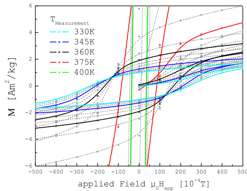
(e) Zoom en champs faibles cas 52.2%Rh
