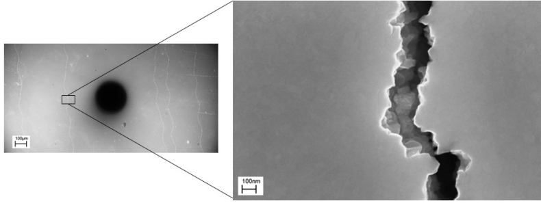
FIGURE III.5 – Visualisation par microscopie électronique à balayage de l'état de surface de l'échantillon de 2μm après un recuit de 700°C pendant 30min.
