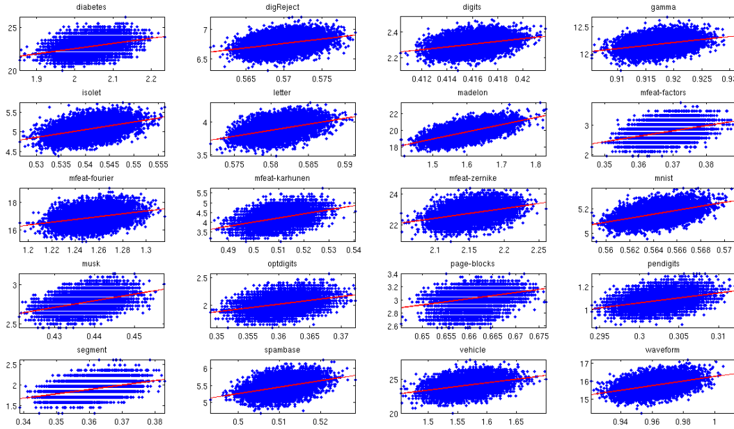
FIG. 4.15: Taux d'erreur en test en fonction de \bar{\rho}_{s^2} obtenus au cours du processus de sélection par algorithme génétique, pour des sous-forêts de 200 arbres. Chaque point représente une de ces sous-forêts avec en abscisse sa valeur de \bar{\rho}_{s^2} et en ordonnée son taux d'erreur sur l'ensemble de test. La ligne rouge représente la droite de régression du nuage de points.
