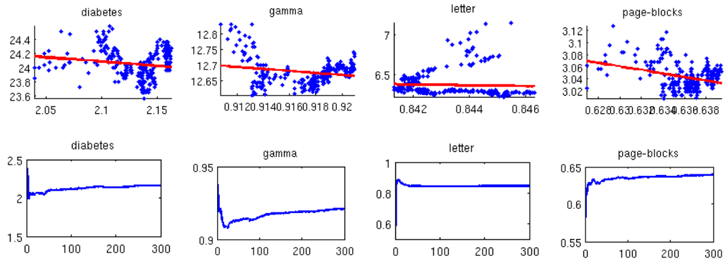
FIG. 4.8: Taux d'erreur des sous-forêts en fonction de \frac{\bar{\rho}}{s^2} pour les bases Diabetes, Gamma, Letter et Page-blocks
