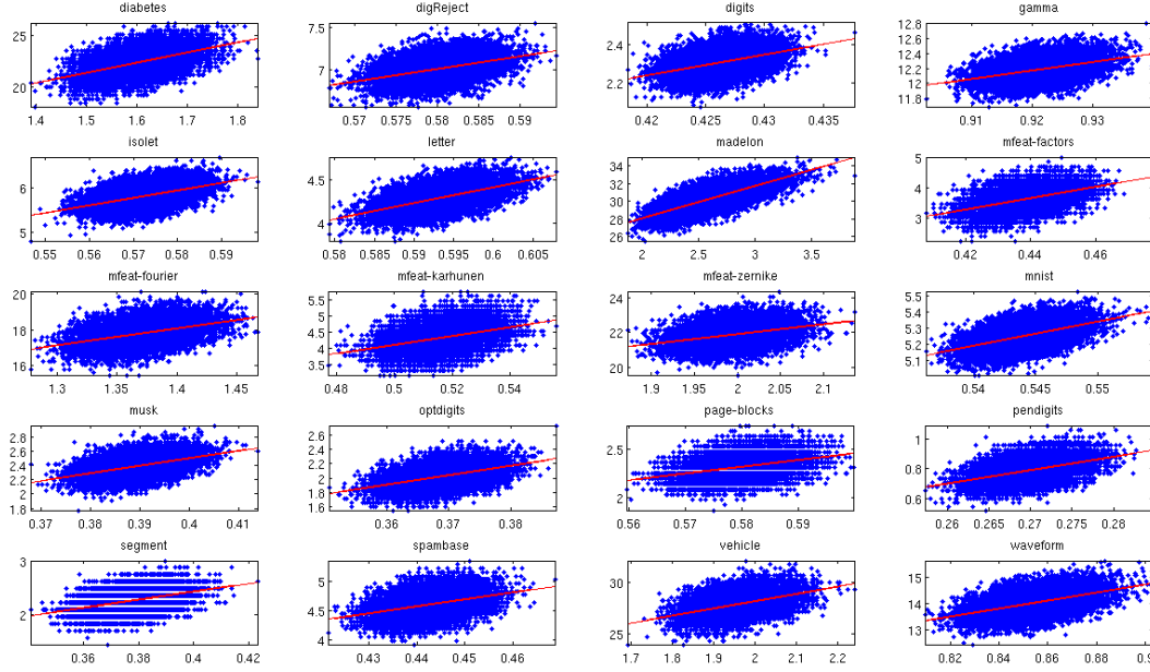
FIG. 4.13: Taux d'erreur en test en fonction de \bar{\rho}_{s^2} obtenus au cours du processus de sélection par algorithme génétique, pour des sous-forêts de 100 arbres. Chaque point représente une de ces sous-forêts avec en abscisse sa valeur de \bar{\rho}_{s^2} et en ordonnée son taux d'erreur sur l'ensemble de test. La ligne rouge représente la droite de régression du nuage de points.
