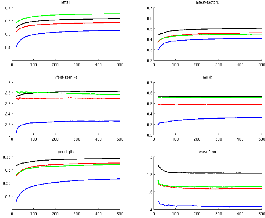
FIG. 5.8: Évolution du rapport \frac{\bar{\rho}}{s^2} en fonction du nombre d'arbres dans les forêts. Les courbes de Forest-RK sont représentées en noir. Les taux de \text{DRF}/W_1^{\text{inv}} correspondent aux courbes rouges ; ceux de \text{DRF}/W_5^{\text{pol}} aux courbes bleues ; et ceux de \text{DRF}/W_{10}^{\text{exp}} aux courbes vertes.
