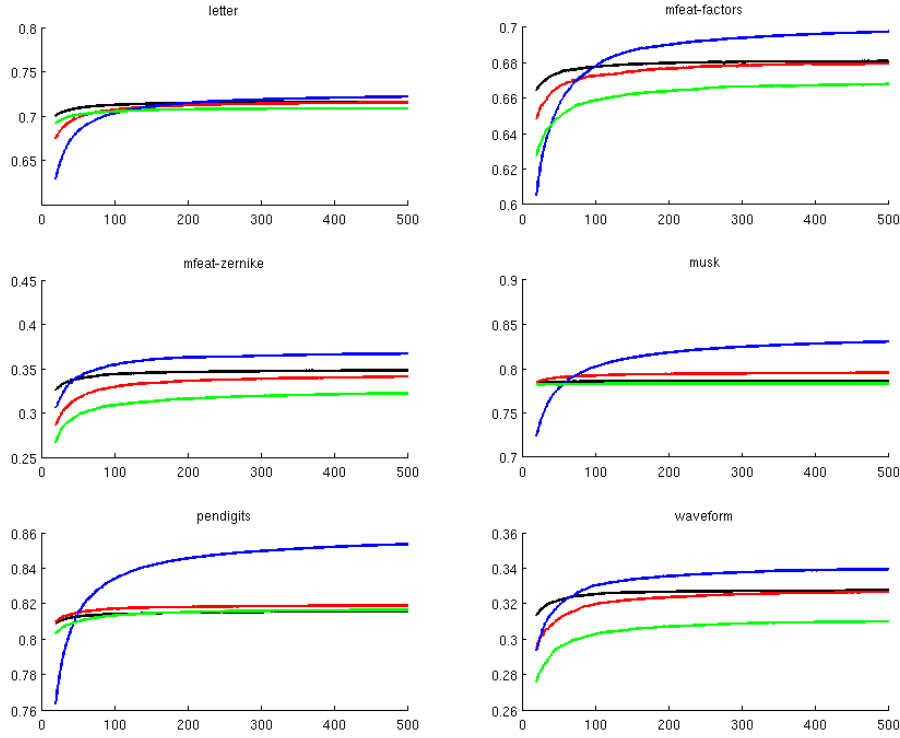
FIG. 5.6: Évolution de la force en fonction du nombre d'arbres dans les forêts. Les courbes de Forest-RK sont représentées en noir. Les taux de \text{DRF}/W_1^{\text{inv}} correspondent aux courbes rouges ; ceux de \text{DRF}/W_5^{\text{pol}} aux courbes bleues ; et ceux de \text{DRF}/W_{10}^{\text{exp}} aux courbes vertes.
