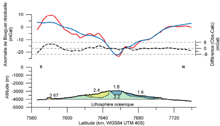
Profil E3
