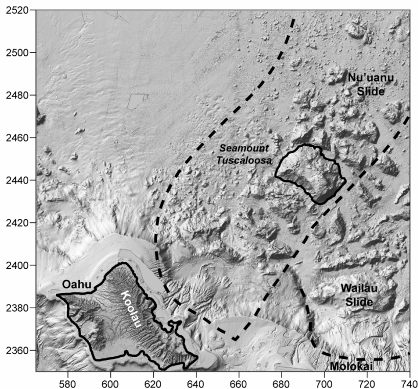
Figure 5-03: a) MNT de l'île de Oahu (Hawaii) et bathymétrie associée (sources MNT : http://www.soest.hawaii.edu/HMT:index.php ). Les secteurs en pointillés délimitent les glissements de Nu'uaniu et de Wailau et les mégablocs associés (d'après Moore et al., 1989, 1994a, b ; Moore et Clague 2002).
