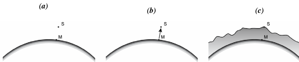
Figure 2-15: Principe du calcul de l'anomalie de Bouguer. a) Modèle de Terre ; b) Correction à l'air libre ; c) Corrections de plateau, de courbure et topographique.
