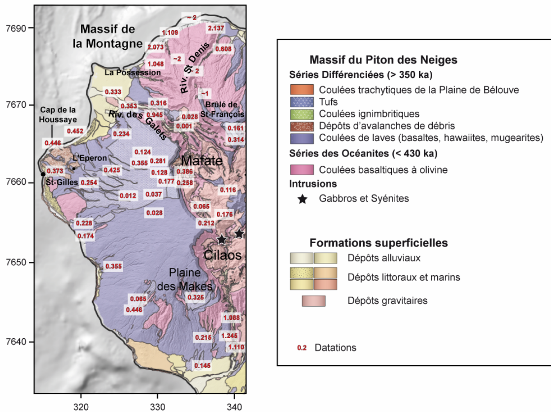
Figure 3-12 : Extrait de la carte géologique simplifiée de la partie occidentale du massif du Piton des Neiges, drapé sur le MNT de l'IGN à 25 m de résolution.
