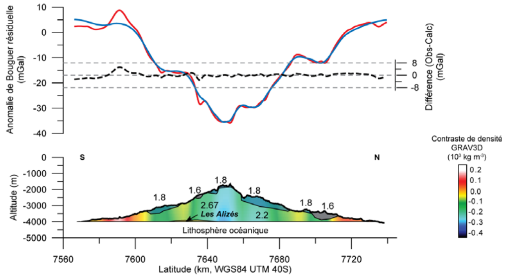
Profil E2
