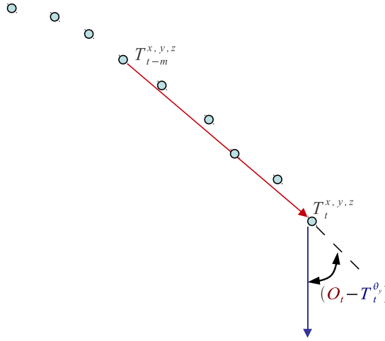
FIGURE 4.11 – Pseudo-observation de l'orientation de la personne en fonction de la trajectoire de marche.
