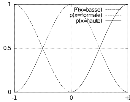
FIGURE 3.6 – Filtres flous utilisés pour le calcul des vraisemblances.
