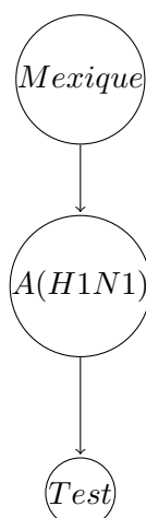
FIGURE 1.1 – Indépendance conditionnelle
