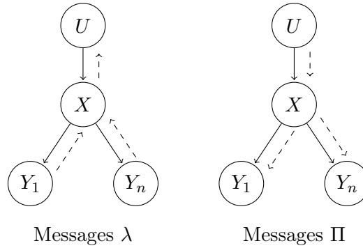
FIGURE 1.5 – Propagation des messages \lambda et \Pi dans l'arbre.
