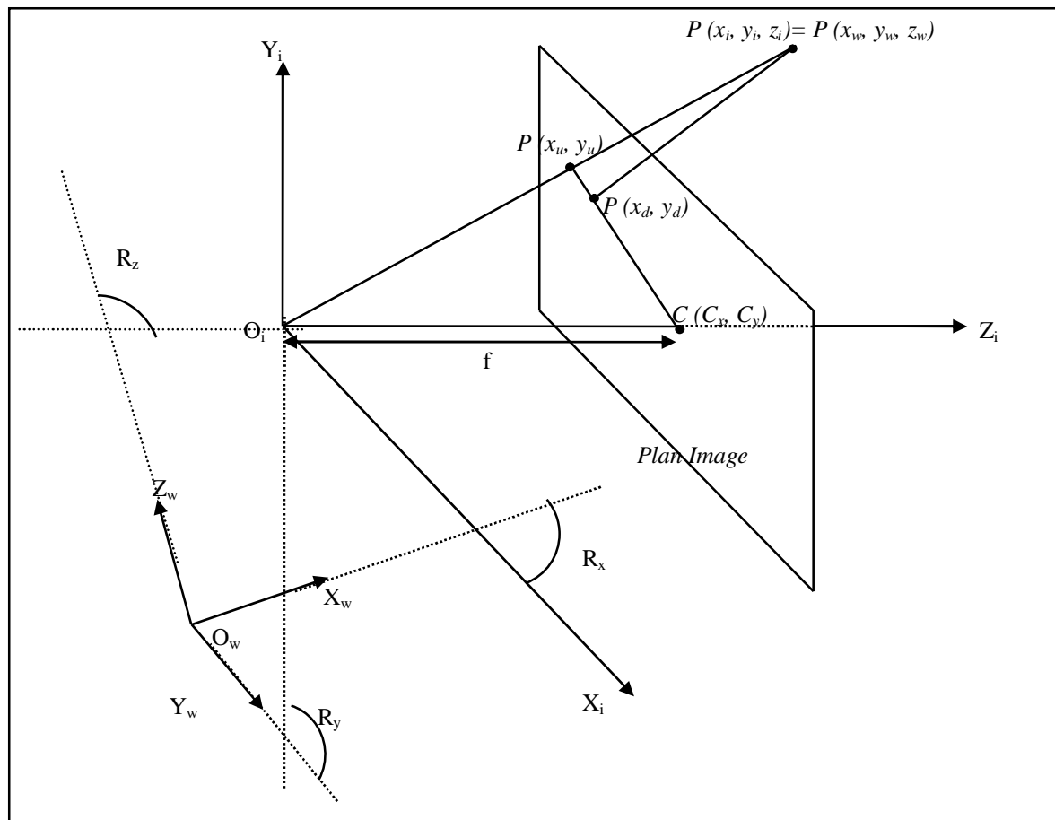
fig. A.1 : Le point P de coordonnées (x_w, y_w, z_w) dans le repère de la scène ( O_w, X_w, Y_w, Z_w ) est projeté dans le repère caméra ( O_i, X_i, Y_i, Z_i ). Son image sera formée à l'intersection du rayon le reliant à la caméra avec le plan image.
