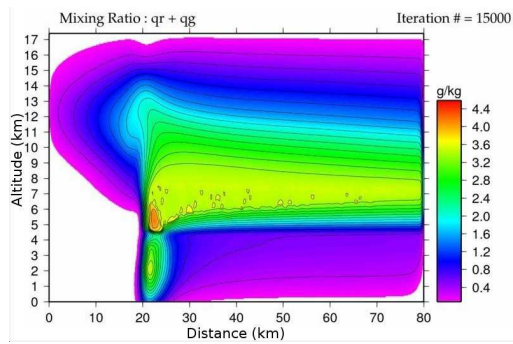
(a) Itérations : 15000
