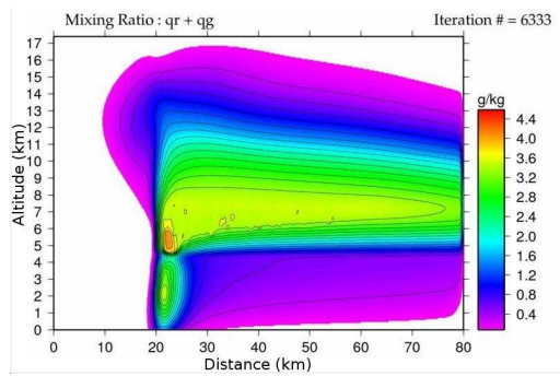
(b) Itérations : 6333
