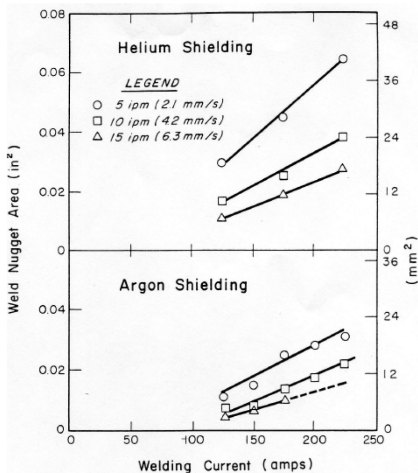
FIGURE 1.31 – Evolution de l'aire de la section du bain de soudage ( \text{mm}^2 ) en fonction du courant (A) d'une pièce en acier HY-80 en GTAW [33]
