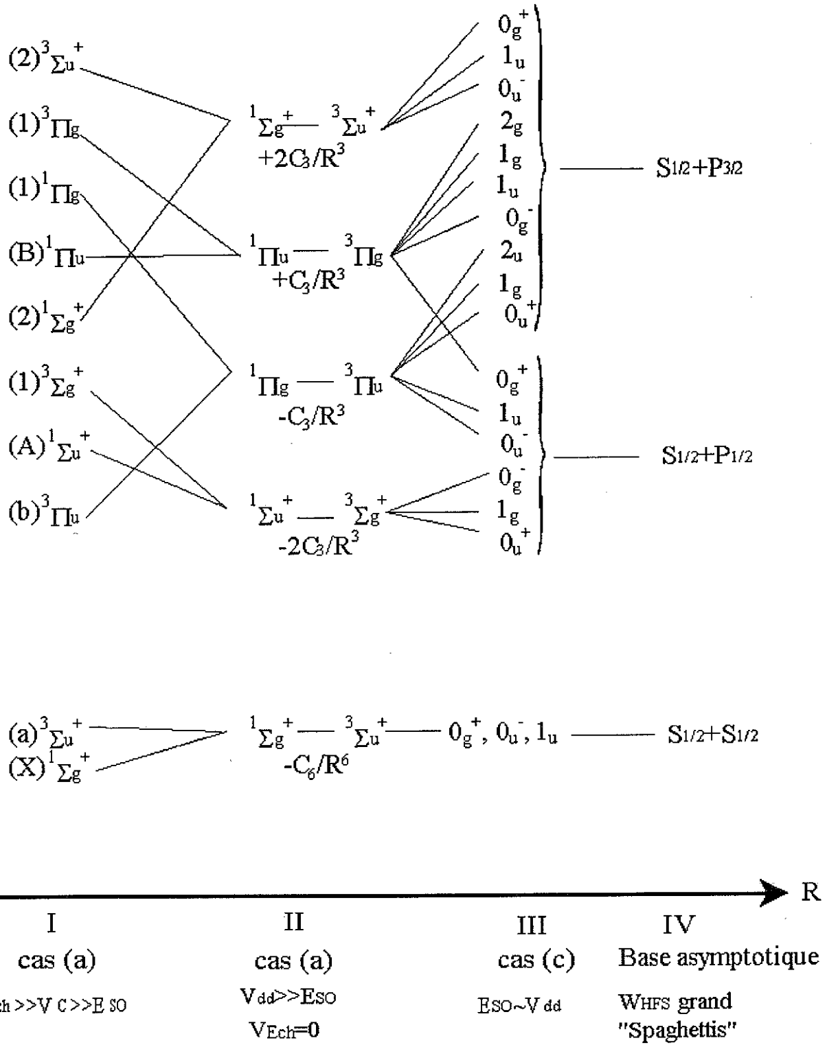
FIG. 2.3: Diagramme de corrélation pour les états électroniques se dissociant sous les limites ^{133}\text{Cs} ( 6S_{1/2} + 6S_{1/2} , 6S_{1/2} + 6P_{1/2} et 6S_{1/2} + 6P_{3/2} ). On représente quatre régions où les interactions dominantes varient, ainsi que les bases bien adaptées. Les variations énergétiques en C_n/R^n sont évaluées dans la section 5.3.1 page 135.
