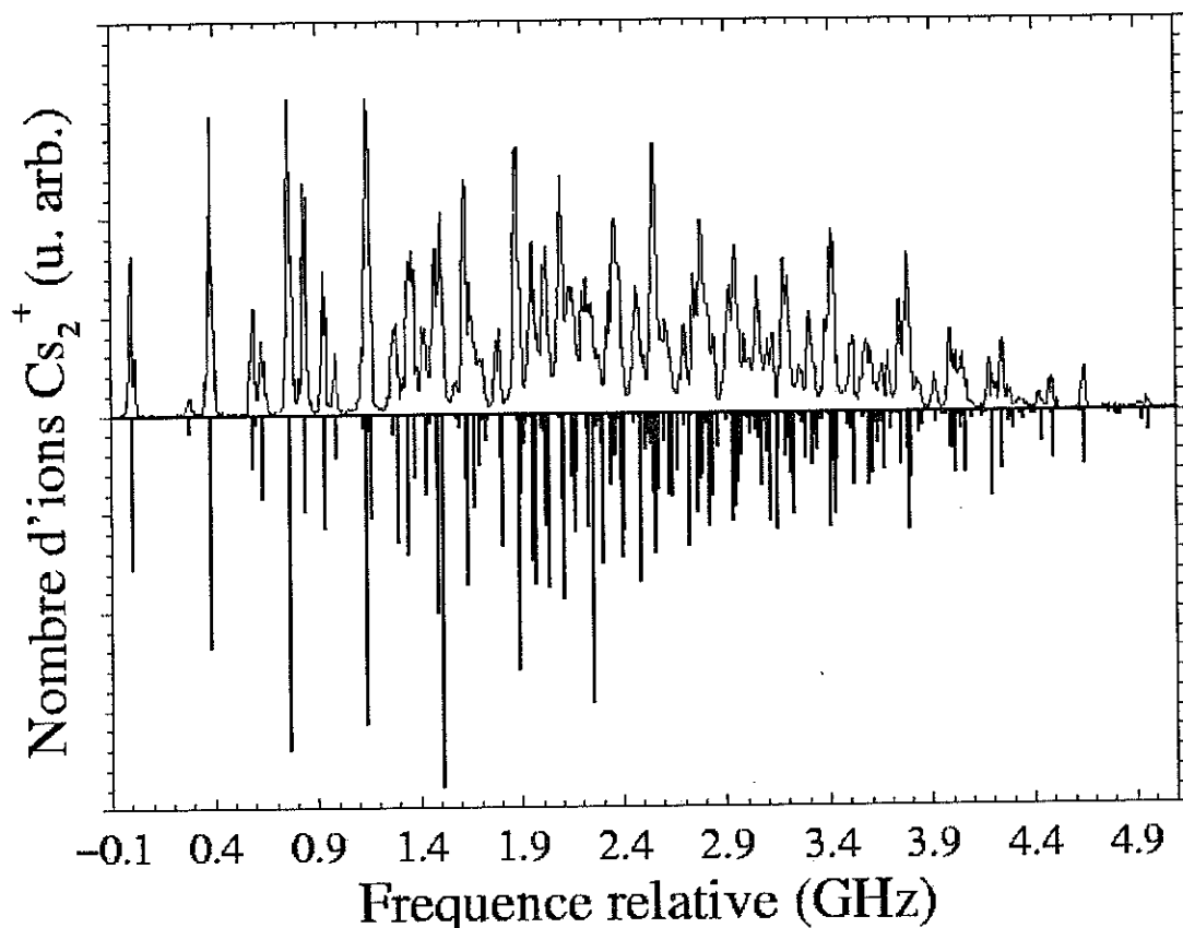
FIG. 5.11: Détail de la structure v = 1 de l'état 1_uP_{3/2} . On représente aussi le résultat du calcul de la position et de l'intensité relative des raies. Celle-ci est schématisée par la hauteur des barres.
