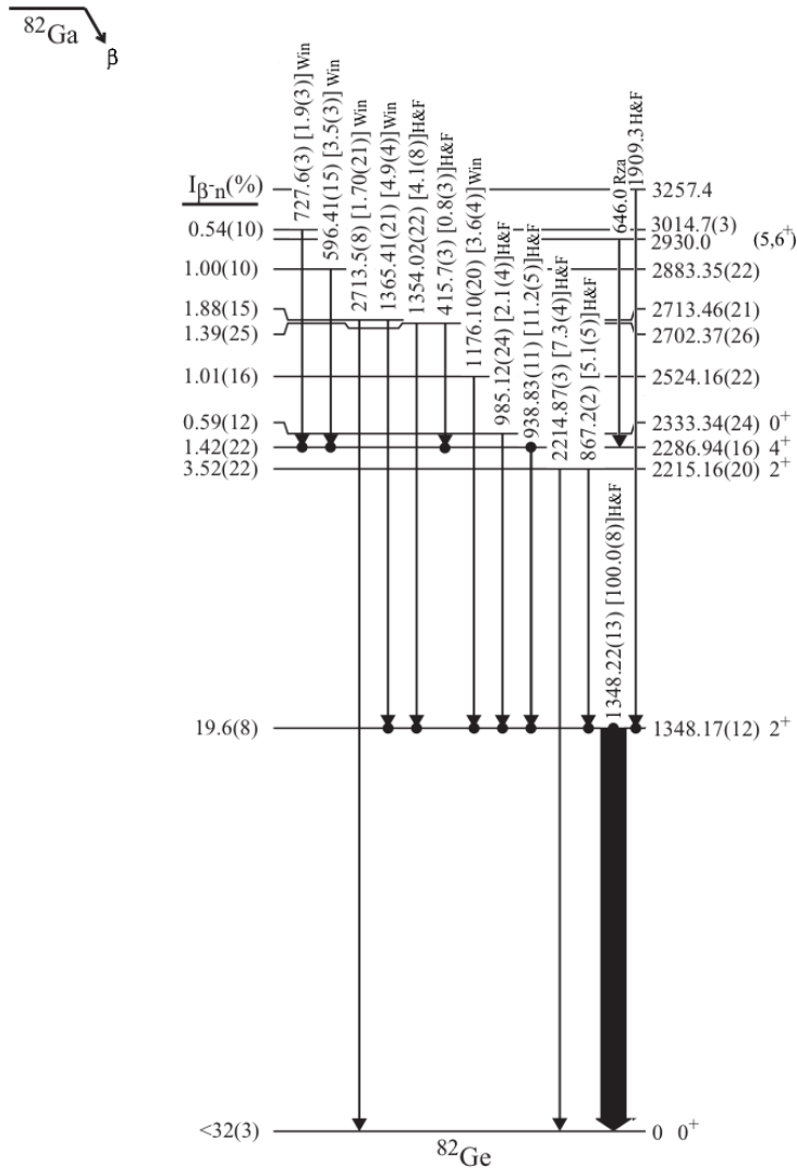
FIGURE V.15: Schéma des niveaux à basse énergie récapitulant les informations obtenues sur ^{82}Ge à partir des travaux de [Hof1981], [Win2010], et [Rza2007]. Les transitions marquées Win ont été proposées dans [Win2010], celles marquées H&F ont été proposées dans [Hof1981] et celle marquée Rza a été proposée dans [Rza2007].
