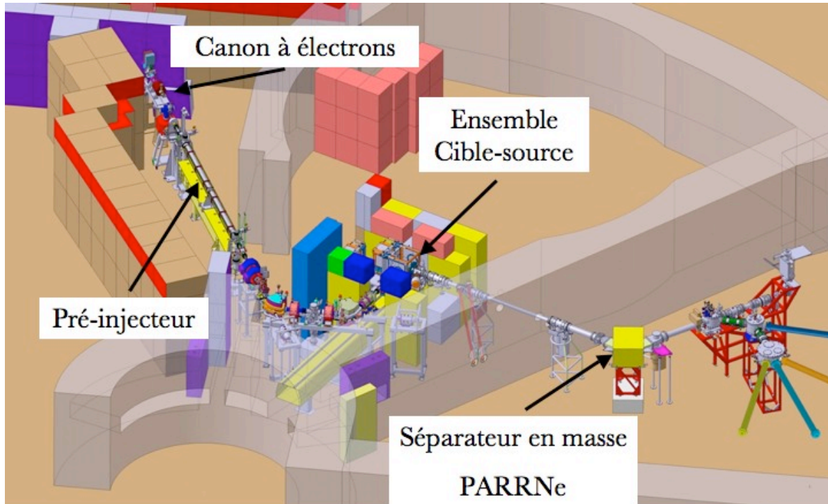
FIGURE III.1: Schéma de l'installation ALTO [Leb2008]
