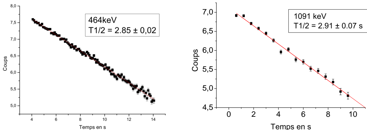
FIGURE V.9: A gauche le spectre en temps de la raie \gamma à 464 keV sur la partie de décroissance des cycles du ^{79}Ga . A droite, celui de la raie à 1091 keV. En rouge, la régression linéaire en échelle logarithmique de la décroissance faite avec l'équation \ln(N_0) - \frac{\ln 2}{T_{1/2}} * t . Chaque canal représente un intervalle de temps \Delta t = t_2 - t_1 , le contenu du canal est proportionnel au nombre de noyaux qui se sont désintégrés entre t_1 et t_2 . Les barres d'incertitudes sont parfois plus petites que les symboles. Les périodes T_{1/2} sont en secondes.
