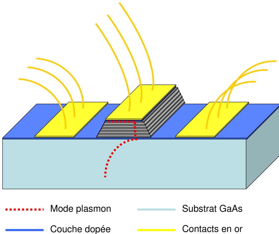
FIGURE 3.8: Représentation schématique d'un ruban laser à cascade quantique. Le mode plasmon servant à propager l'onde électromagnétique dans le guide est représenté en pointillés rouges.
