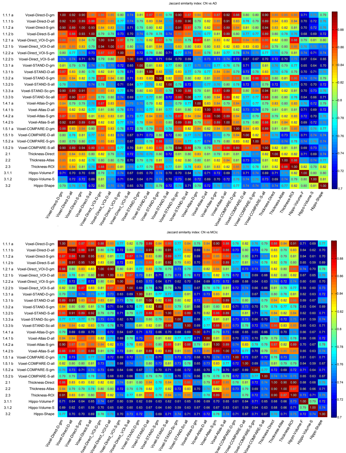
FIGURE 2.11 : Coefficient de similarité de Jaccard entre les différentes méthodes de classification pour les comparaisons CN vs AD et CN vs MCI_c . Le coefficient de similarité de Jaccard entre deux méthodes est le nombre de sujets classés correctement par les deux méthodes divisé par le nombre de sujets classés correctement par au moins l'une des deux.
