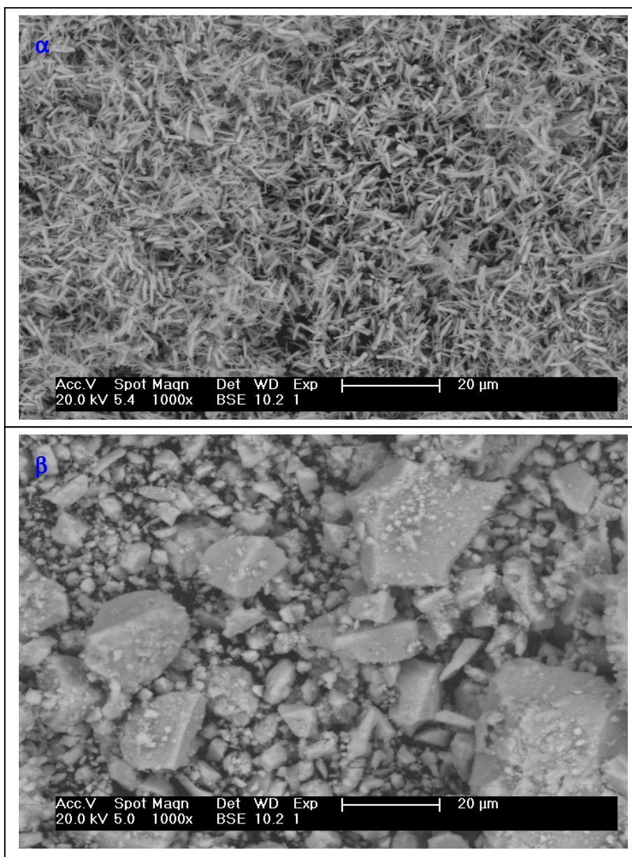
Figure II.17.b : Images MEB de la poudre de dioxyde de cérium ( \text{CeO}_2 ) : \alpha ) synthétisée par la décomposition thermique de \text{Ce}_2\text{O}(\text{CO}_3)_2, \text{H}_2\text{O} à 200^\circ\text{C} , \beta ) élaborée à température ambiante par la voie B.
