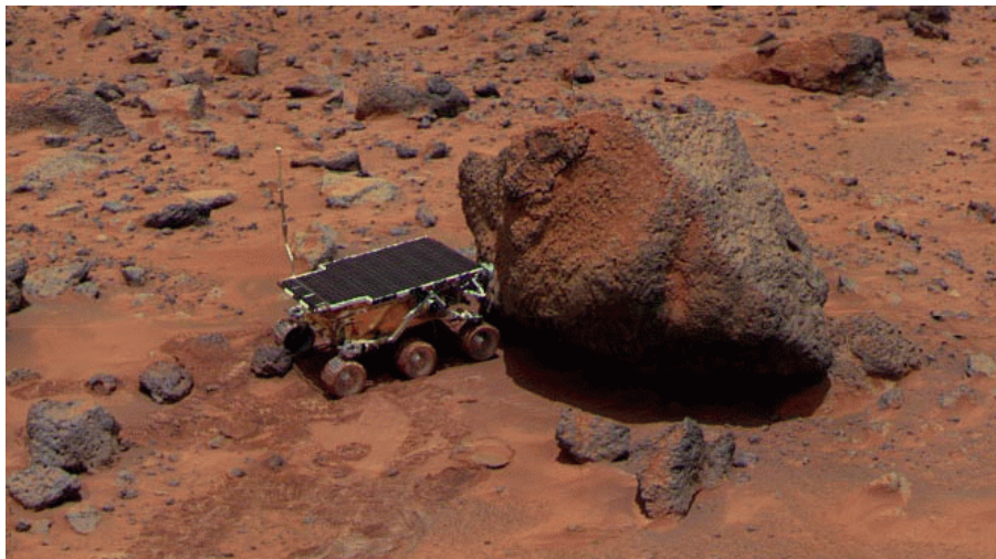
FIG. 3.2 – Sojourner sur la planète Mars. Ce robot est semi-autonome, il dispose d'algorithmes lui permettant d'éviter les obstacles simples alors que les obstacles trop importants requièrent l'intervention d'un opérateur humain, tâche rendue difficile par les délais de communication entre la planète Terre et la planète Mars.
