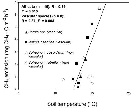
Figure 19. Corrélation entre la température du sol (-10 cm) et les émissions de CH 4 des plots dominés par des sphaignes et des végétaux vasculaires. La droite de régression ( Y = 1.56 X - 19.5, R^2 = 0.35 ) a été dessinée en utilisant toutes les données.
