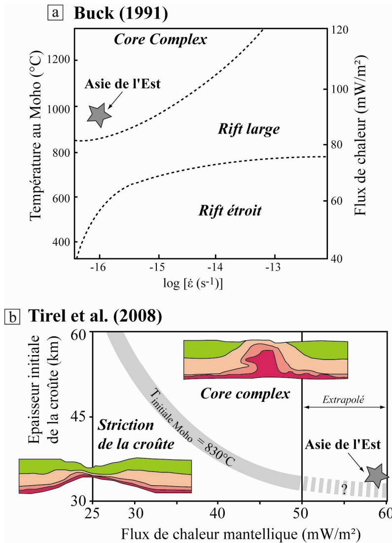
Figure 7.12 : (a) et (b) Conditions exceptionnelles présentes en Asie de l'Est permettant le développement de dômes extensifs sans croûte préalablement épaissie. Les conditions pour le modèle de Buck (1991) sont une croûte d'épaisseur initiale de 40 km et une rhéologie crustale avec du quartz non hydraté.
