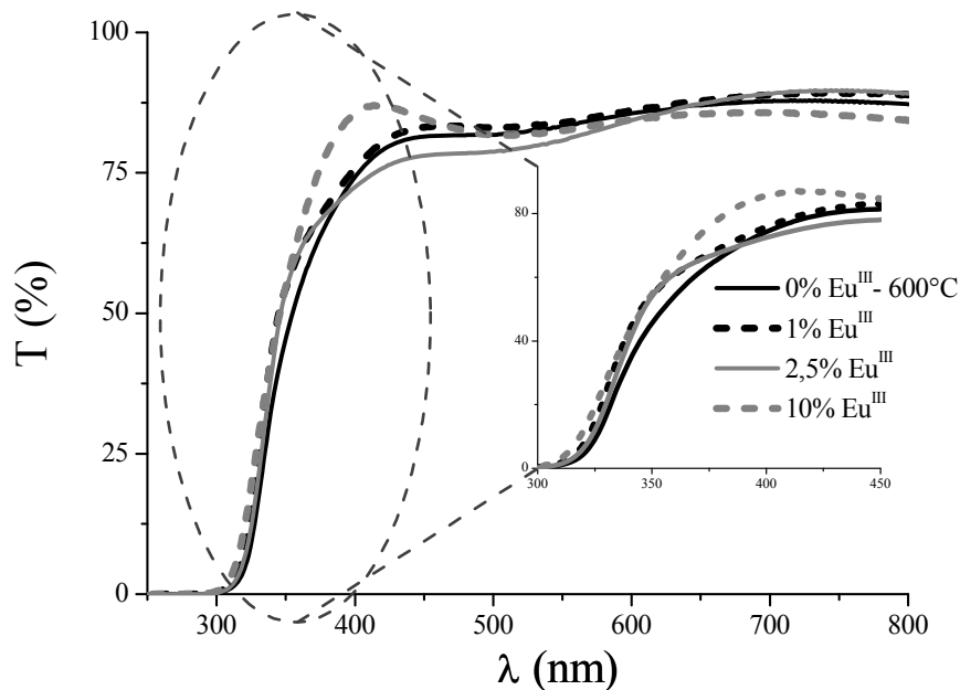
Figure III-8 : Spectres de transmission UV-Visible de films mésoporeux \text{TiO}_2 , dopés et non dopés avec des ions \text{Eu}^{\text{III}} (En encart : zoom du spectre sur la gamme de longueurs d'onde allant de 200 à 260 nm).
