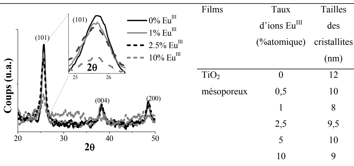
Figure III-7 (à gauche) : Diffractogrammes des films denses \text{TiO}_2:\text{Eu}^{\text{III}} traités à 600^\circ\text{C} contenant 0% (—), 1% (—), 2,5% (- -) et 10% (- -) d'ions \text{Eu}^{\text{III}} – L'encart à droite montre le diffractogramme réalisé avec un temps de comptage accru sur le domaine angulaire correspondant à la réflexion (101) de l'anatase.
