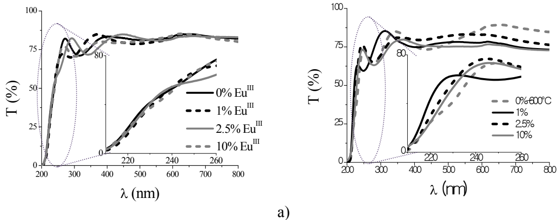
Figure IV-6: Spectres de transmission UV-visible de films mésoporeux ZrO_2:Eu^{III} traités à a) 300°C et b) 600°C, pour différentes concentrations en ions Eu^{III} (En encart : zoom des spectres sur la gamme de longueurs d'onde allant de 200 à 260 nm).
