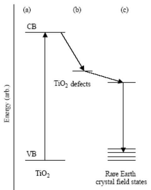
Figure III-15 : Schéma de photosensibilisation de la luminescence d'ions \text{Eu}^{\text{III}} [ Frindell 2003 ]
