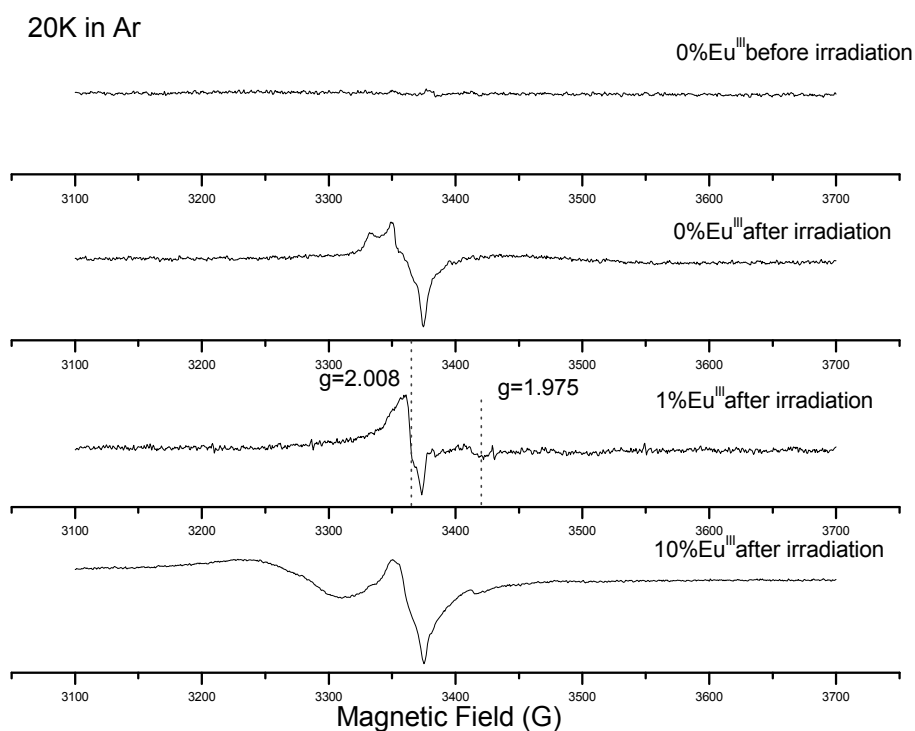
Figure V-13 : Spectres RPE obtenus après irradiation pendant 1 heure à 365nm sous argon, de films TiO 2 contenant 0, 1 ou 10% d'ions Eu III
