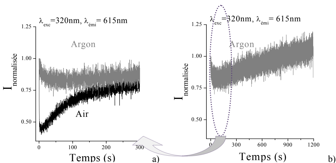
Figure V-8 : Evolution temporelle – aux temps courts (à gauche) et aux temps longs (à droite) – de l'intensité d'émission d'un film mésoporeux \text{TiO}_2:1\%\text{Eu}^{\text{III}} traité à 600^\circ\text{C} soumis à une irradiation continue à 320 nm sous argon. L'évolution temporelle de l'intensité d'émission mesurée sous air a été rajoutée aux temps courts (à gauche) pour mettre en relief la faiblesse de la variation de l'intensité d'émission, observée sous argon.
