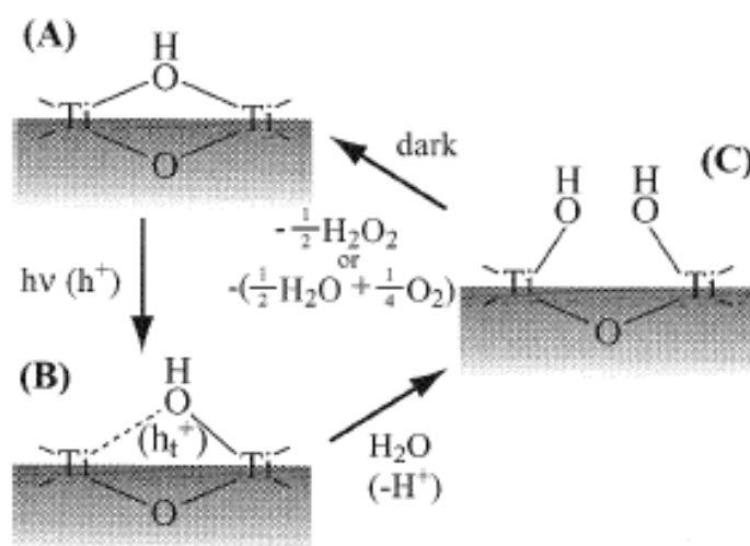
Figure I-18 : Modélisation du processus d’adsorption-désorption d’eau à la surface de \text{TiO}_2 [Sakai 2003]
