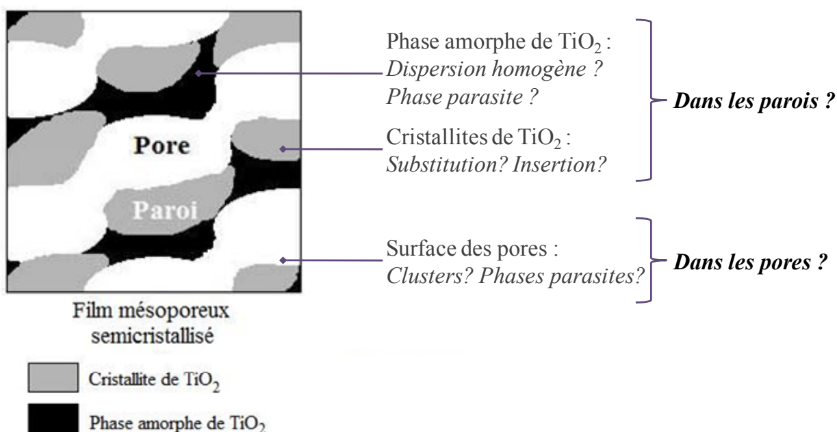
Figure III-1 : Schéma représentant les différentes hypothèses de localisation des ions au sein de films mésoporeux \text{TiO}_2:\text{Eu}^{\text{III}} semicristallisés.
