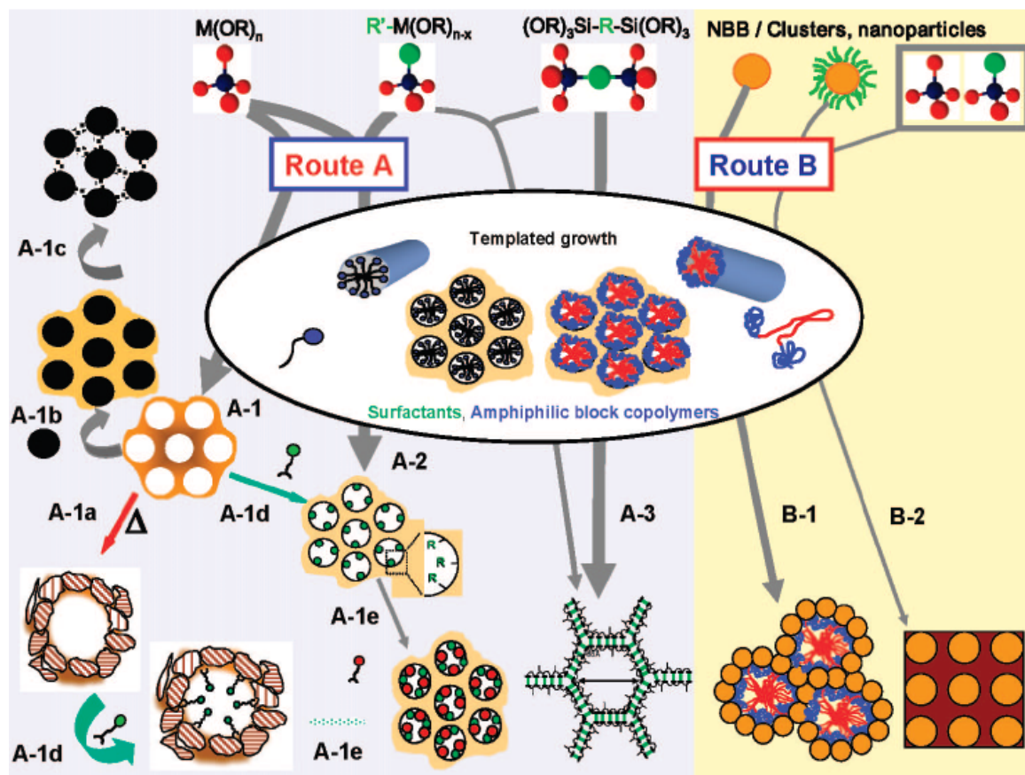
Figure I-3: Les différentes approches pour la réalisation de solides mésoporeux [Sanchez 2008]
