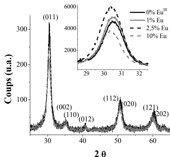
Figure IV-5 (à gauche) : Diffractogrammes des films mésoporeux ZrO_2:Eu^{III} traités à 600^\circ C – L'encart à droite montre le diffractogramme réalisé avec un temps de comptage accru (1000s) sur le domaine angulaire correspondant à la réflexion (011) de la zircone quadratique.
