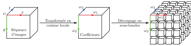
FIG. 5.1 – Découpage des coefficients de la transformée en cosinus locale pour obtenir comme dans une analyse multi-résolutions différentes sous-bandes de détails.
