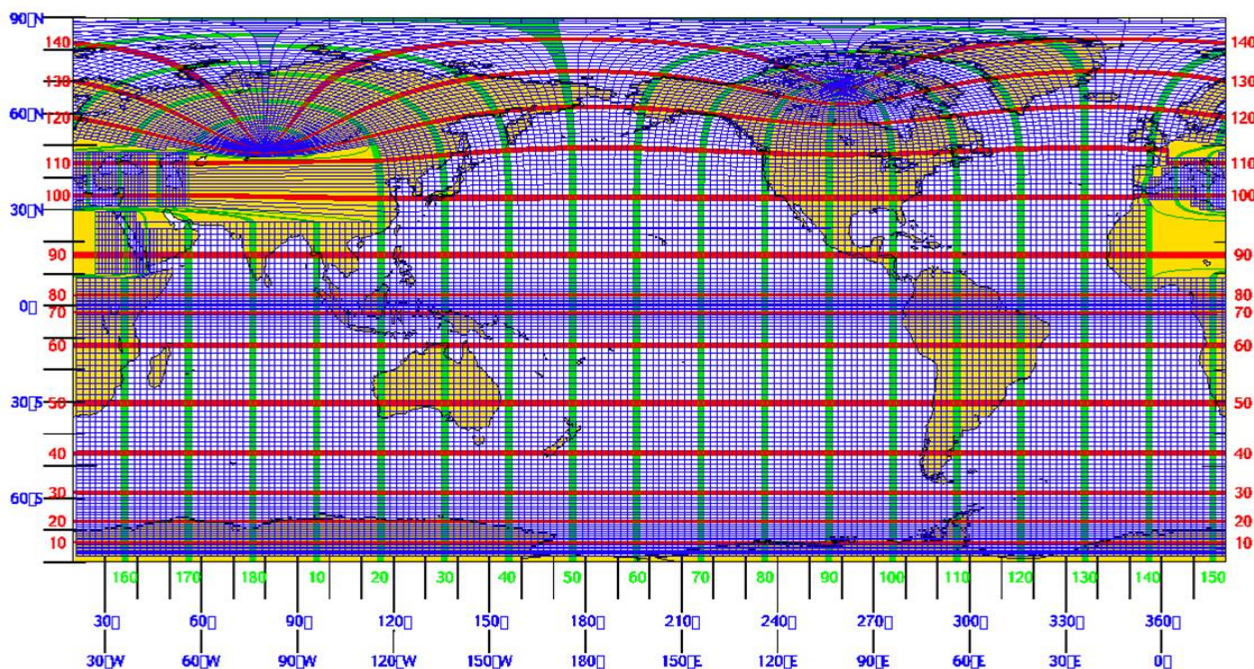
FIGURE 2.1 – Maillage de la grille ORCA2. Les nombres verts et rouges représentent les indices horizontaux et verticaux de la grille.
