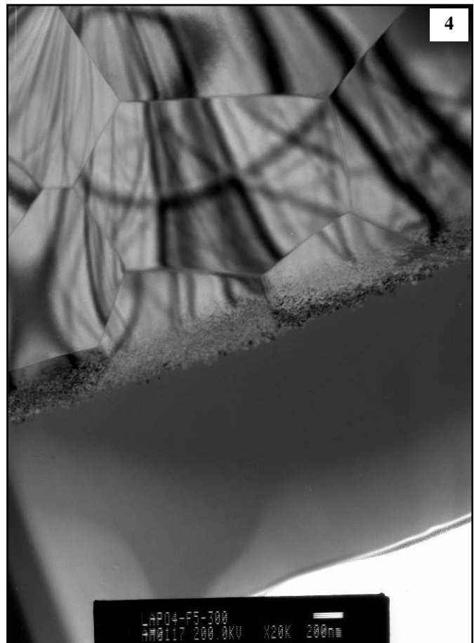
Figure 3: Différents exemples de découpes réalisées avec une sonde ionique focalisée (FIB-Focused Ion Beam). 1 à 3: 3 images de coupes FIB en places dans l'échantillon et 4- image MET en champ clair d'une partie d'une feuille FIB. 1) Coupe effectuée à l'interface entre 2 cristaux de dureté différente (le cristal de droite, plus tendre, apparaît en dessous de la surface); notez la présence de porosité dans le cristal de gauche et le joint de grain (clair) de plusieurs centaines de nm d'épaisseur d'inclinaison "NW-SE". 2) Coupe FIB réalisée à travers une petite inclusion (~2μm de large en surface). 3) Coupe FIB effectuée transversalement à une surface d'altération dans un cristal de feldspath. 4) Image en MET champ clair d'une partie de feuille FIB réalisée perpendiculairement à une surface d'irradiation (bombardement externe par un faisceau d'ions Au qui induit l'amorphisation d'une zone sous la surface d'environ 1.5 μm). Voir aussi Wirth (2004 et 2009).
