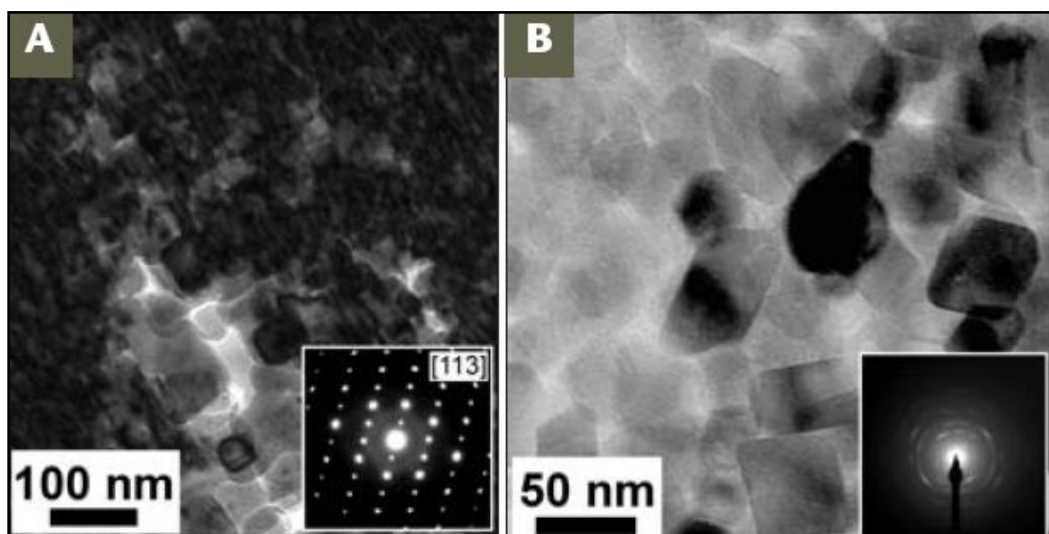
Figure 25: Photos MET (BF) de zircons amorphes (A- Geisler et al., 2004 ; B- Schmidt et al., 2006) altérés expérimentalement. Notez la présence de nano-cristallites orientés (A) ou sans orientation préférentielle (B), séparés par une nano-porosité ainsi que la présence de matière amorphe (cercles diffus en diffraction dans A). D'après Geisler et al. (2007).
