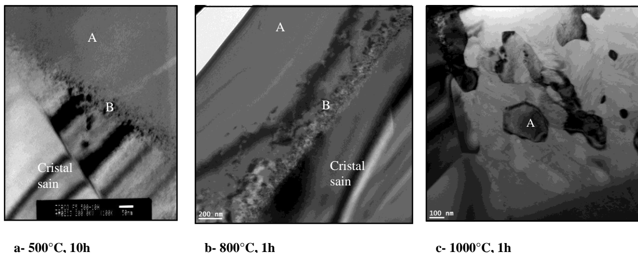
Figure 17. Images MET en champs clairs de frittés de zirconolites irradiées à la fluence F5 (cf tableau 1) puis recuits à 500°C, 10h (a), 800°C, 1h (b) et 1000°C, 1h (c). Notez la cristallisation de la zirconolite amorphe dès 800°C (contrastes de Bragg visibles) et se terminant à 1000°C; les défauts "intermédiaires" restent stables jusqu'à 800°C inclus. Rq: la zirconolite ne recristallise pas sous le faisceau électronique.
