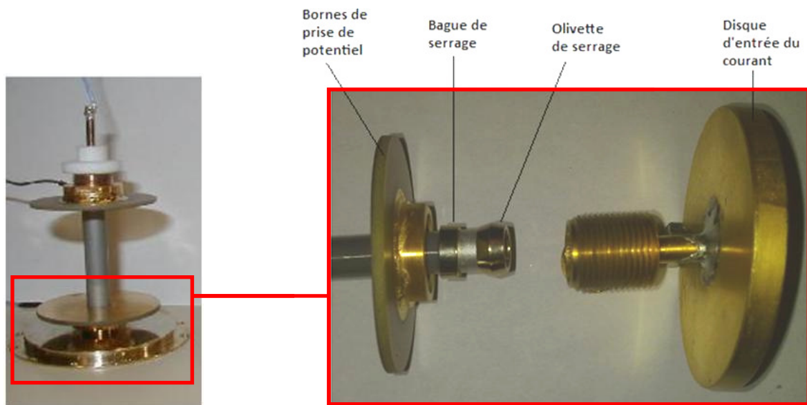
Fig.45 : Premier dispositif coaxial pour la mesure des résistances
