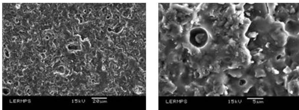
Fig.56 : Micrographies MEB de la surface d'une résistance de 1914 \Omega à différents grossissements
