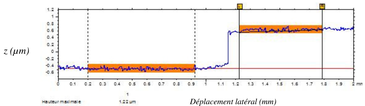
Fig.69 : Profil d'épaisseur obtenu par profilométrie sur un substrat plan en alumine (extrémité gauche du barreau en acier)
