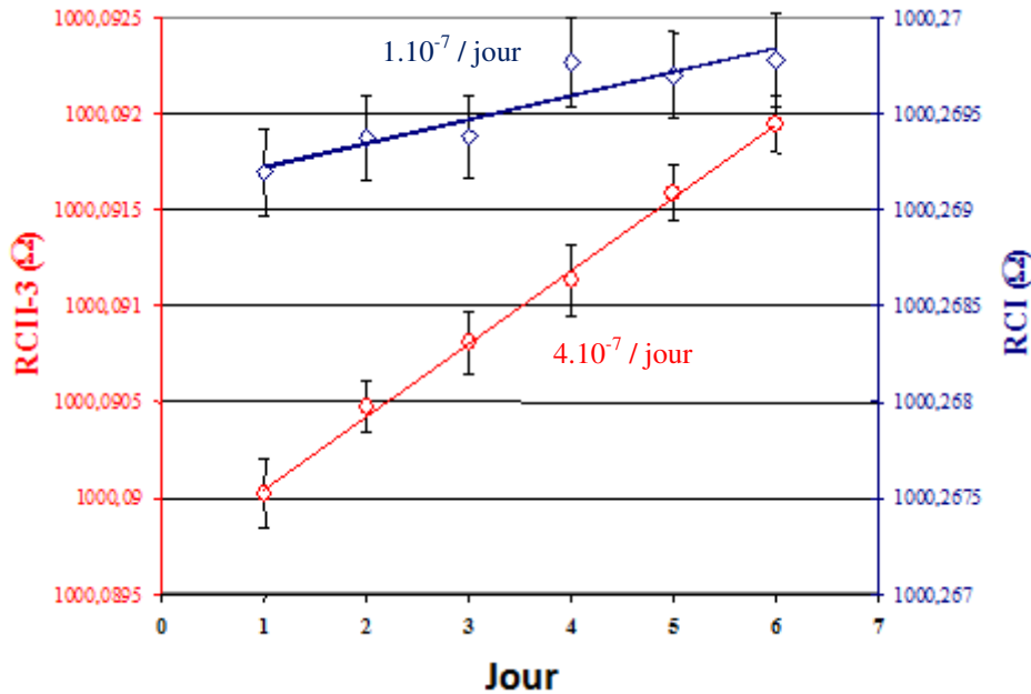
Fig.24 : Evolution de la résistance RCII-3 et RCI-1 à 27 °C en fonction du temps
