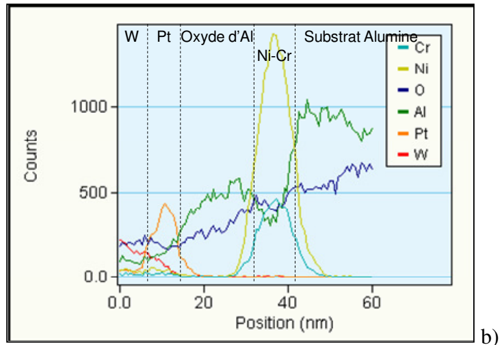
Fig.83 : Profil EDS (a) et spectres associés (b) des éléments chimiques en présence
