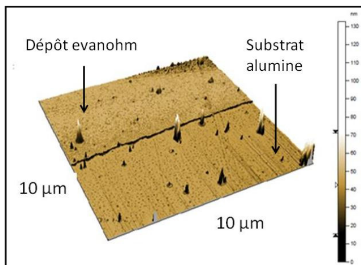
Fig.77 : Cartographie AFM de l'état de surface d'un revêtement d'evanohm ultra-mince de 9 nm d'épaisseur au niveau de la marche sur un substrat plan en alumine
