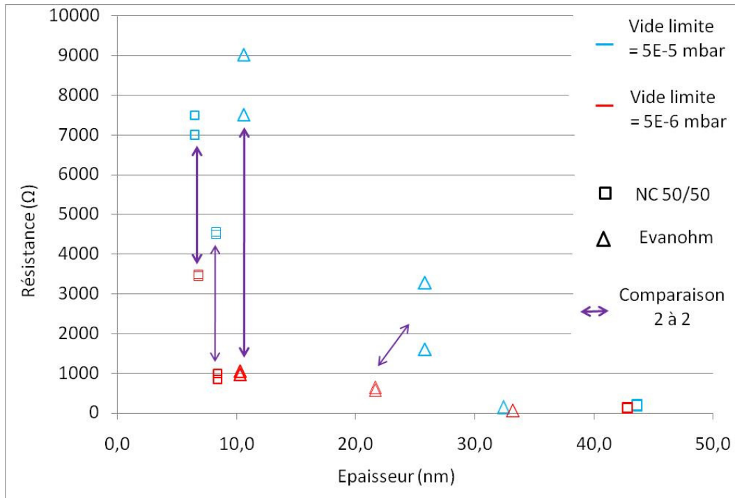
Fig.91 : Evolution de la valeur des résistances en fonction de l'épaisseur réelle des couches pour des vides limites différents
