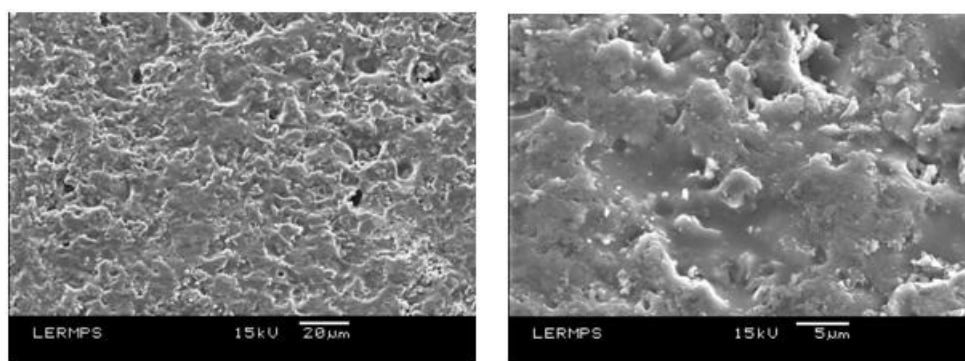
Fig.54 : Micrographies MEB de la surface d'une résistance de 290 \Omega à différents grossissements
