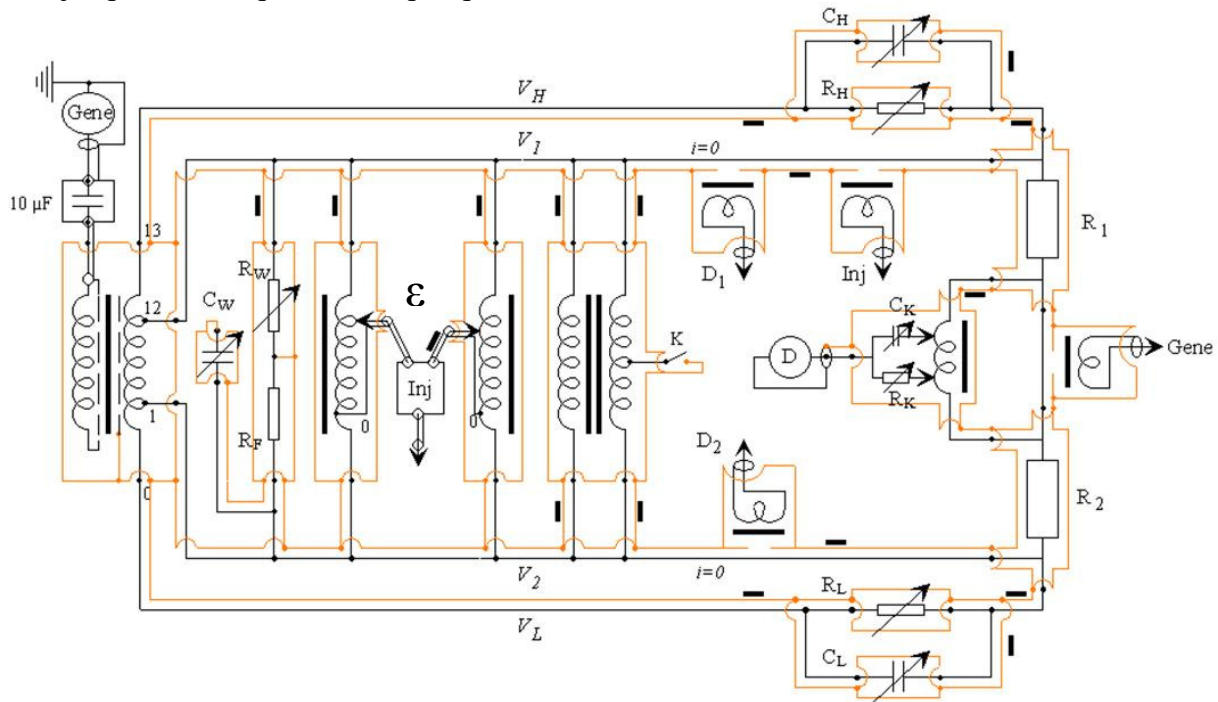
Fig.25 : Schéma électrique du pont de comparaison coaxial à quatre paires de bornes
