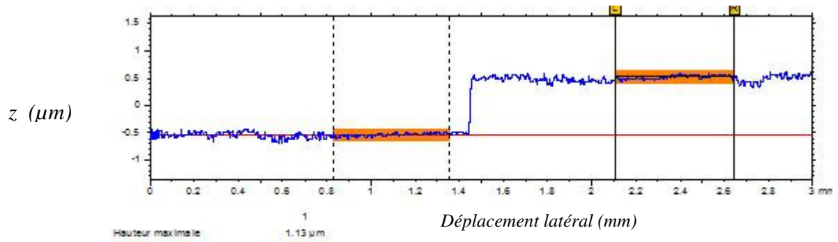
Fig.68 : Profil d'épaisseur obtenu par profilométrie sur un substrat plan en alumine (extrémité droite du barreau en acier)
