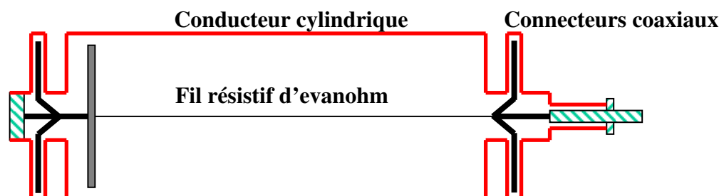
Fig.8 : Schéma simplifié d'une résistance à fil de type Haddad
