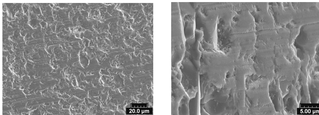
Fig.74 : Micrographies MEB à différent grossissement de la surface d'un bâtonnet couvert d'un film d'evanohm d'environ 70 nm d'épaisseur
