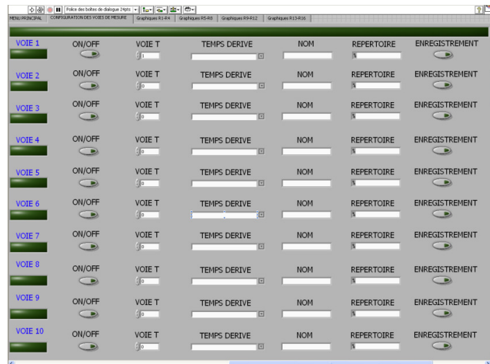
Fig.51 : Face avant du programme Labview pour le pilotage des voies de mesure
