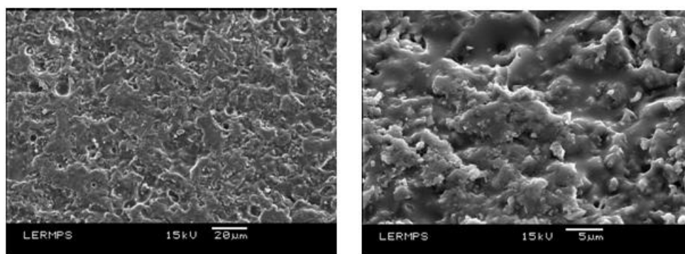
Fig.55 : Micrographies MEB de la surface d'une résistance de 1090 \Omega à différents grossissements
