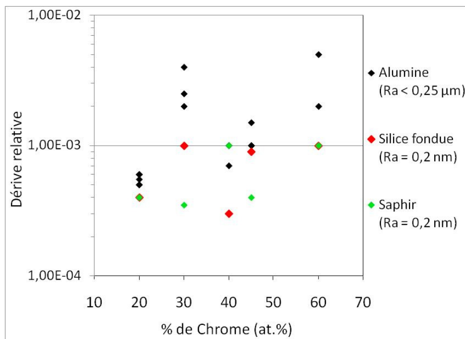
Fig.101 : Evolution de la dérive relative de résistances en nichrome de même épaisseur mais de différentes compositions chimiques et pour différents substrats
