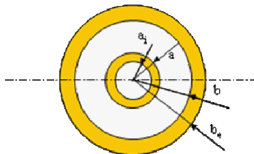
Fig.16 : Coupe schématique transversale d'une résistance calculable coaxiale
