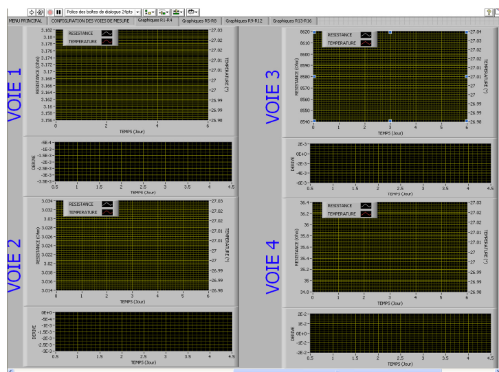
Fig.52 : Face avant du programme Labview pour la visualisation graphique des données acquises
