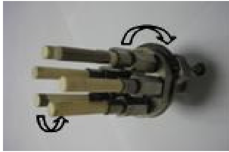
Fig.32 : Porte-échantillon rotatif multiple
