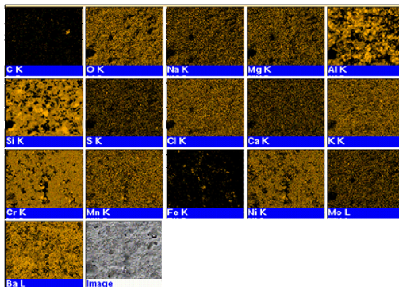
Fig.61 : Cartographie des éléments présents (en jaune) dans la zone étudiée (cf. image MEB associée) de la surface d'un revêtement
