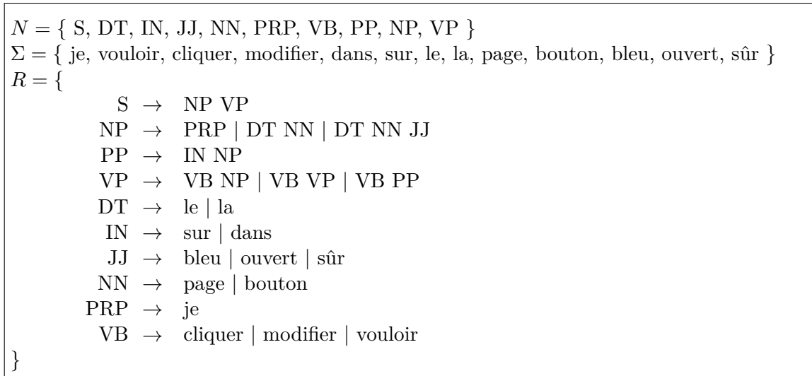
Figure 1.7 Exemple de grammaire \mathcal{G}_{ex}
