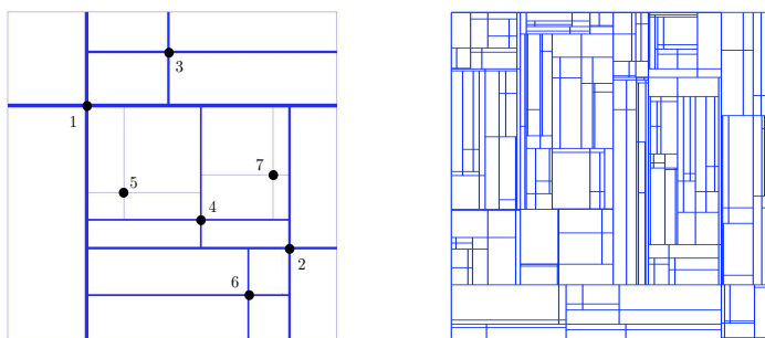
FIGURE 2.4 – Deux quadtrees. L'un avec 7 points l'autre avec 100.
