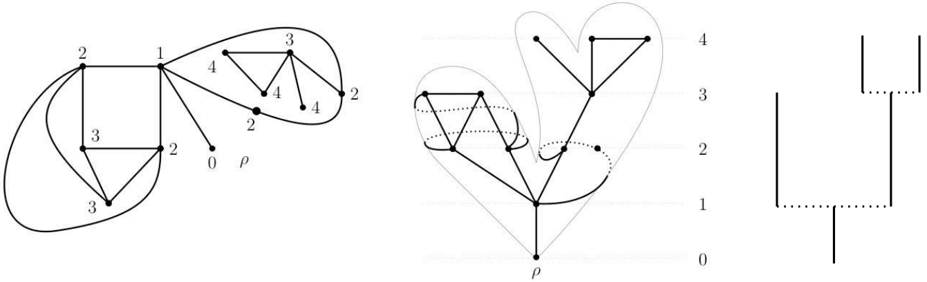
FIGURE 1.4 – Une carte planaire pointée en \rho et sa représentation en « cactus »
