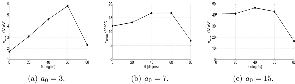
FIGURE 6.8 – Énergie maximale des protons en face arrière pour a_0 = 3, 7 et 15.
