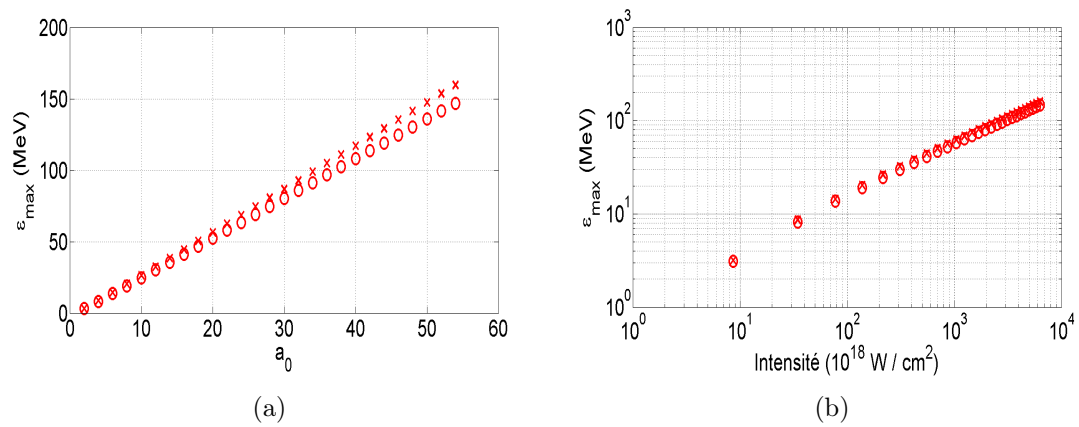
FIGURE 6.11 – Energie maximale des protons calculée pour l'angle limite, en utilisant p'_{xf}/m_e c = 3a_0 avec les paramètres du laser LUIRE a) en fonction de a_0 et b) en fonction de l'intensité pour T_h^W (ronds) et T_h^{Ha} (croix).
